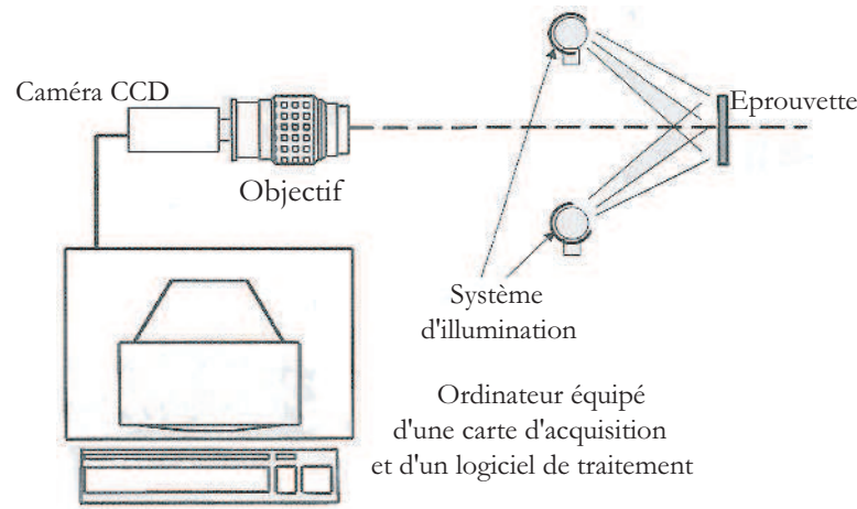
FIG. 2.7 – Schéma d'un système d'acquisition de données pour un montage de corrélation d'image numérique bi-dimensionnel (Extrait de [144]).
