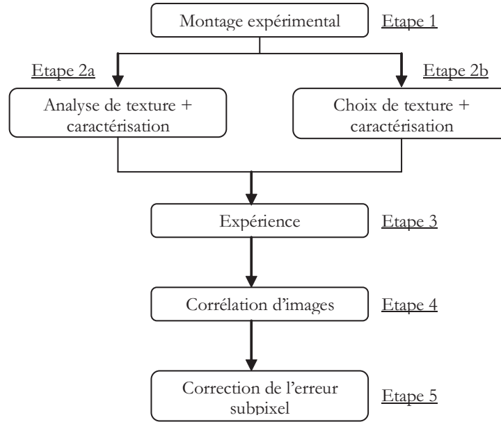
FIG. 3.28 – Procédure à appliquer pour l'aboutissement d'une expérience de corrélation d'images numériques fiable et répétitive.
