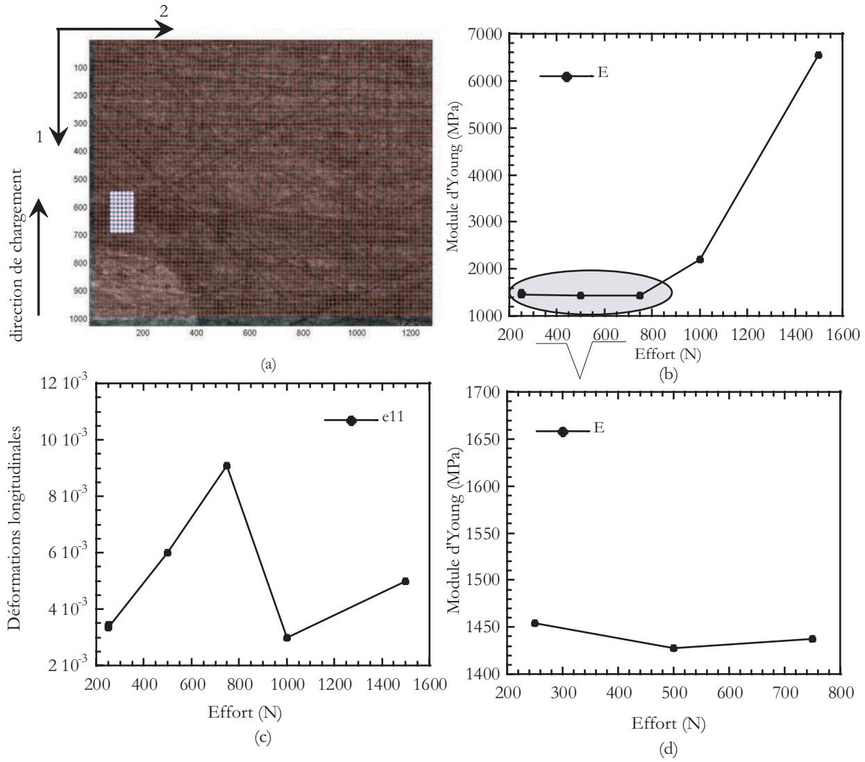
FIG. 4.11 – Evolution longitudinales (c) et du module d'Young (b) de la zone 1 (a). L'illustration (d) montre la zone de comportement élastique du tracé (b).
