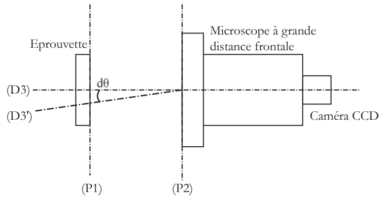
FIG. 3.4 – Parallélisme des plans (P1) , correspondant à la surface de l'objet, et (P2) de la lentille du système d'observation. (D3) représente l'axe idéal de positionnement et (D3') un axe avec un défaut d'angle d\theta par rapport à (D3) .
