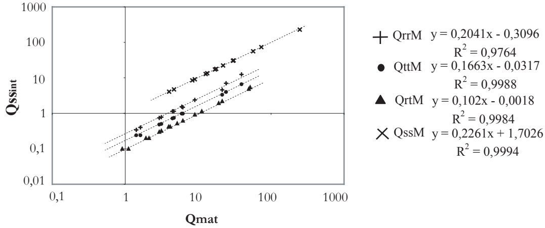
FIG. 6.5 – Influence des variations de rigidité de la matrice ( Log(\%) ) sur la rigidité Q_{ssint} de l'interphase ( Log(\%) ). A droite du graphique sont indiquées les équations des droites approximant les points avec leurs coefficients de corrélation.
