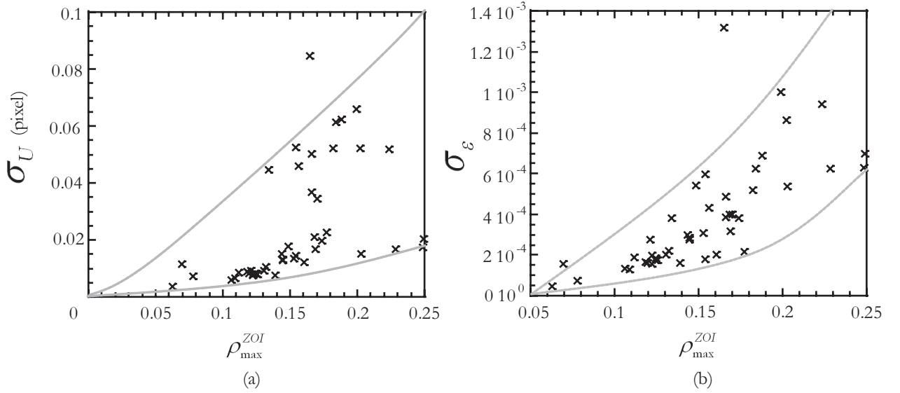
FIG. 3.13 – Influence du critère de rayon de corrélation sur les performances d'incertitude en déplacement (a) et en déformation (b).
