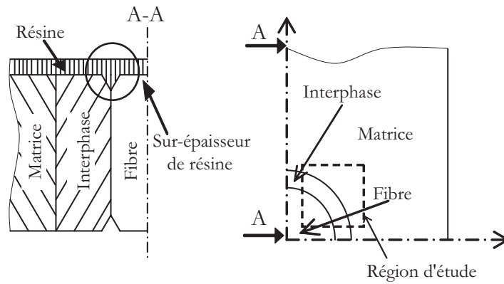
FIG. 5.12 – Illustration du positionnement de la sur-épaisseur de résine au niveau de l'interface fibre - interphase.
