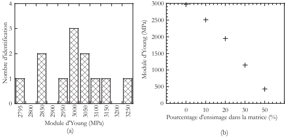
FIG. 6.10 – Module d'Young de la résine utilisée pour la matrice lors de plusieurs essais (a) et évolution du module d'Young pour une éprouvette avec différents pourcentages d'ensimage (b).
