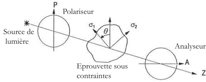
FIG. 2.3 – Montage technique d'un polariscope linéaire (Extrait de [34]).
