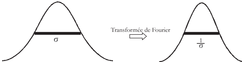
FIG. 2.2 – Transformée de Fourier d'une fonction Gaussienne.
