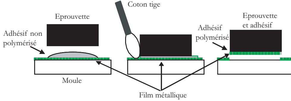
FIG. 5.1 – Dépôt de réseau de diffraction sur l'éprouvette par réplique.
