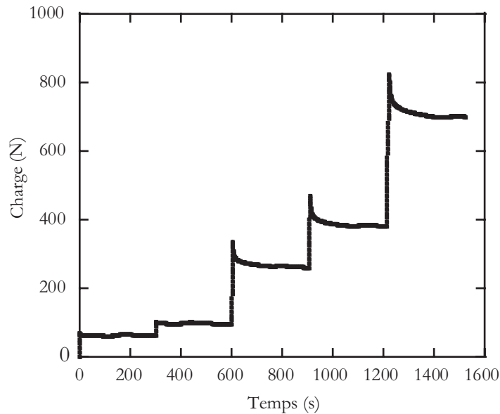
FIG. 4.5 – Mesure du capteur de charge (max. 5 kN) de la traverse au cours de l'expérience.
