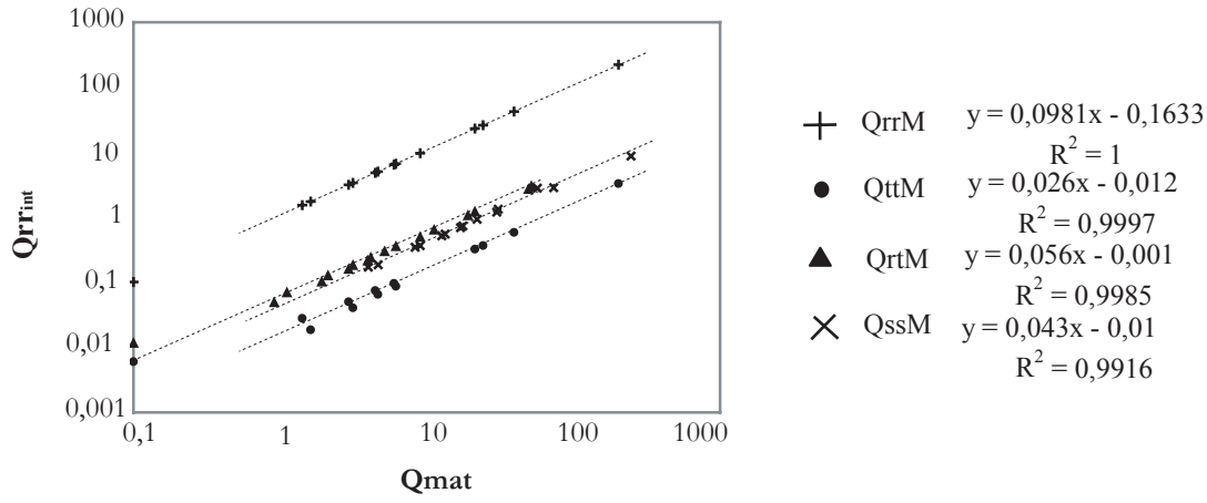
FIG. 6.4 – Influence des variations de rigidité de la matrice ( Log(\%) ) sur la rigidité Q_{rrint} de l'interphase ( Log(\%) ). A droite du graphique sont indiquées les équations des droites approximant les points avec leurs coefficients de corrélation.
