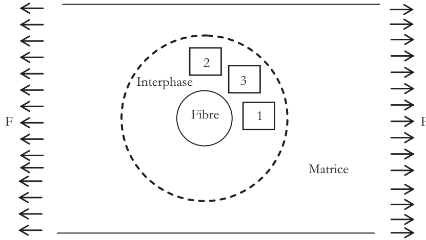
FIG. 4.10 – Zones permettant l’identification directement des propriétés mécaniques de l’interphase : zone 1 - le module d’Young, zone 2 - le coefficient de Poisson et zone 3 - cisaillement maximum.
