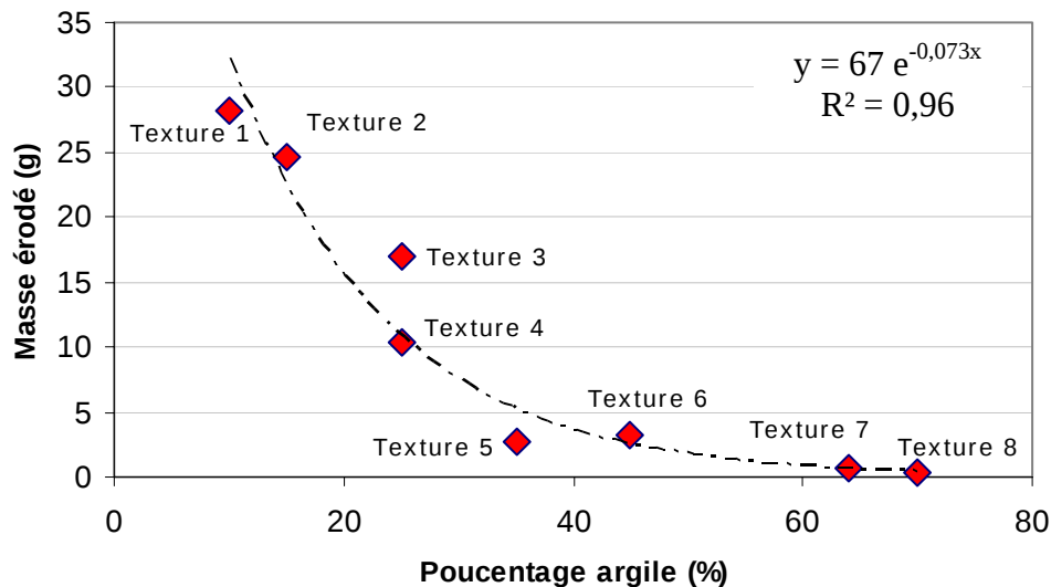
Figure 5-1 : Masse érodée en fonction du pourcentage d'argile
