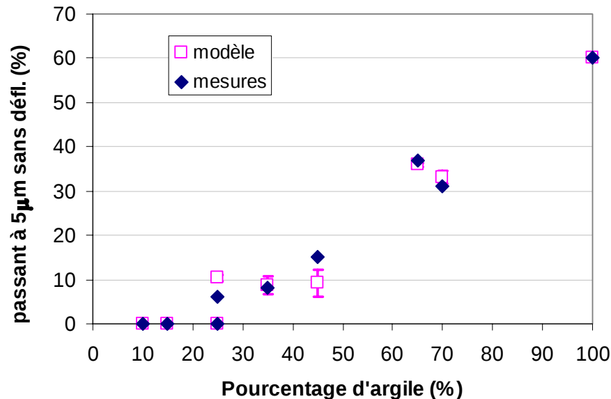
Figure 5-5 : Passant à 5\mu\text{m} sans défloculant: comparaison du modèle et des valeurs mesurées. Les points et les barres d'erreur correspondant au modèle sont obtenus avec \varphi = 0,6 \pm 0,1 .
