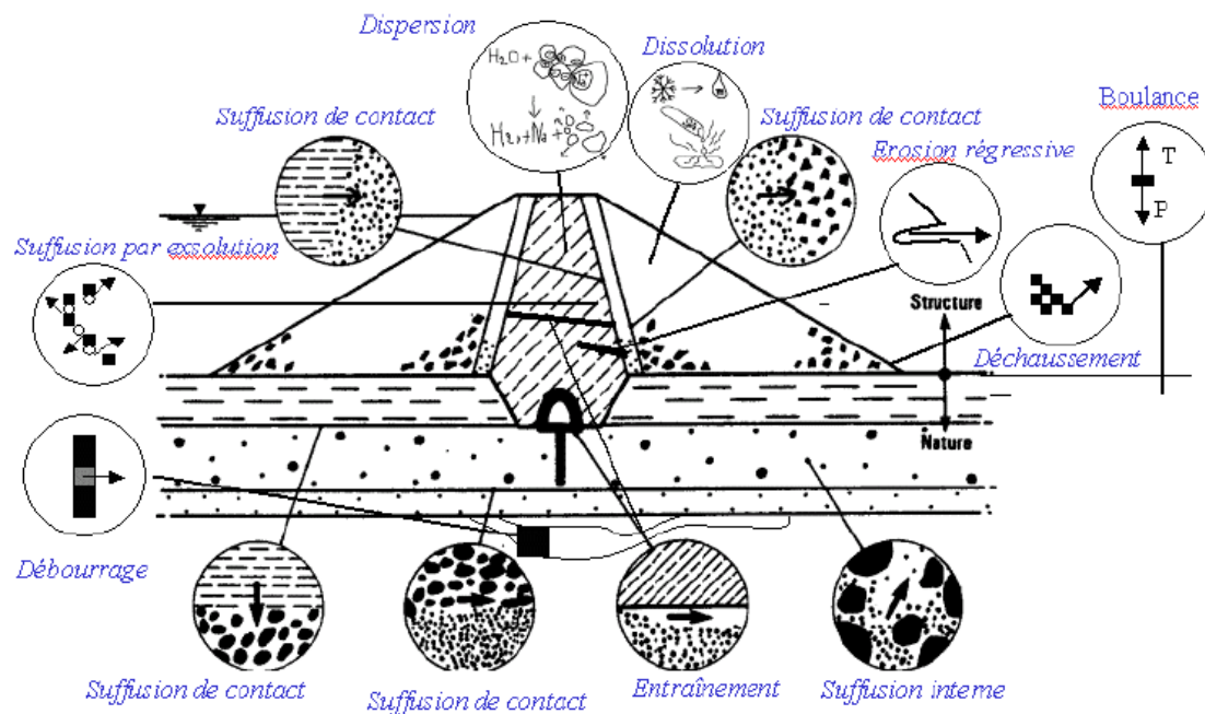
Figure 1.15 : Schéma représentatif des divers phénomènes initiateurs de l'érosion dans un barrage (adapté de Schuler et Brauns 1996, cité par Blais, 2004)
