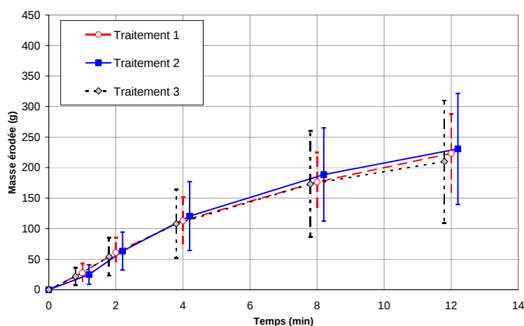
Figure 3.25 : Résultat des essais d'érodimétrie selon notre nouveau protocole pour le site 2
