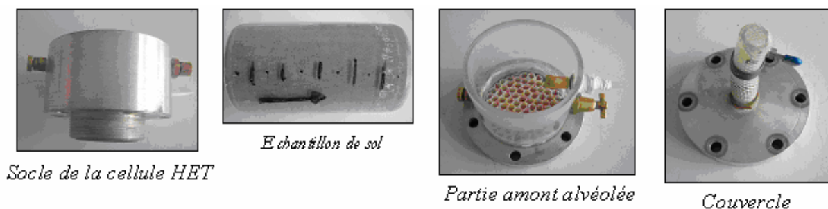
Figure C.2 Schéma détaillé de la cellule d'essai, HET, 1 LCPC
