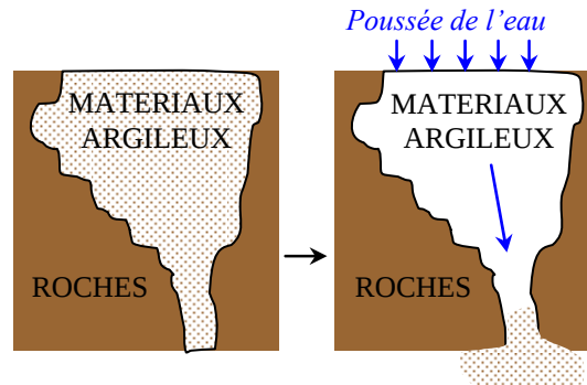
Figure 1.13 : Phénomène de débouillage
