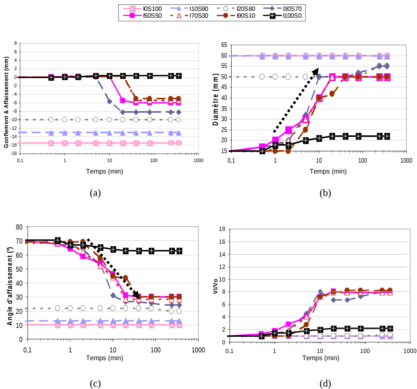
Figure 5-12. Mélange illite (I)/sable (S) (a) Courbe de gonflement/affaissement (b) Courbe d'élargissement, (c) Angle d'affaissement (d) Rapport du volume à l'instant t et volume initial
