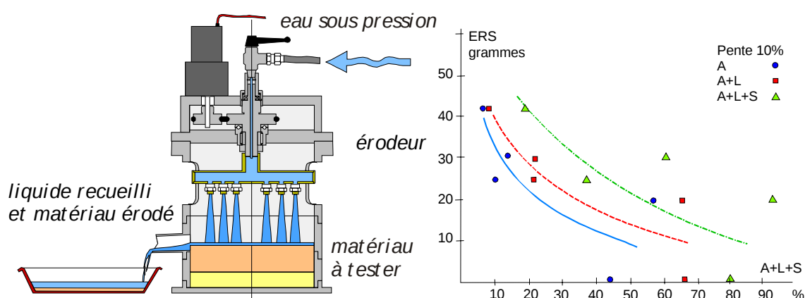
Figure 1.29 : Schéma de l'essai d'érosion par érodimètre LCPC (Hénensal et al., 1987) et variation de l'érodabilité en fonction de la texture (Hénensal et Rampon, 1994)
