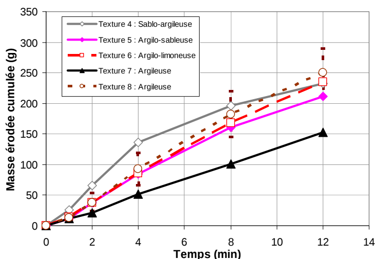
Figure 3.7 : Masse érodée des différentes textures de sol avec l'érodimètre à jets mobiles
