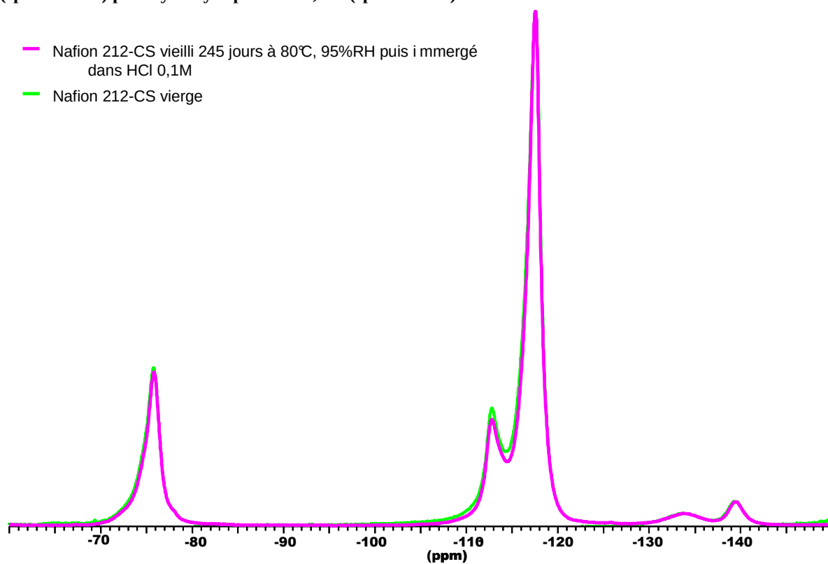
Figure VI- 6 Superposition du spectre RMN ^{19}\text{F} du Nafion ® 212-CS vierge et d'un échantillon de Nafion ® 212-CS vieilli 245 jours à 80°C, 95%RH puis hydrolysé par HCl 0,1M
