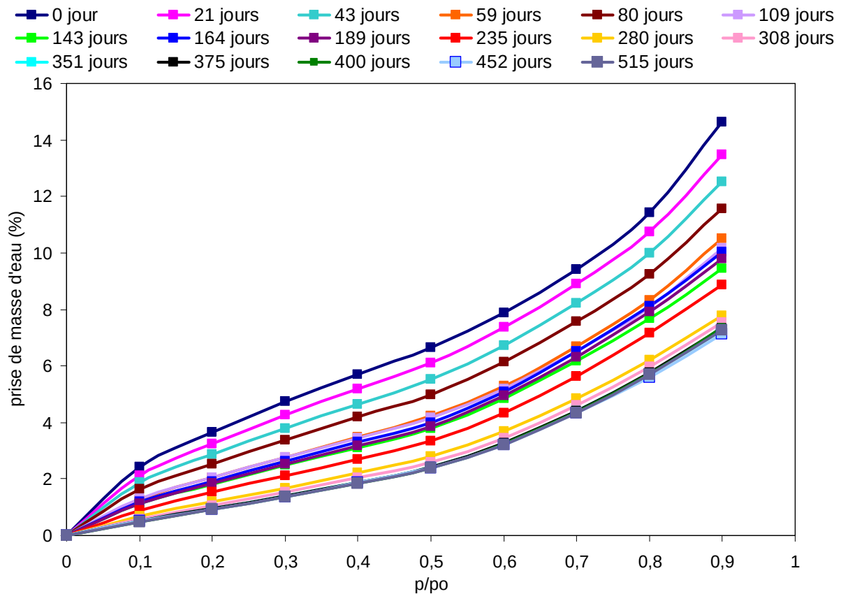
Figure IV- 5 Evolution des isothermes de sorptions d'échantillons de Nafion® 212-CS vieillies à 80°C, 80%RH
