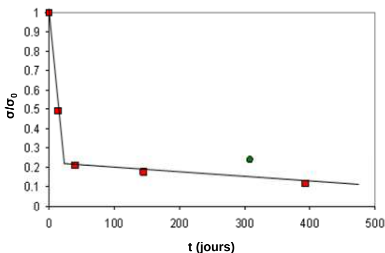
Figure IV- 8 Conductivité ionique du Nafion® 112 (points rouges) et 212-CS (point vert) en fonction du temps de vieillissement en enceinte climatique (80°C, 80%RH)
