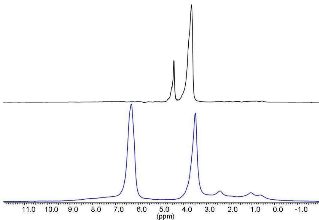
Spectres RMN ^1\text{H} d'échantillon de Nafion® 112 vieilli 203 jours à 80°C, 80%RH (spectre bleu) puis hydrolysé par NaOH (spectre noir)
