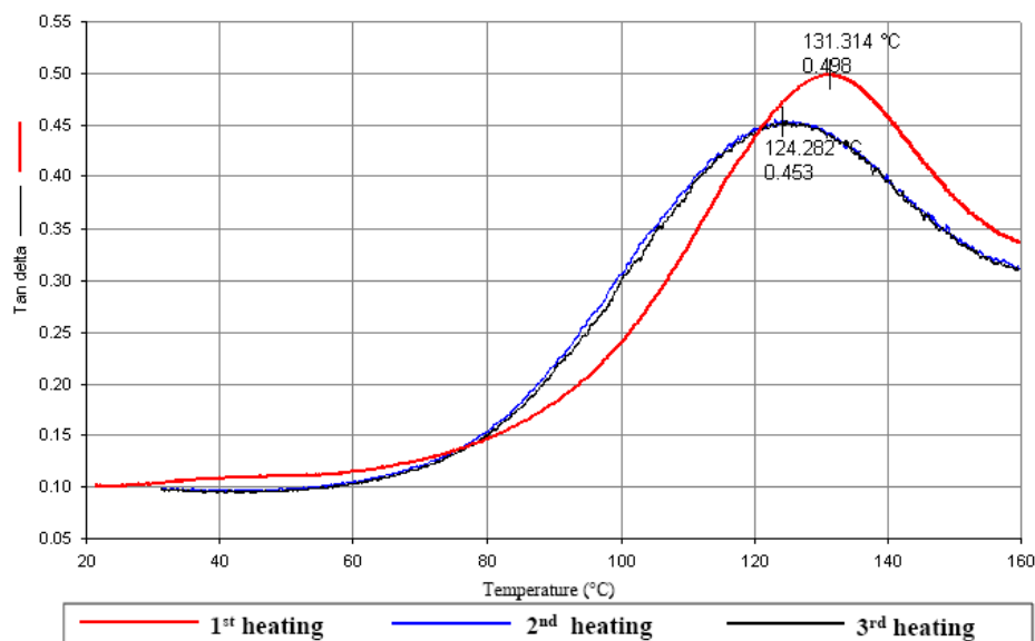
Figure I- 23 Evolution de tangente \delta pour des échantillons vieillis à 90°C pendant 80 jours dans de l'eau déionisée 22
