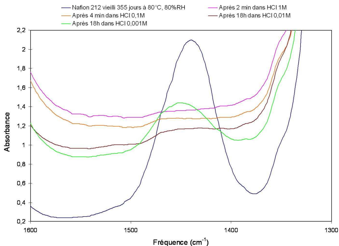
Figure VI- 4 Superposition du spectre d'un échantillon de Nafion ® 212-CS vieilli 355 jours à 80°C, 80%RH puis hydrolysé par différentes solution d'acide chlorhydrique
