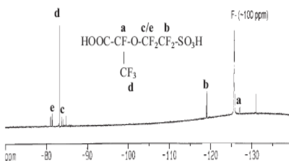
Figure I- 20 Spectre RMN 19 F d'un des produits de dégradation du Nafion® (Figure tirée de la référence 74)
