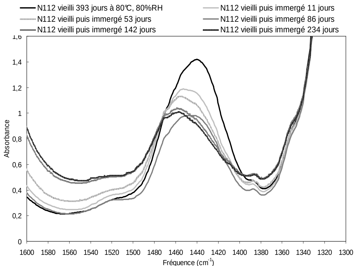
Figure VI- 1 Observation de la bande de l'anhydride sulfonique ( 1440\text{ cm}^{-1} ) d'un échantillon de Nafion ® 112 vieilli 393 jours en enceinte climatique ( 80^{\circ}\text{C} , 80\%\text{RH} ) puis immergé dans l'eau à 80^{\circ}\text{C} au cours du temps
