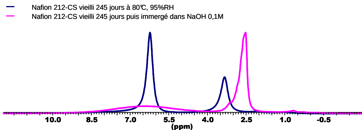
Figure VI- 11 Spectres RMN ^1\text{H} d'échantillon de Nafion ® 212-CS vieilli 245 jours à 80°C, 95%RH (spectre bleu) puis hydrolysé par NaOH 0,1M (spectre rose)
