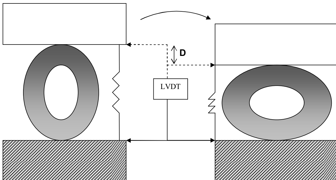
Figure IV.5 : Principe de fonctionnement du capteur LVDT D = Déplacement enregistré par le LVDT correspondant à la déformation de l'échantillon
