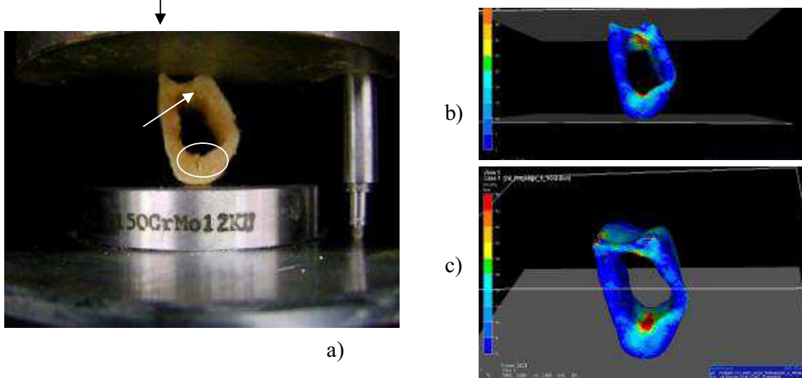
Figure IV.12 : Fin de compression, apparition simultanée de l'endommagement expérimental (a) et des champs de contraintes maximum (b, c) avec \sigma_{max} = 60 MPa
