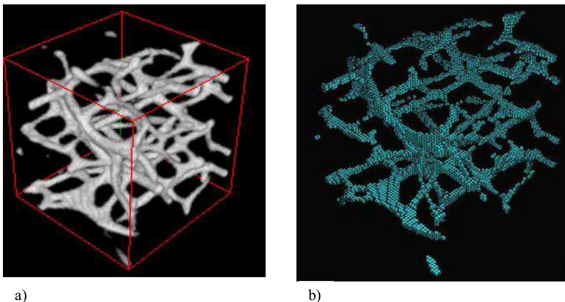
Figure V.2 : a) Modélisation des trabécules de l'os spongieux par microtomographie ( \mu CT) b) Maillage volumique en éléments finis d'après Follet [FOL 07]
