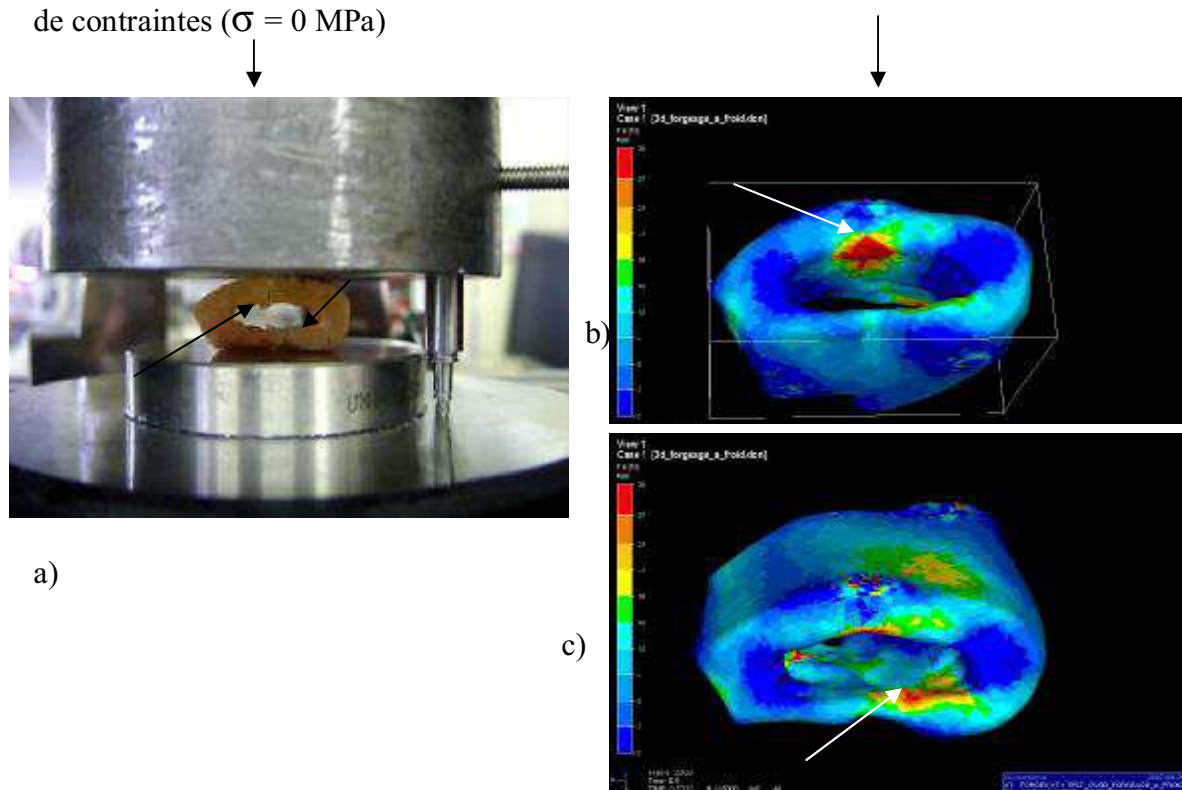
Figure IV.9 : Compression et corrélation entre les zones d'endommagement expérimental de S11P2 (a) et des zones d'apparition des champs de contraintes maximales (b, c) avec \sigma_{\max} = 30 MPa.
