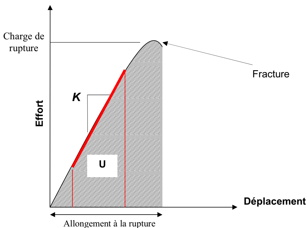
Figure II.10: Courbe d'effort/déplacement
