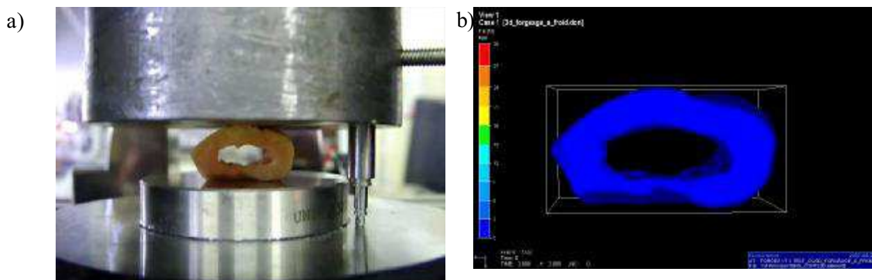
Figure IV.8 : Position initiale de S11P2 expérimental (a) et numérique (b), absence de contraintes ( \sigma = 0 MPa)
