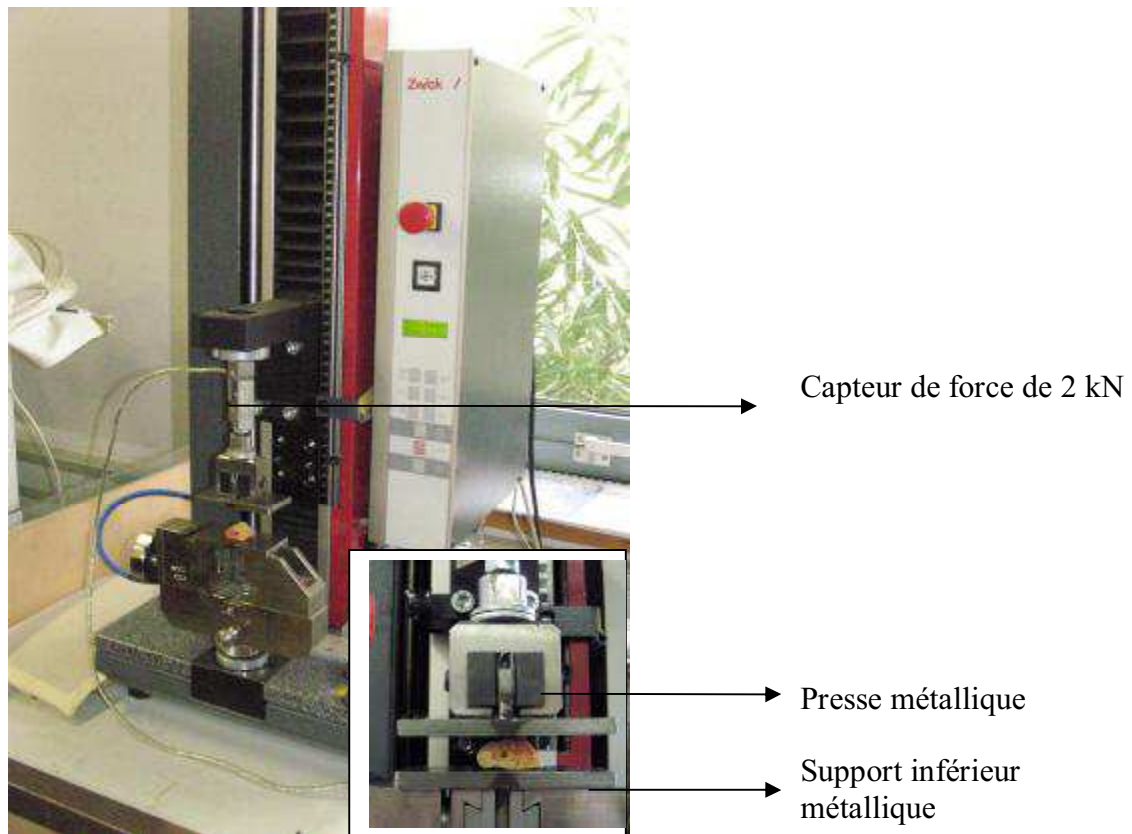
Figure IV.2 : Machine d'essai Zwick®
