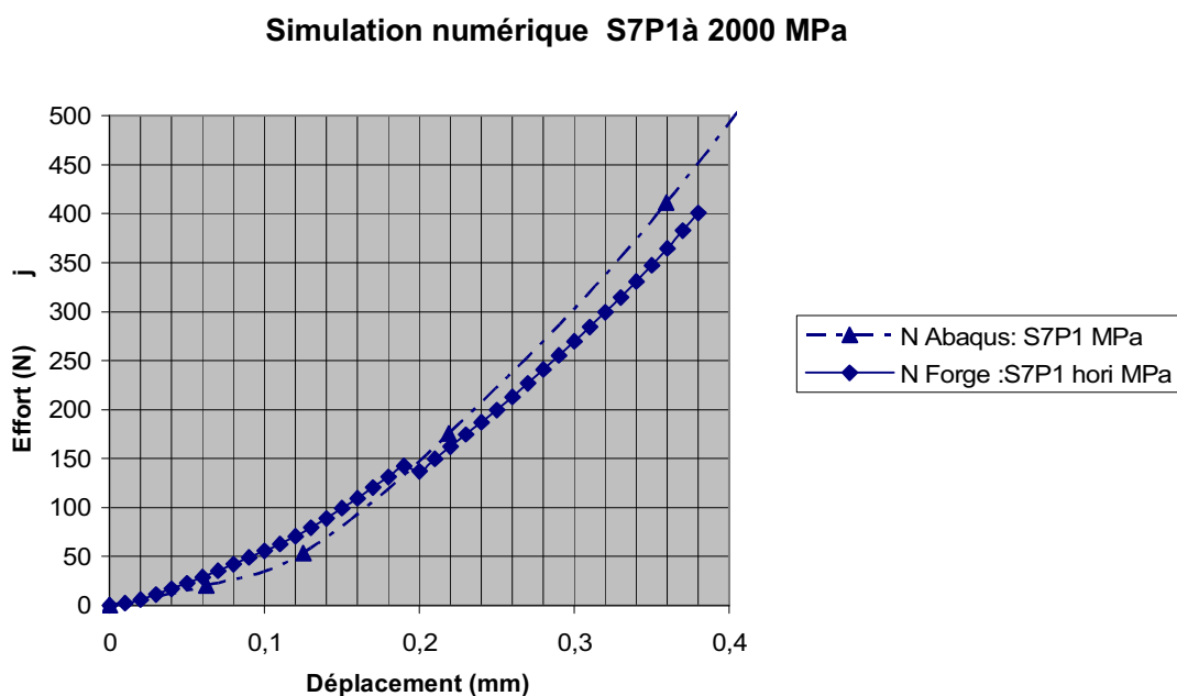
Figure IV.7 : Comparaison des courbes numériques de S7P1 (module d'Young égal à 2000 MPa) issues des simulations par les logiciels ABAQUS® et FORGE®.
