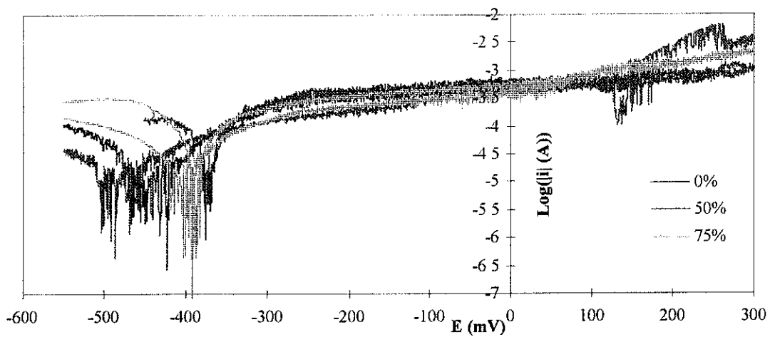
Figure 3 7: Influence de la surface exposée sur le courant total sous frottement (A3, 60 N)
