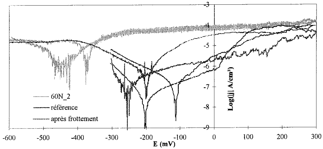
Figure 3 6: Courbe intensité-potentiel après frottement en solution A3
