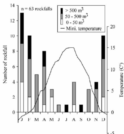
Figure 8. Distribution annuelle des chutes de pierres et de blocs entre 1948 et 2004 et de la température moyenne minimale entre 1971 et 2000 aux environs de Grenoble (Frayssines et al, 2006).
