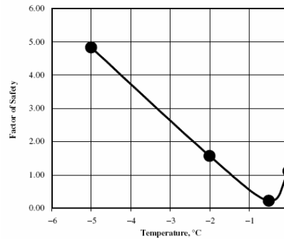
Figure 13. Exemple de diminution du coefficient de sécurité d'une pente avec l'augmentation de la température de la glace dans le joint (Davies et al, 2001).
