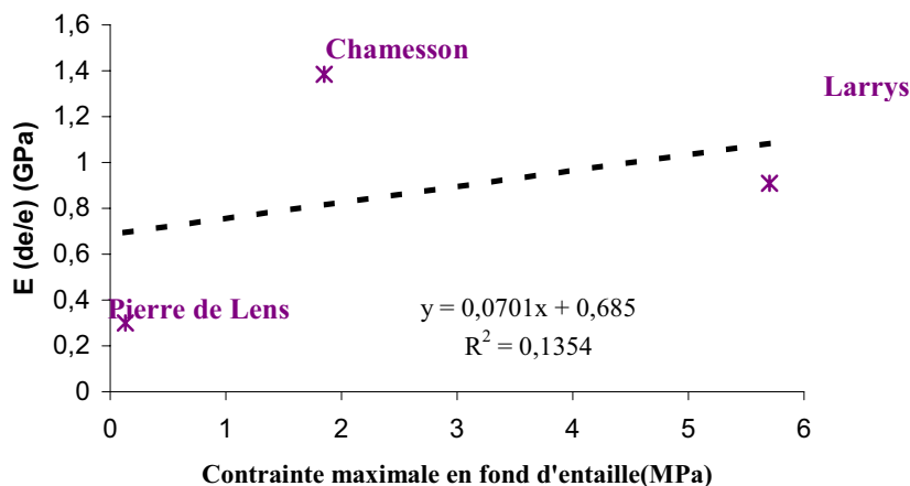
Figure 108. Allure de la contrainte en fond d'entaille en fonction du produit du module par la d eformation de l'ouverture.
