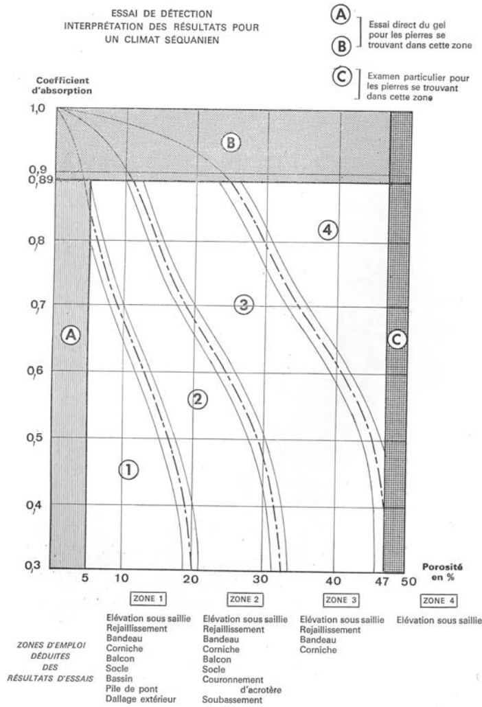
Figure 24. Exemple de classification vis-à-vis du gel, selon Mamillan (1975), pour un climat séquanien.
