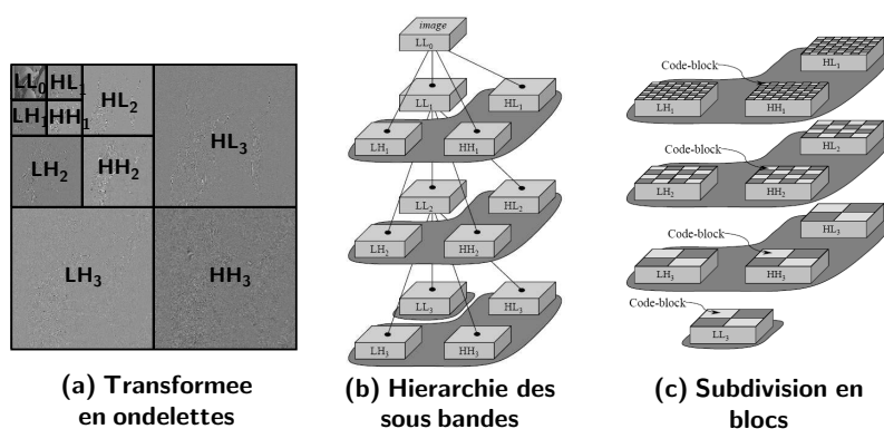
Fig. 3.2 Subdivision en blocs 64 \times 64 des coefficients d'une transformée en ondelettes.
