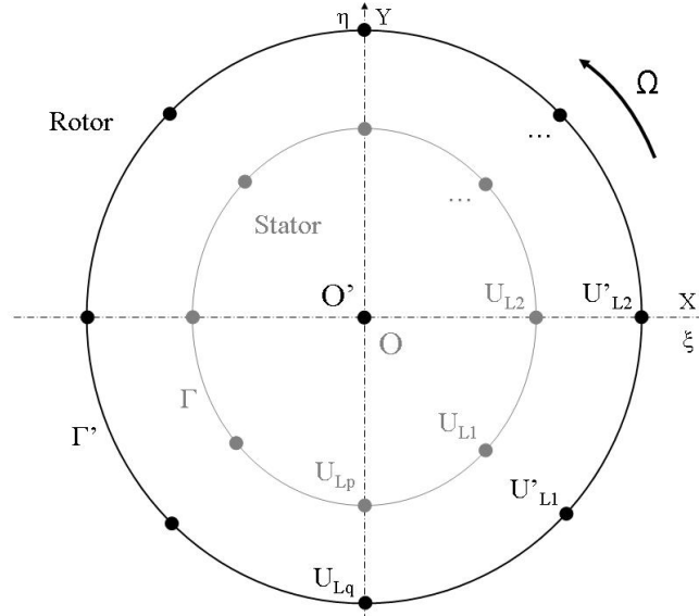
Figure B.2: Représentation schématique des degrés de liberté de liaison physiques
