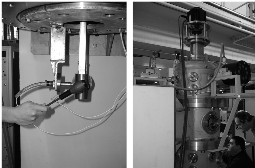
(a) "Marteau de choc" et capteurs
