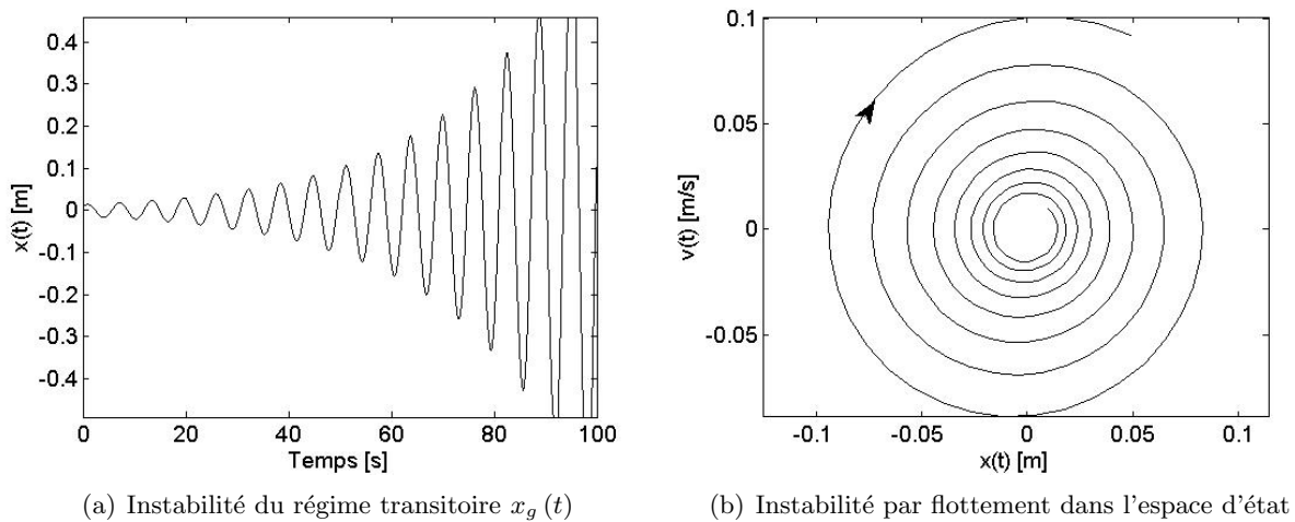
Figure 1.4: Diverses représentations de l'instabilité dynamique pour \zeta = -0.04
