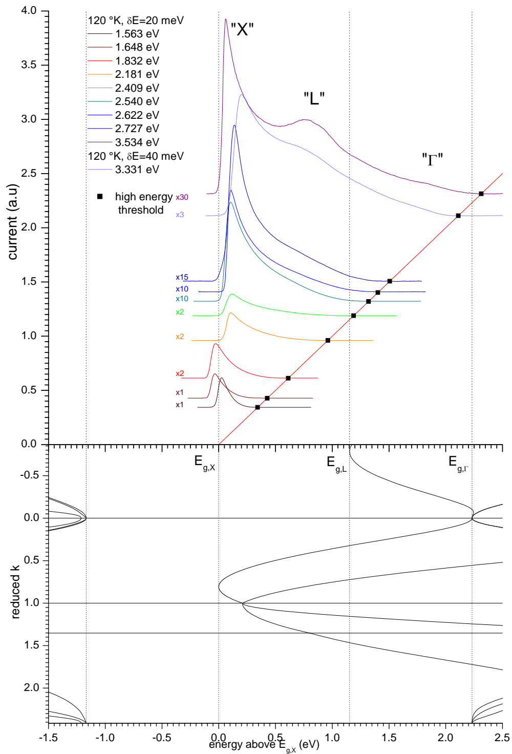
Figure 4-23 : EDC à 120 °K, et haute résolution. Les courbes ont été normalisées par l'aire de la courbe à 1.563 eV, puis multipliées par un facteur choisi pour optimiser la lisibilité de la figure. Le positionnement des EDC est expliqué dans le texte. Les lignes verticales en pointillé représentent la position en énergie des principaux gaps théoriques.
