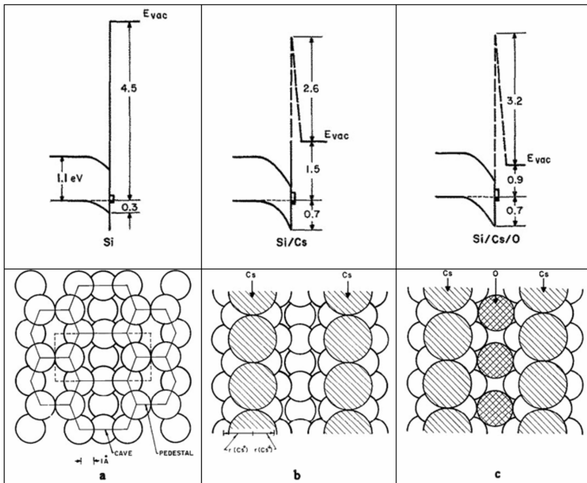
Figure 4-8 : formation d'une couche dipolaire de Cs-O sur une surface de Si 2 \times 1 , d'après le modèle structural de Levine [112] . (a) : surface de Si reconstruite 2 \times 1 obtenue après nettoyage sous UHV. (b) : dépôt d'une demi-couche de Cs sur les sites en piédestal. (c) : insertion des atomes d'oxygène sur les sites en creux. Les moments dipolaires césium-oxygène sont ainsi dirigés vers l'extérieur du cristal.
