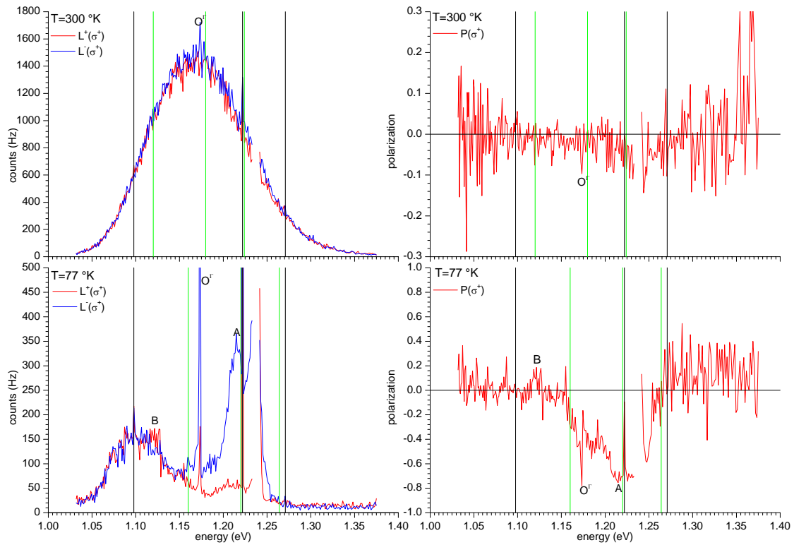
Figure 3-11 : spectres de luminescence de l'échantillon SiA76 sous lumière \sigma^+ d'énergie 1.239 eV, à température ambiante (en haut), et à basse température (en bas).
