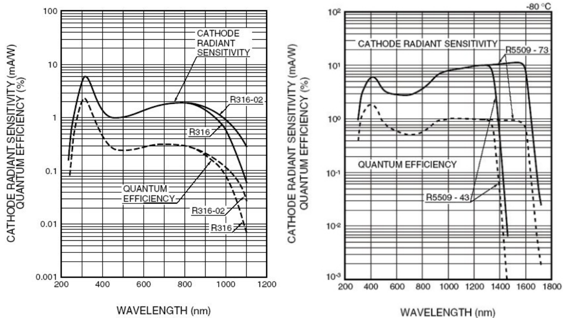
Figure 3-4 : rendements quantiques comparés d'une photocathode S1 (à gauche) et InP/InGaAsP (à droite). Source : Hamamatsu.
