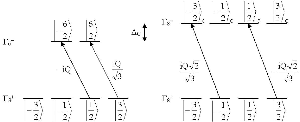
Figure 2-1 : éléments de matrice de p^+ , en lumière \sigma^+ , des transitions à partir de \Gamma_8^+ vers \Gamma_6^- et \Gamma_8^- , séparées par l'énergie de couplage spin-orbite \Delta_C dans la bande de conduction.
