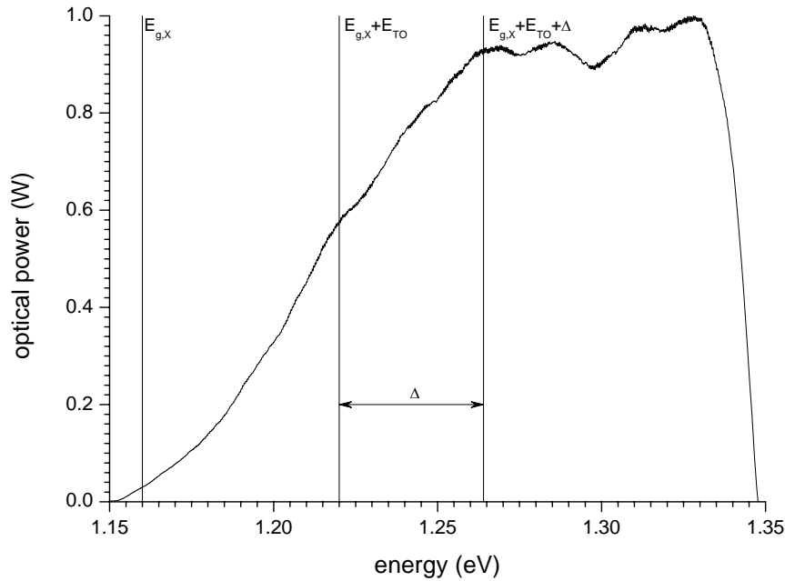
Figure 3-2 : puissance du laser Ti:Al_2O_3 en fonction de l'énergie d'excitation.
