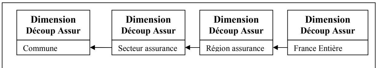
Figure 55 – Schéma de la Dimension « Découpage Assurance »
