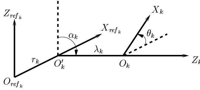
FIG. 6.2: Le paramétrage de Khalil-Kleinfinger décrit le passage du repère ref_k au repère k en effectuant une translation r_k et une rotation \alpha_k le long de l'axe X_{ref_k} , puis une translation \lambda_k et une rotation \theta_k le long de l'axe Z_k .
