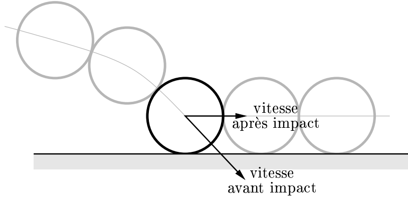
FIG. 2.4: Lorsqu'un solide rentre en contact avec le sol, le fait qu'il ne puisse en aucun cas pénétrer dedans peut nécessiter que sa vitesse soit instantanément déviée, ce qui traduit un impact du solide sur le sol.
