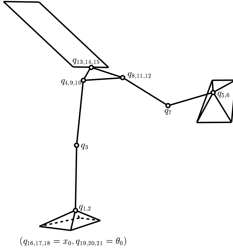
FIG. 1.2: Les positions articulaires q_{1...15} permettent de décrire la posture du robot, tandis que la position et l'orientation q_{16...21} de l'un de ses solides (ici, le pied droit) permettent de déduire son emplacement et son orientation. Le vecteur q_{1...21} ainsi défini décrit alors complètement la position du robot.
