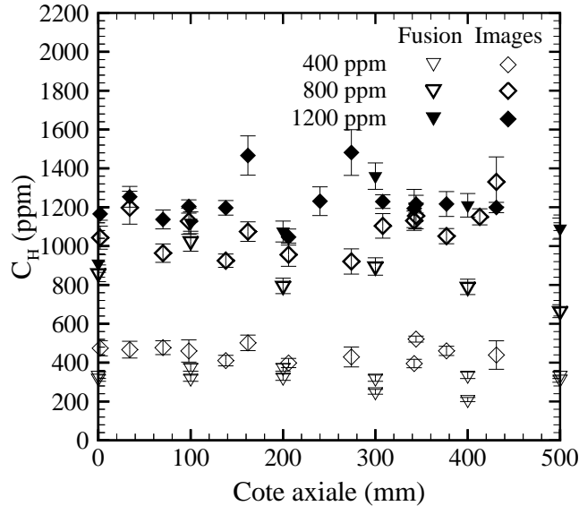
Figure C.2 – Teneurs en hydrogène mesurées pour chaque teneur de consigne (400 ppm, 800 ppm et 1200 ppm) à l'aide d'une méthode de fusion et d'une méthode d'analyse d'images.
