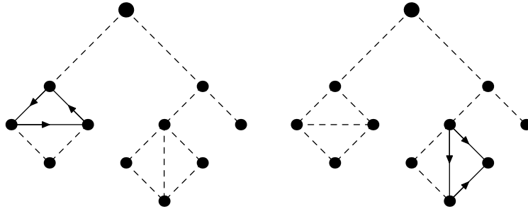
FIG. 1.19 – Exemples de boucle admissible qui ne soit pas de type 1.
