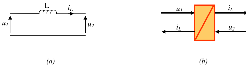
Figure A 6 : Exemple d'une bobine modélisée par le formalisme REM
