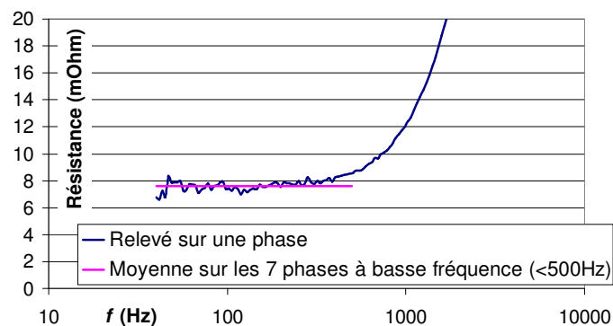
Figure A 20 : Mesure de la résistance d'une phase par un analyseur d'impédance
