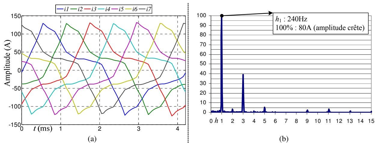
Figure 33 : Courants réels mesurés expérimentalement (a) et décomposition harmonique (b) ; mode alternateur, N = 1800 \text{ tr/min} , i_F = 2,7 \text{ A}
