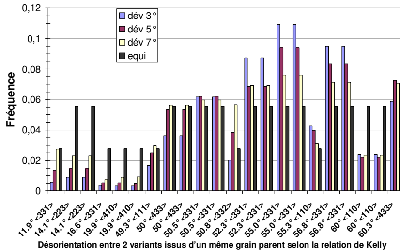
Figure III.32 : Répartition des couples axe/angle minimal de désorientation entre variants du domaine bainitique d'une analyse EBSD réalisée sur l'échantillon non déformé de la campagne de torsion, selon la relation d'orientation de Kelly avec trois angles de tolérance (« dév ») : 3, 5 ou 7°. La répartition équiprobable (notée 'Equi') correspond à une répartition aléatoire des 24 variants présents avec une même proportion. Les paires axe/angle sont désignées à l'aide des indices de Miller approchés.
