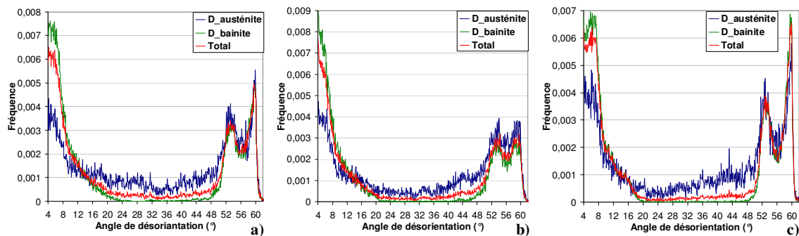
Figure III.15 : Répartition des angles de désorientation minimale d'échantillons des catégories 1 et 2 issue des domaines des anciens joints de grains austénitiques (noté D_austénite , en bleu), bainitique (noté D_bainite , en vert) et de la cartographie entière (noté Total , en rouge) : a) échantillon non déformé de la campagne de torsion, b) échantillon déformé par torsion puis recristallisé, c) transformation isotherme à 560°C avec une austénitisation à 1070°C (560_L).
