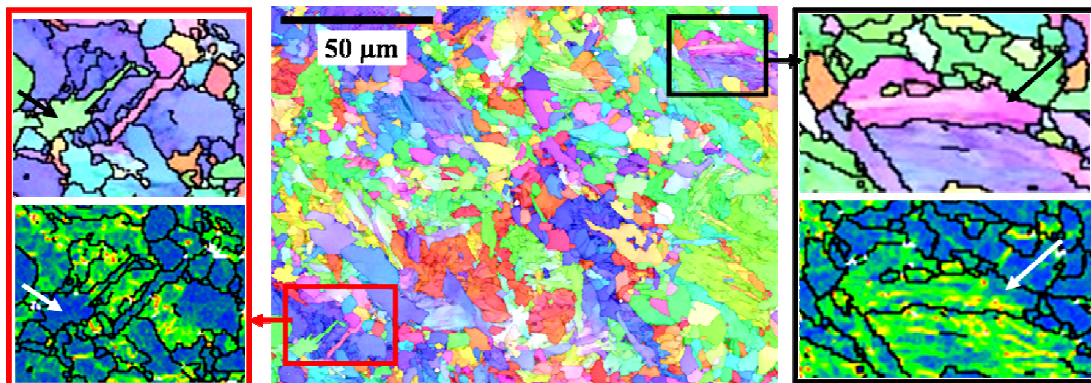
Figure III.21 : Echantillon déformé à 770°C, 1s -1 : au centre, cartographie de l'orientation cristalline avec l'indice de qualité et en encarts des zones de faibles désorientations entre un grain de ferrite équiaxe et un variant de ferrite bainitique (flèches). Les joints en noir présentent une désorientation supérieure à 10°.
