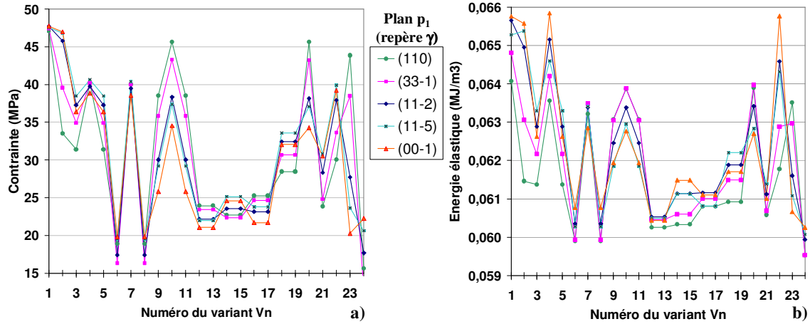
Figure IV.13 : Sensibilité des résultats du modèle au choix du plan de cisaillement p_1 avec comme plan d'habitat \{557\}_\gamma , a) contrainte équivalente dans l'austénite, b) énergie élastique stockée.
