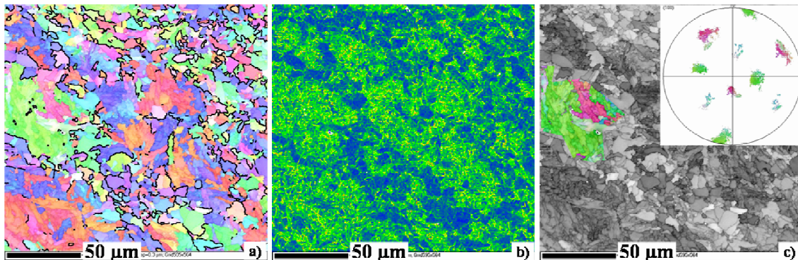
Figure III.17 : Echantillon déformé à 770°C, 1s^{-1} : a) cartographie des joints non endotaxiques, b) cartographie des désorientations locales, c) subset d'un ancien grain d'austénite et la figure de pôles \{001\}_\alpha associée
