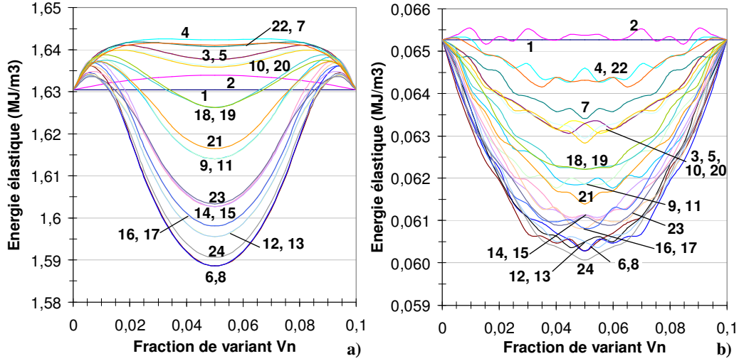
Figure IV.10 : Énergie élastique stockée pour les 24 couples de variants V_1 - V_n avec \{557\}_\gamma comme plan d'habitat et p_1 : (11-5)_\gamma selon : a) Modèle initial, b) Modèle avec les nouvelles lois de comportement
