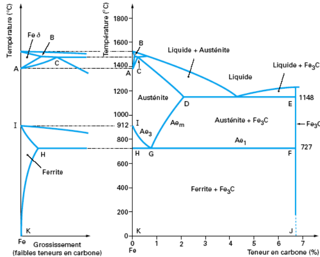
Figure I.1 : Diagramme Fe-Fe 3 C [MUR98], la ferrite CC est notée δ ou α et l'austénite correspond à la structure CFC notée γ
