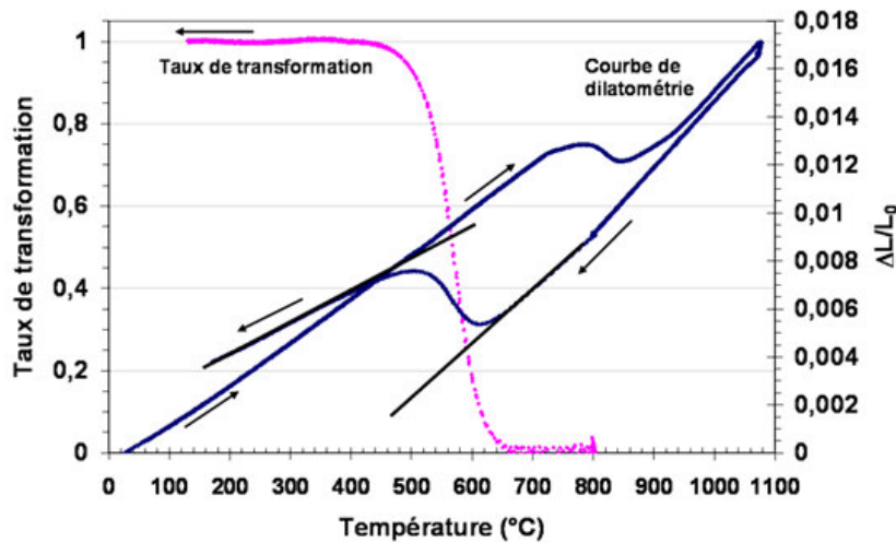
Figure II.4 : Détermination des températures de transformation pour différents taux de bainite formée, à partir de la courbe de dilatométrie pour un refroidissement à 30°C/s.
