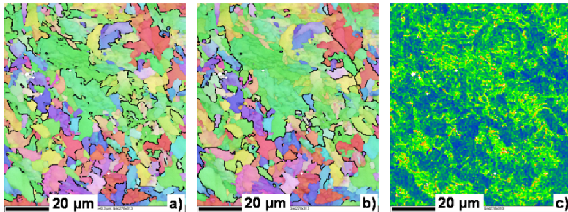
Figure B.1 : Echantillon déformé à 800°C, à 1 s -1 , a) Joints de grains entre variants issus d'un même grain parent selon la relation de Kelly (sauf 4.7°), b) Joints de grains « non endotaxiques», c) Cartographie des désorientations locales
