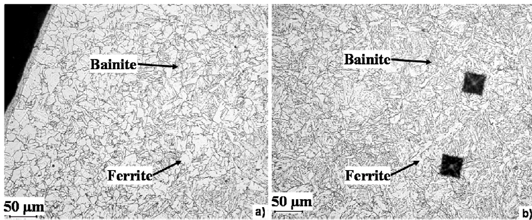
Figure II.19 : Micrographies de l'échantillon déformé à 800°C, 0.1 s -1 a) près de la zone de décarburation, b) au cœur de l'échantillon (attaque au Nital 2%)
