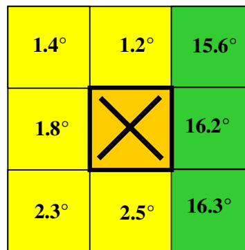
Figure III.2 : Calcul de la désorientation locale en un pixel. Dans ce cas, la désorientation locale pour le pixel étudié (localisé par une croix) est de 1.8^\circ (c'est-à-dire égale à (1.2 + 1.4 + 1.8 + 2.3 + 2.5) / 5 )
