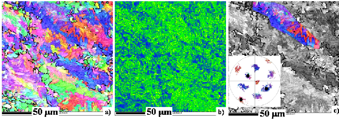
Figure III.18 : Echantillon déformé à 800°C, 10s -1 : a) cartographie des joints non endotaxiques, b) cartographie des désorientations locales, c) subset d'un ancien grain d'austénite et la figure de pôles {001} α associée
