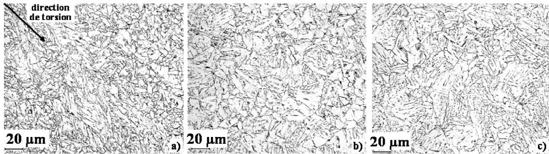
Figure III.3 : Micrographies en microscopie optique après attaque nital 2%, des échantillons a) déformé à 800°C, 0.1s -1 , b) déformé à 1000°C, 1s -1 suivi d'un palier de recristallisation, c) non déformé. Les micrographies a) et b) ont été réalisées au centre de méplats.
