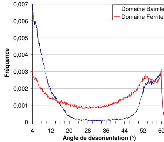
Figure III.26 : Répartition des angles de désorientation sur la moyenne des domaines de ferrite équiaxe et bainitique des échantillons déformés dans le domaine austénitique au-dessous de T_m .
