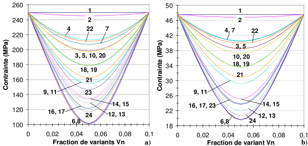
Figure IV.9 : Contrainte équivalente dans l'austénite pour les 24 couples de variants V_I - V_n avec \{557\}_\gamma comme plan d'habitat et p_1 : (11-5)_\gamma selon a) la modèle initial, et b) le modèle avec les nouvelles lois de comportement
