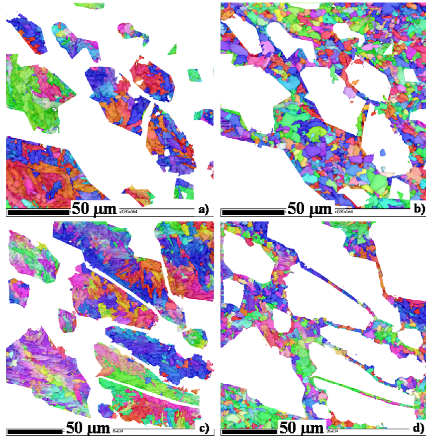
Figure III.19 : Domaines bainitiques (a, c) et ferritiques (b, d) des échantillons déformés à 770°C, 1s -1 (a, b), et à 800°C, 10s -1 (c, d).
