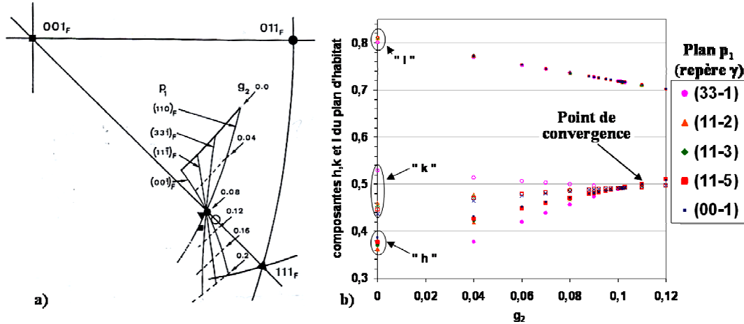
Figure IV.4 : Variation de la solution pour le plan d'habitat pour différents plans p_1 avec : a) S_2 : (100)[0-11]_\gamma [KEL92], b) S_2 : (511) [0-11]_\gamma
