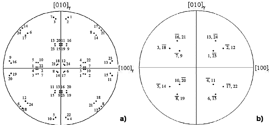
Figure IV.8 : Figure de pôles \{100\}_\alpha (a) et plans d'habitat \{557\}_\gamma (b) des 24 variants de phase fille, dans le repère de l'austénite mère.
