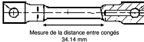
Figure II.13 : Zone de mesure de la distance entre congés des éprouvettes de torsion
