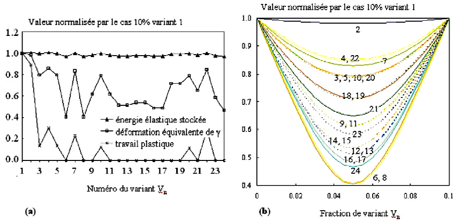
Figure 1.33 : Résultats du modèle micromécanique pour les 24 couples ( V_I , V_n ) possibles, a) pour 5% de chaque variant V_I et V_n en fonction du choix de V_n et b) contrainte équivalente dans l'austénite, pour 10% d'austénite transformée, en fonction de la fraction de variant V_n . Les courbes sont repérées par l'identité du variant n . [GOU03]
