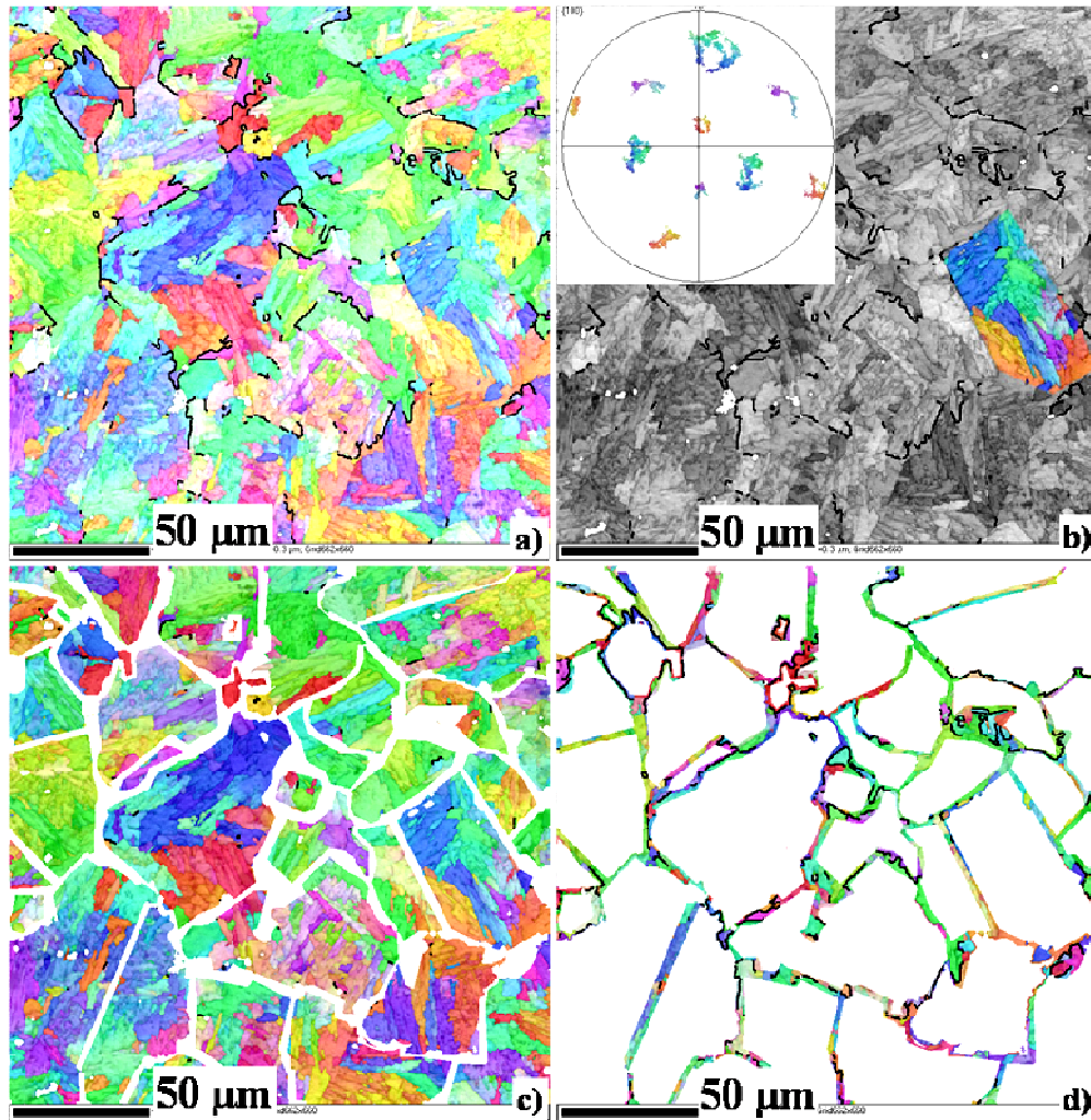
Figure III.14 : Echantillon non déformé de la compagne de torsion : a) cartographie EBSD des joints « non endotaxiques » avec l'orientation cristalline et l'indice de qualité, b) subset supposé d'un ancien austénitique et en encart la figure de pôles \{001\}_\alpha associée, c) en coloré le domaine bainitique, d) en coloré le domaine des « anciens joints austénitiques » avec les joints non-endotaxiques en noir.
