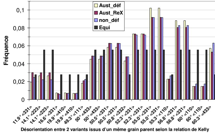
Figure III.36 : Répartition des couples axe/angle de désorientation selon la relation de Kelly pour les 3 types d'échantillons de torsion non déformé, recristallisé et déformé. Les barres noires représentent la répartition équiprobable.
