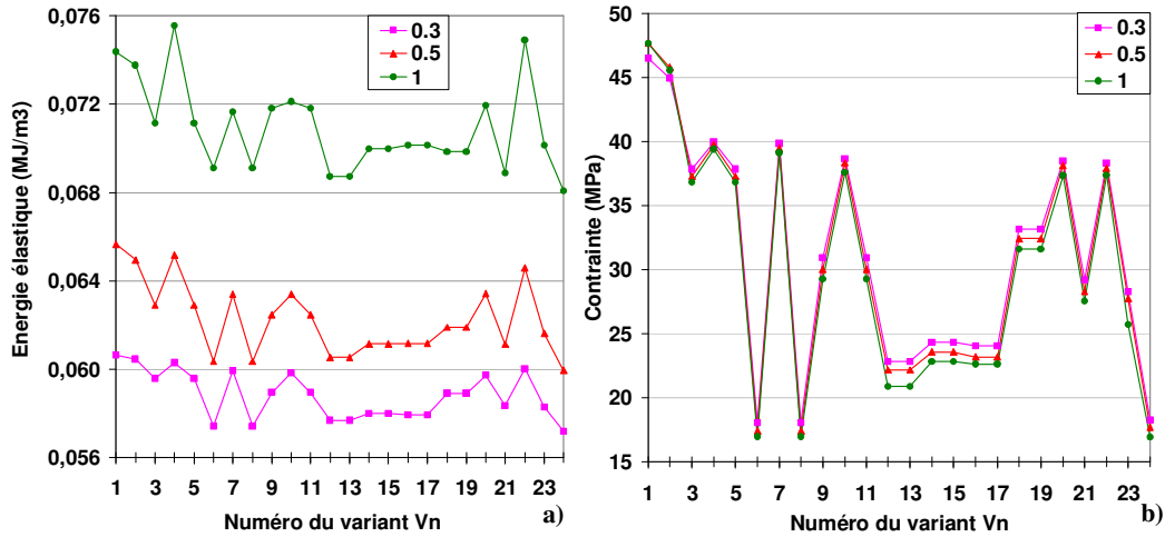
Figure IV.16 : Influence du facteur d'amplification sur a) l'énergie élastique stockée, b) la contrainte équivalente dans l'austénite pour un plan d'habitat de type \{557\}_\gamma et p_1 = (11-2)_\gamma
