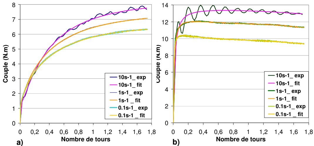
Figure II.24 : Exemple de lissage (courbes notées "fit") des courbes expérimentales du couple en fonction du nombre de tours a) des échantillons déformés dans l'austénite à 770°C, b) des échantillons déformés dans le domaine bainitique à 630°C.
