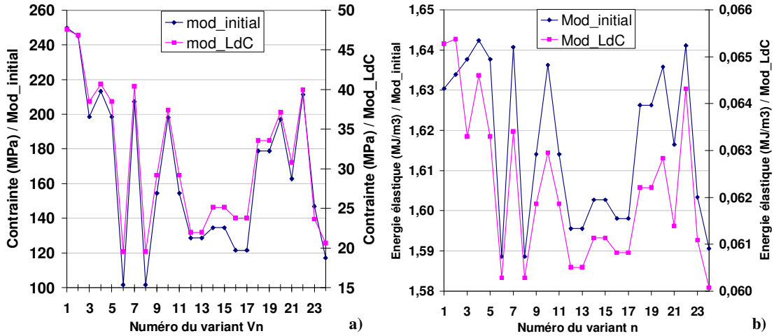
Figure IV.11 : a) Contrainte équivalente dans l'austénite et b) énergie élastique stockée pour 5% de variant V_1 et 5% de variant V_n en fonction du choix de V_n avec \{557\}_\gamma comme plan d'habitat et p_1 : (11-5)_\gamma .
