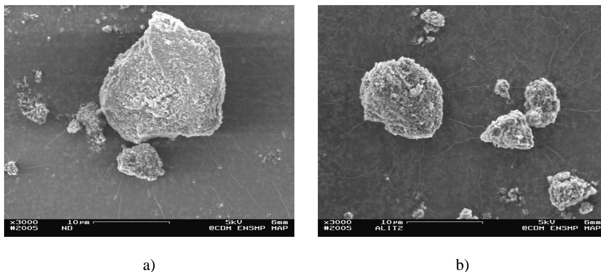
Fig. III.4 – Micrographies des nanodiamants U.D.D.G a) et U.D.D b)
