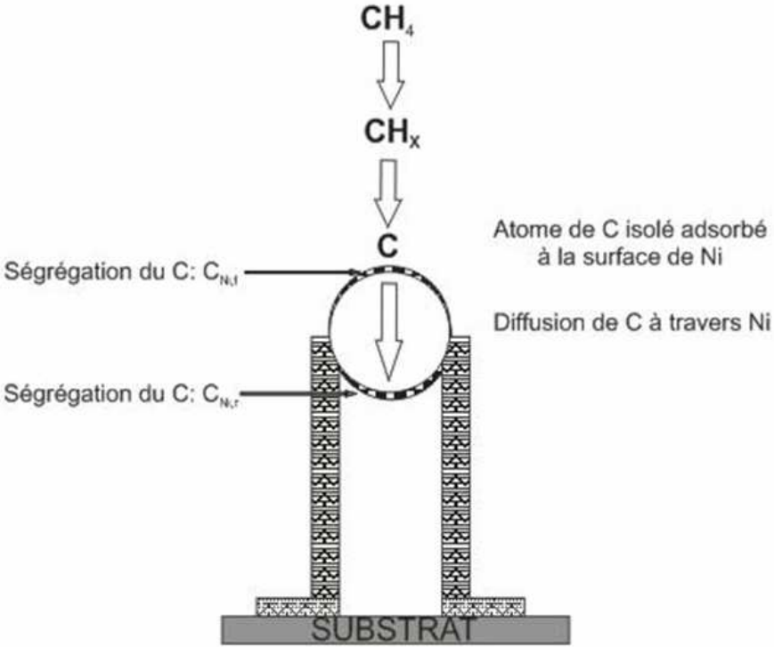
Fig. I.7 – Modèle de croissance de nanotube de carbone de Snoeck [7]
