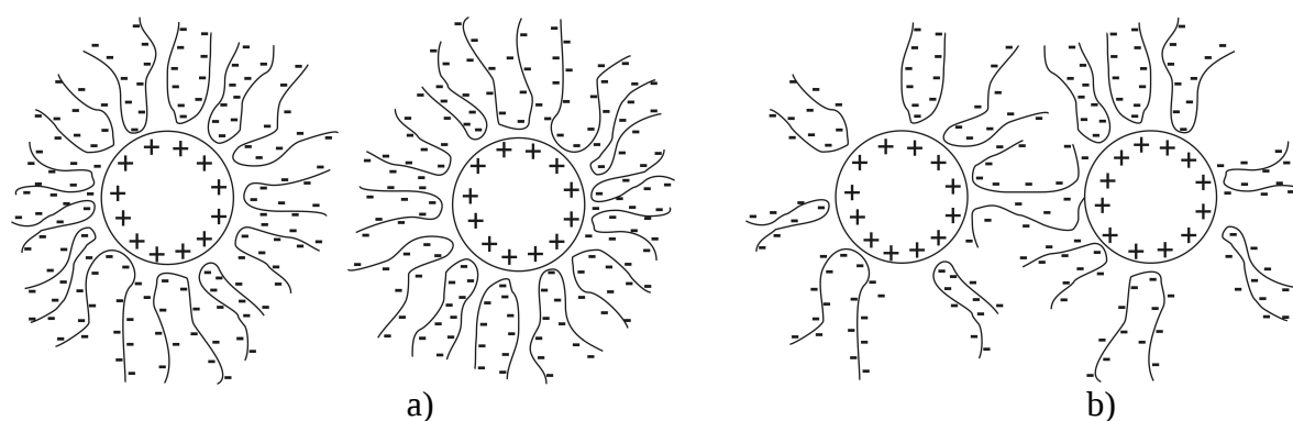
Fig. II.3 – Encombrement stérique a) et ponts b) créés par les chaînes du dispersant
