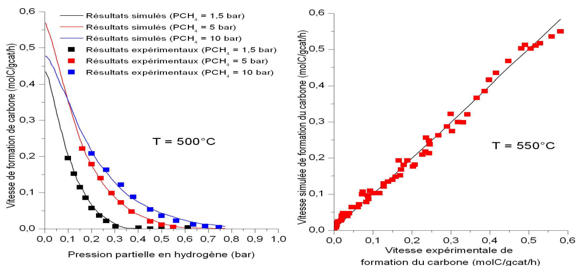
Fig. 1.9 – Comparaison entre le modèle de Snoeck et les résultats expérimentaux [7]
