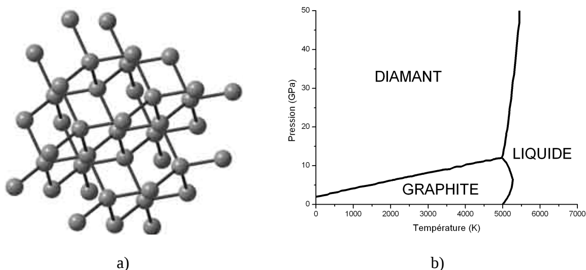
Fig. III.1 – a) Structure cristalline du diamant b) Diagramme de stabilité du diamant
