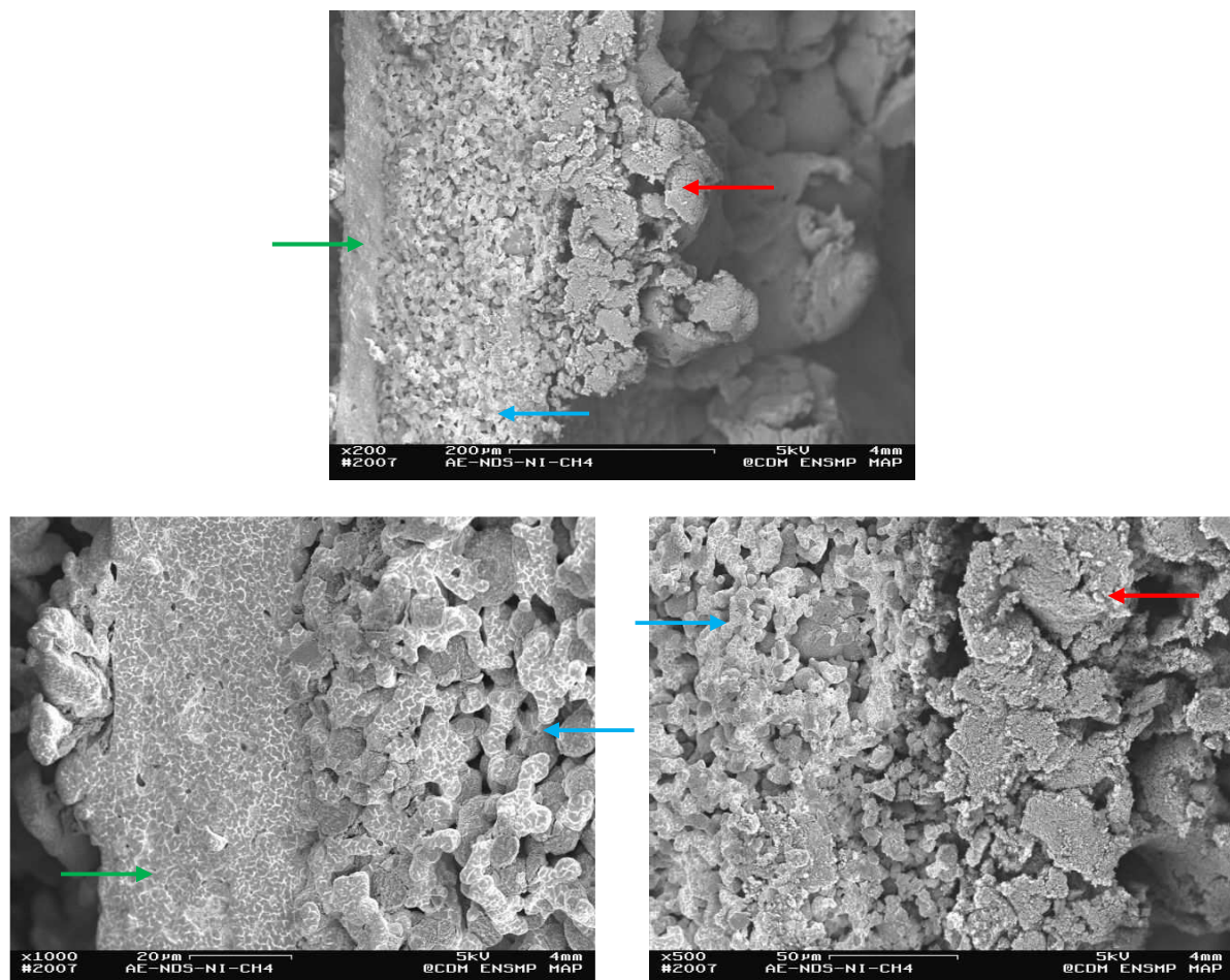
Fig. V.19 – Anode de P.C.F.C à reformage interne et séquestration de carbone
