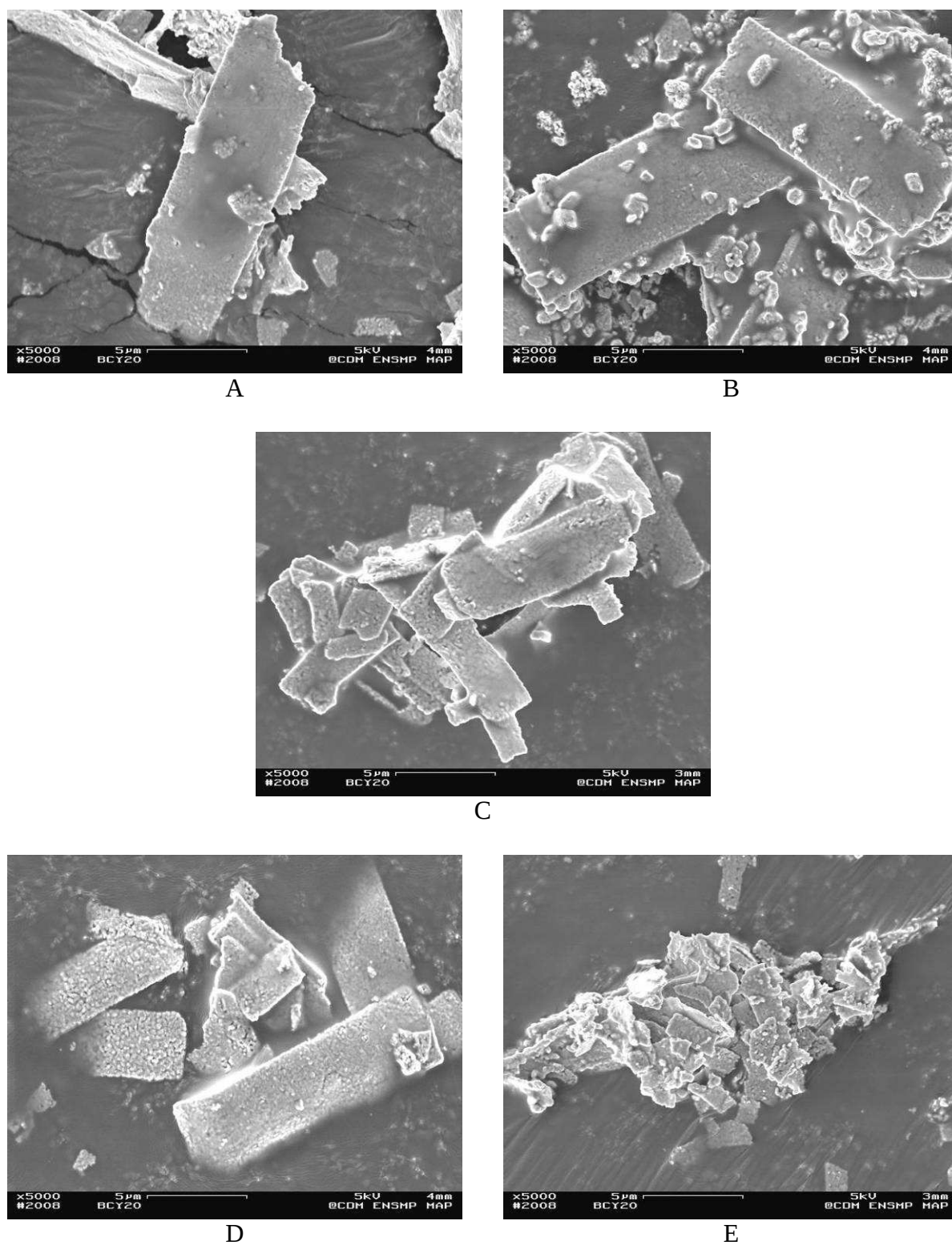
Fig. IV.31 – BZY 20 obtenus avec différentes concentrations (cf. Tab.VI.12)
