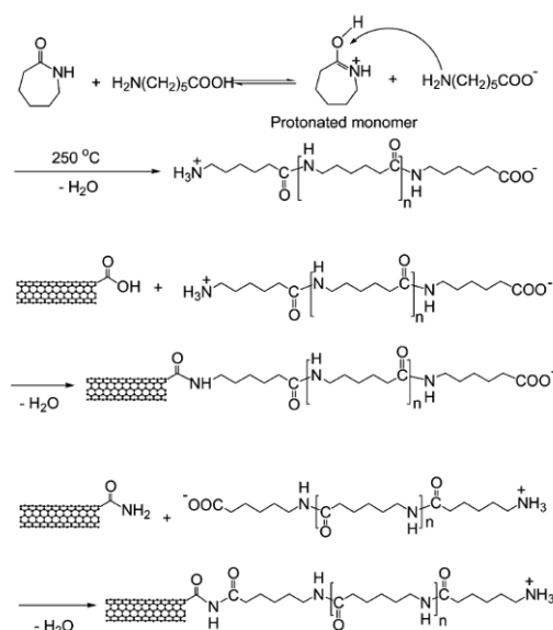
Figure 1-14 : Synthèse de composite SWNTs/PA-6 avec des nanotubes fonctionnalisés COOH et CONH 2 . 65
