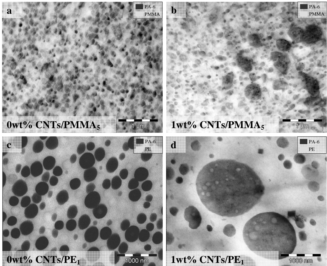
Figure A7-7 : Images TEM des composites a) \text{PMMA}_5\text{-30PA6}^{15} b) \text{PMMA}_5\text{-1NT-30PA6}^{15} c) \text{PE}_1\text{-30PA6}^{15} d) \text{PE}_1\text{-1NT-30PA6}^{15} . (Marquage : acide phosphotungstique)
