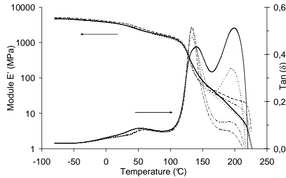
Figure A7-13 : Analyse dynamique mécanique (module E' et \tan(\delta) ) des composites \text{PMMA}_2\text{-30PA6}^{15} (—), \text{PMMA}_2\text{-1NT-30PA6}^{15} (----), \text{PMMA}_7\text{-30PA6}^{15} (— —), \text{PMMA}_7\text{-1NT-30PA6}^{15} (— — —).
