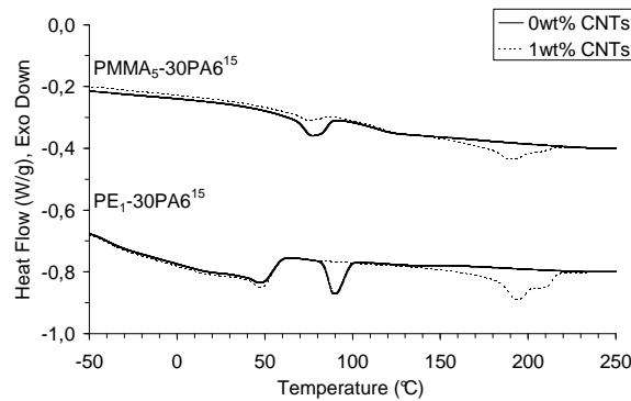
Figure A7-8 : Thermogrammes au refroidissement des composites PMMA 5 -30PA6 15 et PE 1 -30PA6 15 avec 0 et 1 wt% de CNTs. ( v = 10 \text{ }^\circ\text{C}/\text{min} )
