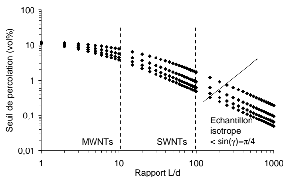
Figure 1-24 : Prédiction du seuil de conductivité pour des charges droites en fonction du rapport L/d et pour différents états d'orientation.
