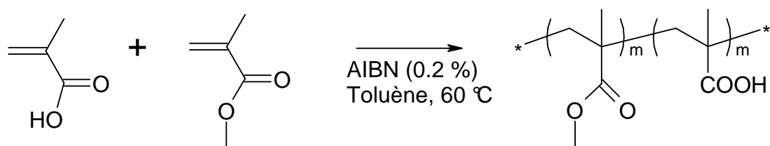
Figure A6-1 : Synthèse du P(MMA-co-MAA) avec 2 % d'acide méthacrylate.
