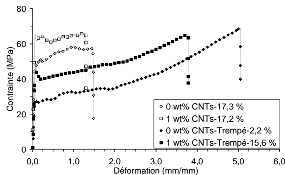
Figure 3-23 : Courbes de traction des composites PA6 15 -0NT-200 et PA6 15 -1NTp-200 après une trempé et un refroidissement à « vitesse modérée », le pourcentage dans la légende est le taux de cristallinité.
