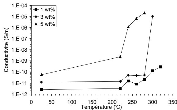
Figure 4-14 : Evolution de la conductivité dans les composites PA6 15 -NTp-200 à différents pourcentages en fonction de la température après un maintien de 40 min à cette température.
