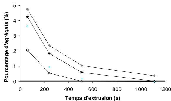
Figure 3-4 : Evolution du pourcentage d'agrégats en fonction du temps pour le composite PA6 15 -1NT extrudé dans différentes conditions à 250 °C, 100 rpm (◆) 250 °C, 200 rpm (mélange poudres) (◇) et 300 °C, 100 rpm(◆) et la limite de détection (—).
