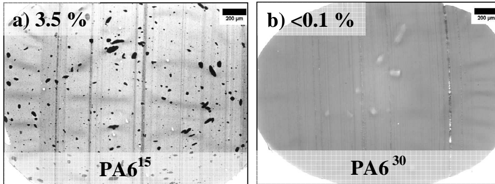
Figure 6-4 : Photos de microscopie optique d'un mélange PA6-3NT-9S 14 11 B 19 M 67 S-100 avec a) PA6 15 b) PA6 30 . Le nombre dans l'insert correspond au S CNTs (%).
