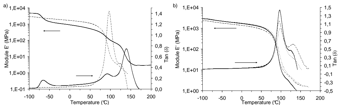
Figure A4-2 : Analyse dynamique mécanique (module E' et \tan(\delta) )
