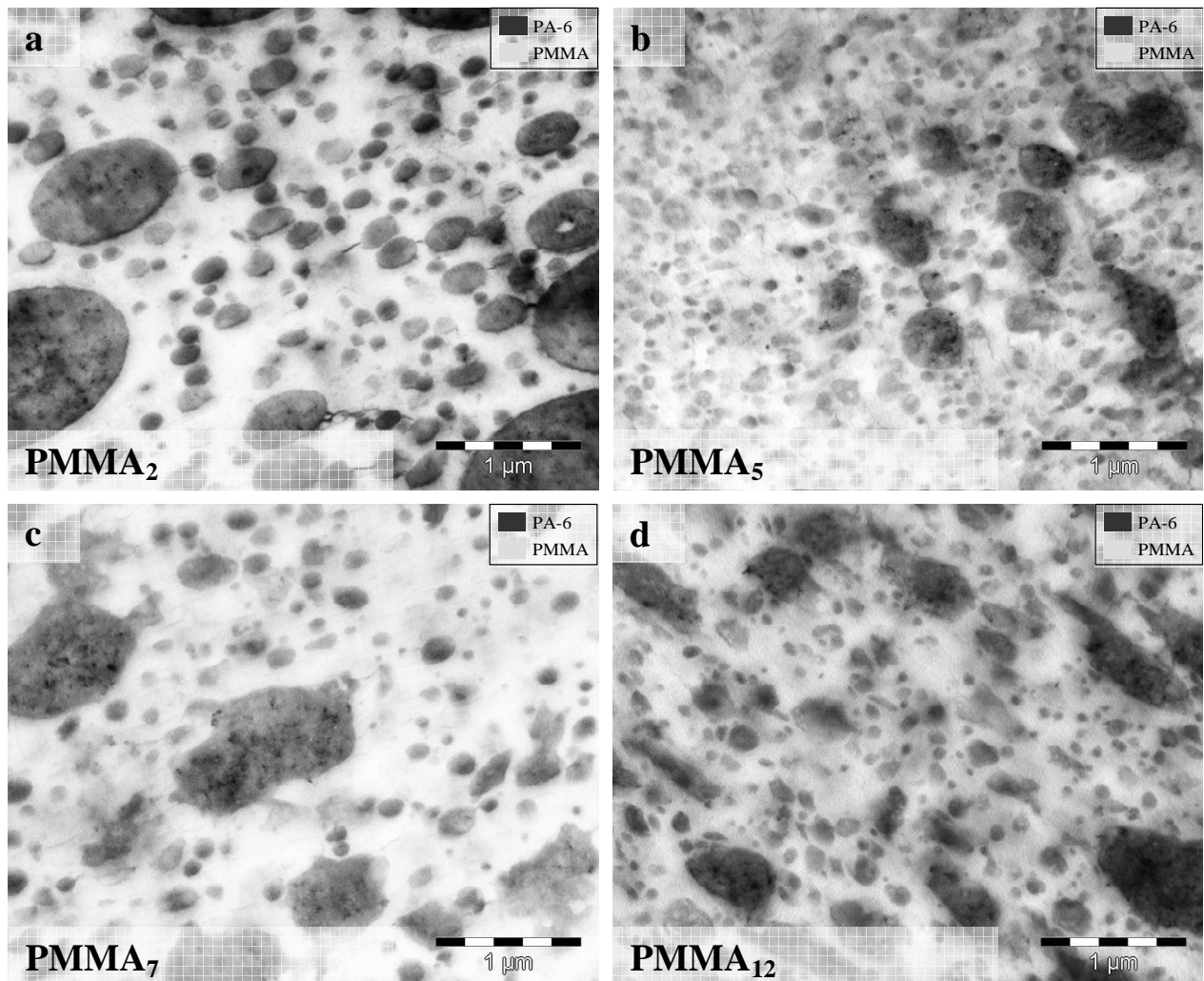
Figure A7-10 : Images TEM des composites a) \text{PMMA}_2\text{-1NT-30PA6}^{15} b) \text{PMMA}_5\text{-1NT-30PA6}^{15} c) \text{PMMA}_7\text{-1NT-30PA6}^{15} d) \text{PMMA}_{12}\text{-1NT-30PA6}^{15} . (Marquage : Acide phosphotungstique)
