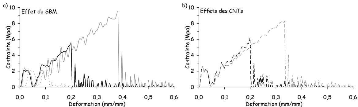
Figure 6-22 : Choc Charpy sur les composites en a) PA6 15 -30S 14 11 B 19 M 67 -200 (—), PA6 15 -200 (⋯), PA6 15 -30S 36 15 B 11 M 53 -200 (— —) b) PA6 15 -1NT-200 (—), PA6 15 -1NT-30S 14 11 B 19 M 67 -200 (— —).
