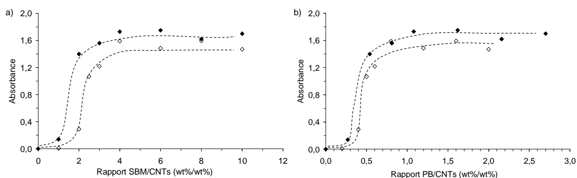
Figure 5-7 : Absorbance UV-visible pour le S_{14}^{11}B_{19}M_{67} brut (◆) et purifié (◇) a)-en fonction du rapport massique SBM/CNTs b)-en fonction du rapport massique PB/CNTs.
