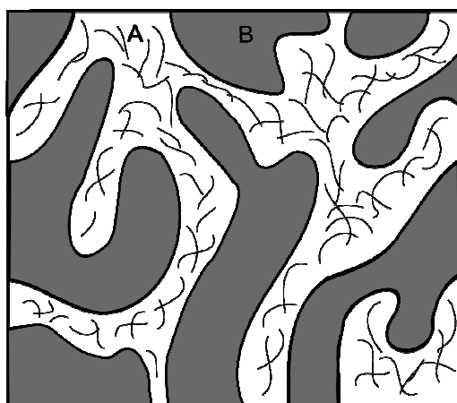
Figure 1-28 : Schéma de la double percolation, localisation des CNTs dans la phase A continu.
