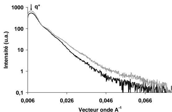
Figure 5-16 : Spectre de diffusion aux petits angles des films de S_{14}^{11}B_{19}M_{67} évaporés dans l'acétone avec 0 (—) et 1 (---) wt% de CNTs.
