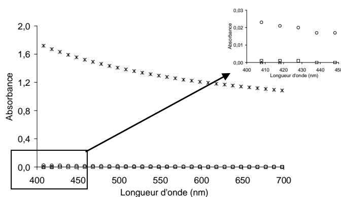
Figure 5-1 : Absorbance UV-visible de l'acétone (□), du \text{CHCl}_3 (△), d'une solution d'acétone avec 1 wt% de \text{S}_{14}^{11}\text{B}_{19}\text{M}_{67} (○) et avec 1 wt% de \text{S}_{14}^{11}\text{B}_{19}\text{M}_{67} plus 0,1 wt% de CNTs (*).
