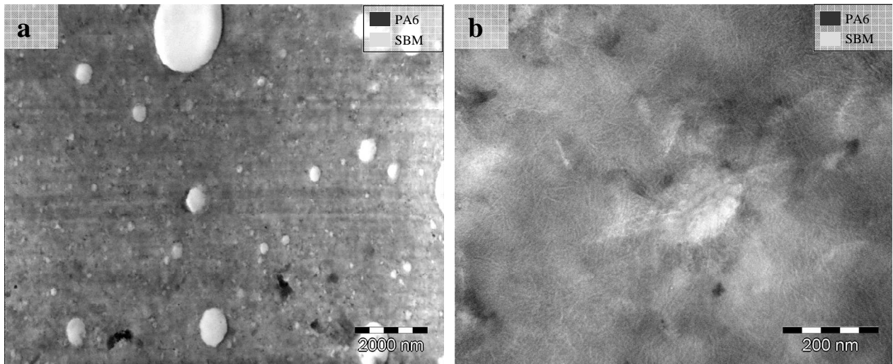
Figure 6-19 : Image TEM du composite PA6 15 -3NT-9S 23 5 B 7 M 70 -100 avec deux grandissements différents en coupe // (Marquage: acide phosphotungstique)
