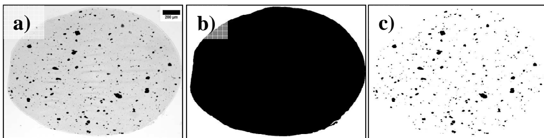
Figure 3-1 : Traitement d'une photo en microscopie optique a) Image initiale b) Surface du jonc ( S_0 ) c) Surface des agrégats de CNTs ( S_{AG} ).
