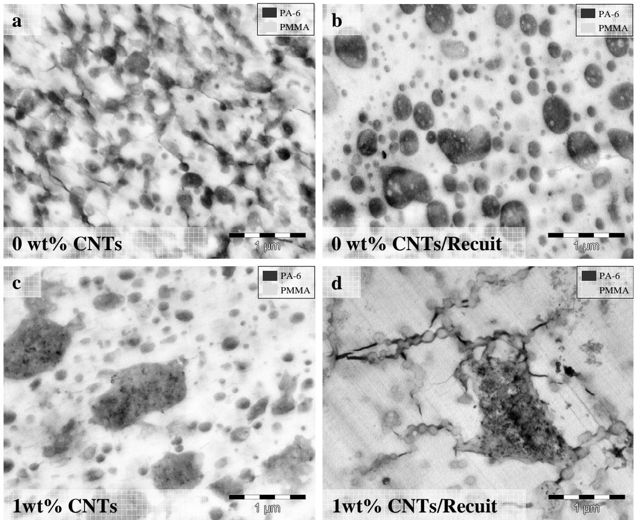
Figure A7-12 : Images TEM des composites a) \text{PMMA}_7\text{-30PA6}^{15} b) \text{PMMA}_7\text{-30PA6}^{15} -recuit c) \text{PMMA}_7\text{-1NT-30PA6}^{15} d) \text{PMMA}_7\text{-1NT-30PA6}^{15} -recuit. (Marquage : Acide phosphotungstique)
