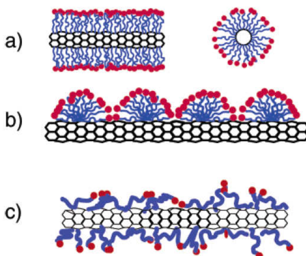
Figure 1-8 : Représentation possible de l'organisation des surfactants à la surface des CNTs a) Organisation en cylindre, b) Organisation en hemimicelles, c) Couche adsorbée aléatoire non organisée. 40
