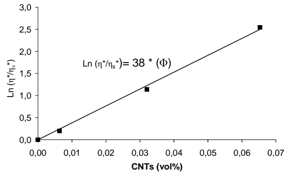
Figure 6-6 : Viscosité pour le composite S_{14}^{11}B_{19}M_{67}\text{-NT-100} (■) à différentes concentrations en CNTs et ajustement avec l'équation (—).
