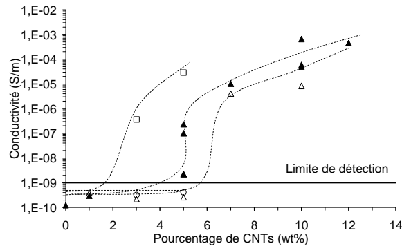
Figure 6-15 : Conductivité des composites PA6 15 -NT-100 (▲), PA6 15 -NTp-200 (△), PA6 15 -NT-S 36 15 B 11 M 53 -100 (□), PA6 15 -NT-PA6 15 -100 (○).
