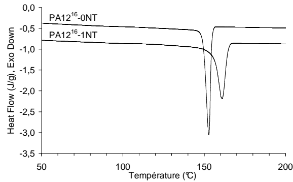
Figure 3-18 : Thermogrammes au refroidissement des composites PA12 16 -NT avec 0 ou 1 wt% de CNTs. ( v = 10 \text{ }^\circ\text{C}/\text{min} )
