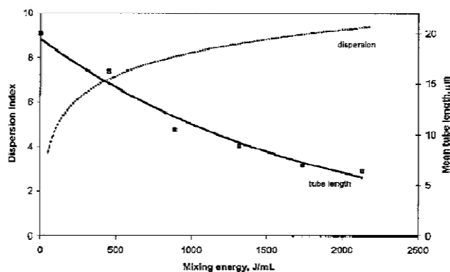
Figure 1-13 : Diminution de la longueur et augmentation de l'état de dispersion avec l'énergie de mélange. 58
