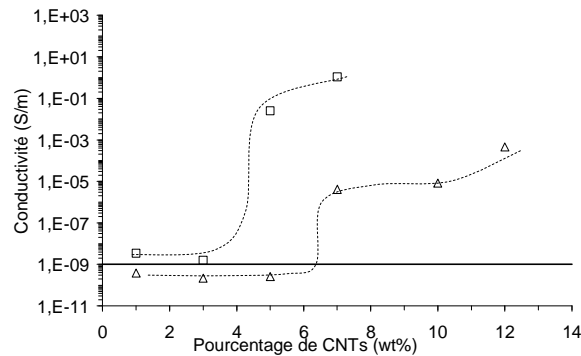
Figure 4-23 : Conductivité pour les composites PA-6/CNTs ( \Delta ) et PMMA/CNTs ( \square ).
