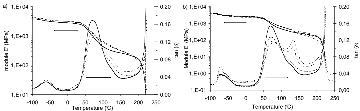
Figure 6-21 : Analyse dynamique mécanique (module E' et \tan(\delta) ) a) des composites PA6 15 -NT-S 36 15 B 11 M 53 -100 préparés par voie fondu avec différents pourcentages de CNTs 0 wt% (—), 1 wt% (— —), 5 wt% (— — — —) b) des composites PA6 15 -NT-S 14 11 B 19 M 67s -100 préparés par voie solvant avec différents pourcentages de CNTs 0 wt% (—), 1 wt% (— —), 3 wt% (— — — —), 4 wt%(— — — —).
