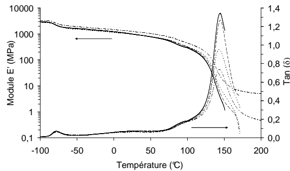
Figure 5-20 : Analyse dynamique mécanique (module E' et Tan ( \delta )) des films de S_{14}^{11}B_{19}M_{67} -NTs évaporés à partir d'une solution dans l'acétone avec différentes concentrations de CNTs : 0 wt% (—), 1 wt% (— —), 5 wt% (— — —), 10 wt% (— — — —).
