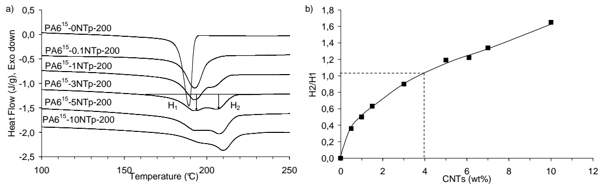
Figure 3-7 : a) Thermogrammes des composites PA6 15 -NTP-200 avec différents taux de charges au refroidissement b) Rapport H_2/H_1 en fonction du pourcentage de CNTs.
