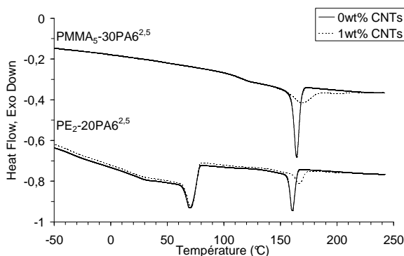
Figure A7-5 : Thermogrammes au refroidissement des composites PMMA 5 -30PA6 2.5 et PE 2 -20PA6 2.5 avec 0 et 1 wt% de CNTs. ( v = 10 °C/min)
