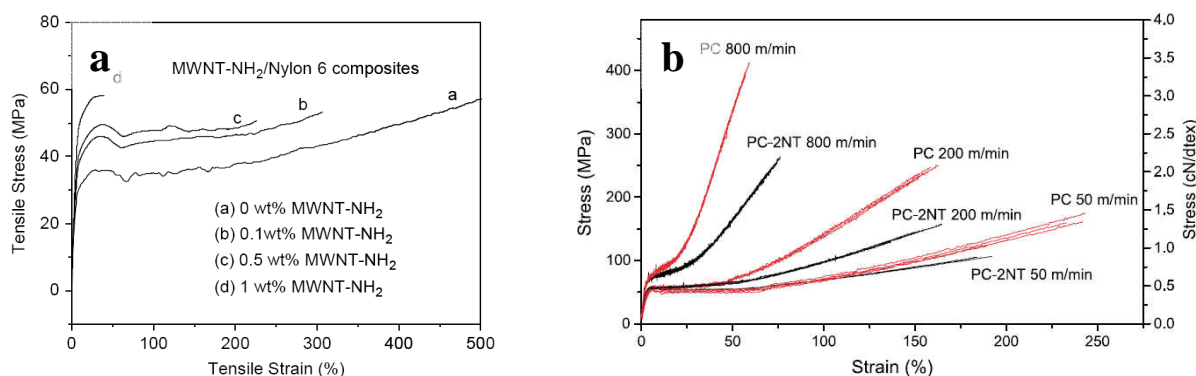
Figure 1-15 : a) Contrainte en fonction de la déformation pour un composite PA-6/MWNTs greffé NH 2 avec différents pourcentage des MWNTs 62 b) Contrainte en fonction de la déformation pour des fibres de polycarbonate avec 2 wt% de MWNTs pour différents étirements. 70
