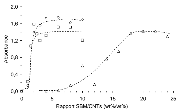
Figure 5-5 : Absorbance UV-visible pour différents SBM, le S_{14}^{11}B_{19}M_{67} (◇), le S_{24}^{11}B_{31}M_{45} (□) et le S_{36}^{15}B_{11}M_{53} (△) en fonction du rapport massique SBM/CNTs.
