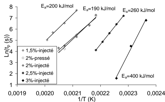
Figure 4-11 : Evolution du temps caractéristique « t p » en fonction de la température pour les composés PMMA 49 -NT à différentes concentrations.
