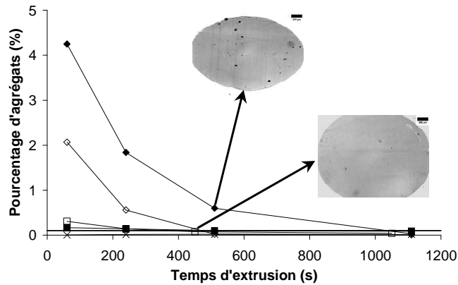
Figure 6-1: Pourcentage d'agrégats en fonction de la durée d'extrusion pour les composites PA6 15 -1NT-100 (◆), PA6 15 -1NT-200 (◇), PA6 15 -1NT-9S 14 11 B 19 M 67 -100 (■), PA6 15 -1NT-9S 14 11 B 19 M 67 S-100 (□) et PA6 15 -1NT-9PA6 15 -100 (×).
