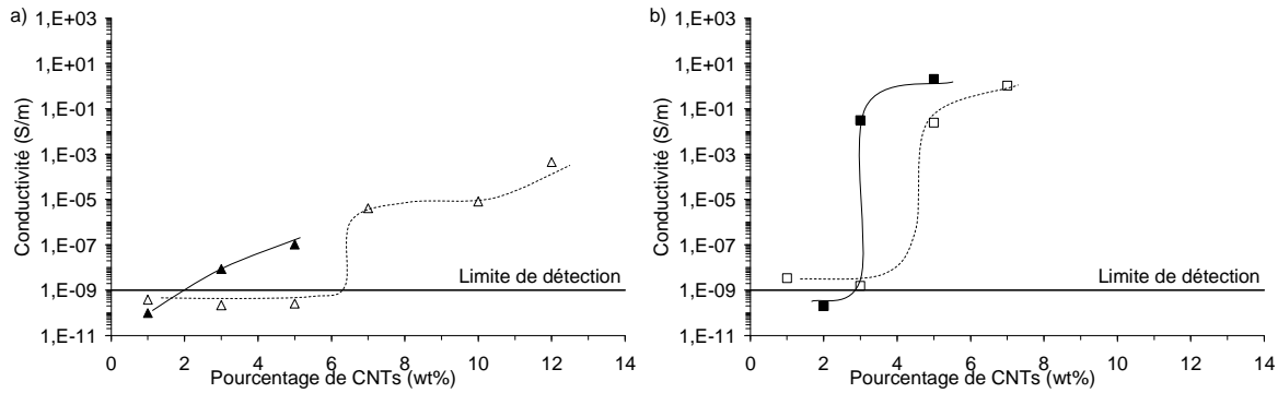
Figure 4-19 : Conductivité pour les composites : a) PA6 15 -NTp-200 extrudés à deux température différentes 250 °C (△) et 300 °C (▲) b) PMMA 49 -NTp-200 extrudés à deux températures différentes 190 °C (□) et 250 °C (■).
