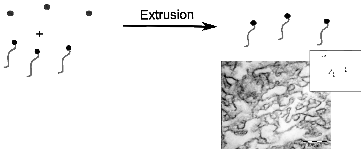
Figure A7-1 : Alliage nanostructuré PE/PA-6 obtenu par extrusion réactive. Image TEM (PE blanc, PA6 noir) et représentation schématique de la phase co-continue.
