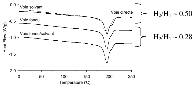
Figure 6-12 : Thermogramme au refroidissement des composites PA6 15 -1NT-9S 14 11 B 19 M 67 -100 (—) correspondant à différents modes de préparation indiqués sur la figure, PA6 15 -1NT-200 (— —). ( v = 10 \text{ }^\circ\text{C}/\text{min} )
