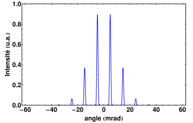
Champ lointain du mode hors phase (n=10)
