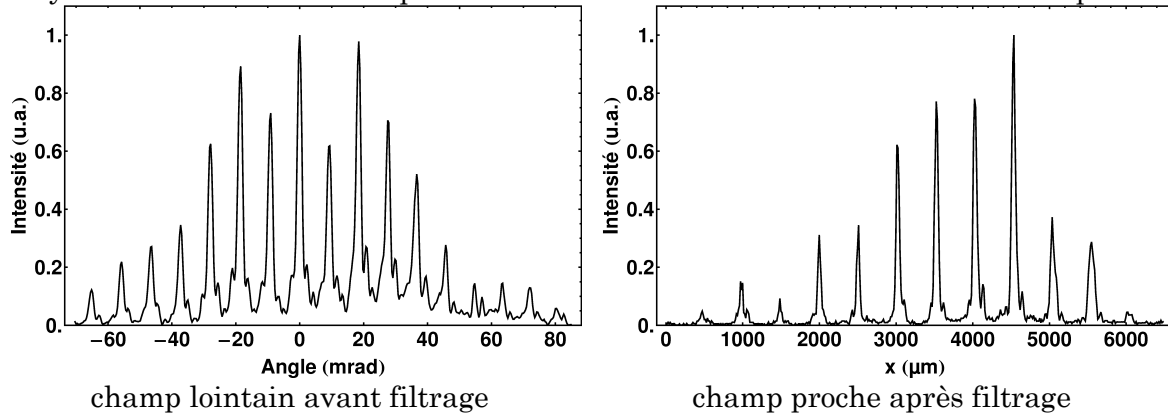
Figure IV-21 : Profils en champ lointain avant filtrage (gauche) et en champ proche après filtrage pour le mode en phase – I = 1,4 A.
