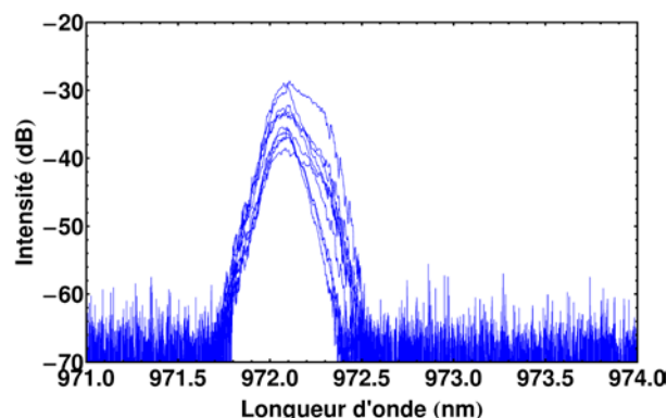
Figure III-14 : Spectre de chaque émetteur mesuré à l'analyseur de spectre optique - R_{\text{RdB}} = 40 \% @ 972 nm, barrette 10IG1-I-5, I = 3 \text{ A} , P = 1,1 \text{ W} , mode en phase, résolution de l'analyseur de spectre: 10 pm.
