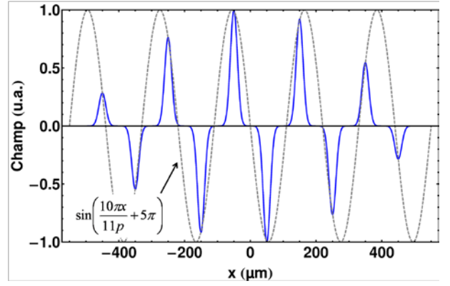
Champ proche du mode hors phase (n=10)
