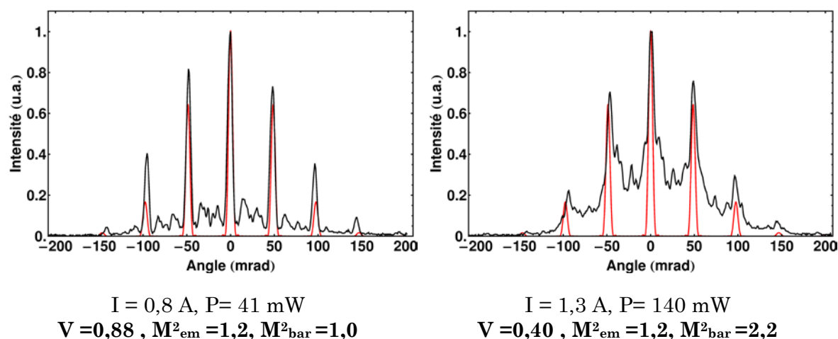
Figure III-21 : Profils en champ lointain en fonction du courant d'alimentation, gauche : près du seuil, droite : I = 1,6 \times I_{seuil} . 1
