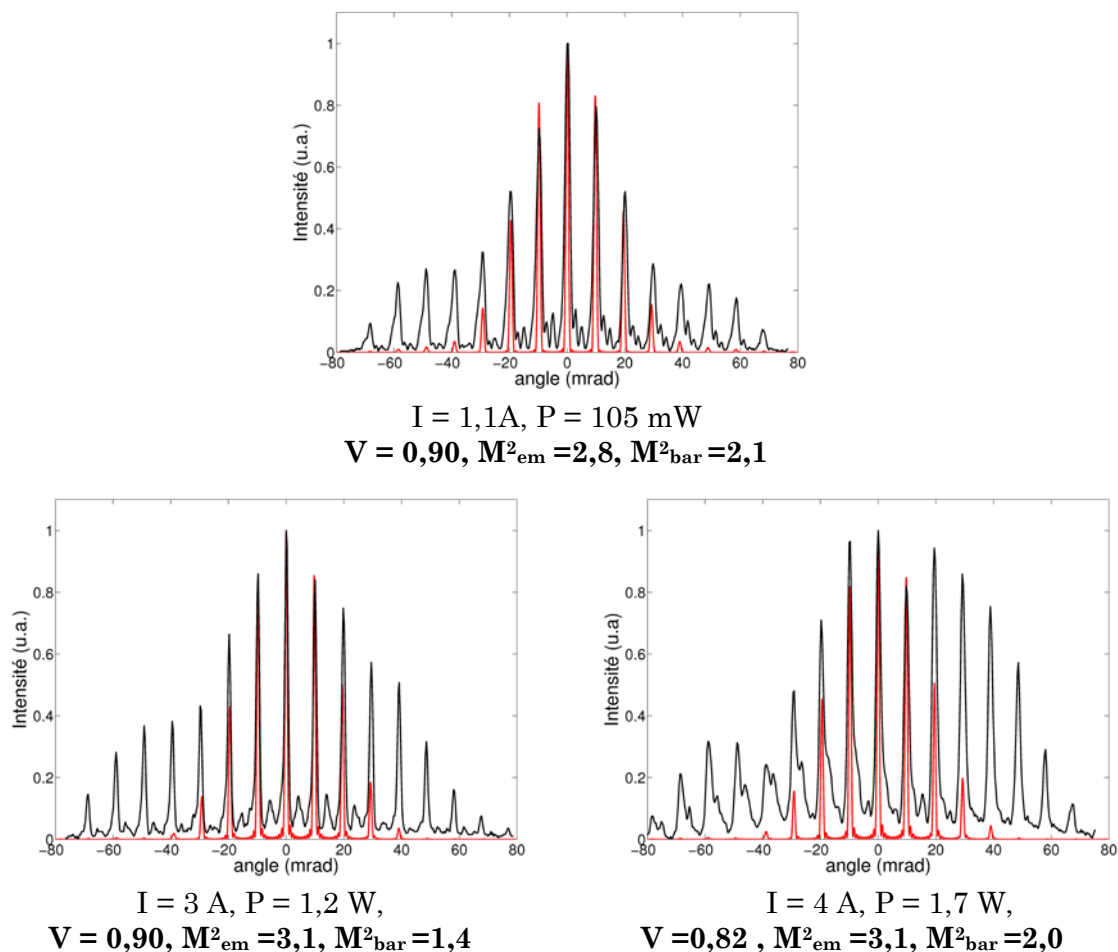
Figure III-19 : Evolution des profils en champ lointain avec le courant d'alimentation– noir : mesures expérimentales, rouge : champs lointains simulés avec le modèle UNott – barrette 10IG1-I-5, R_{dB} = 40\% à 976 nm.
