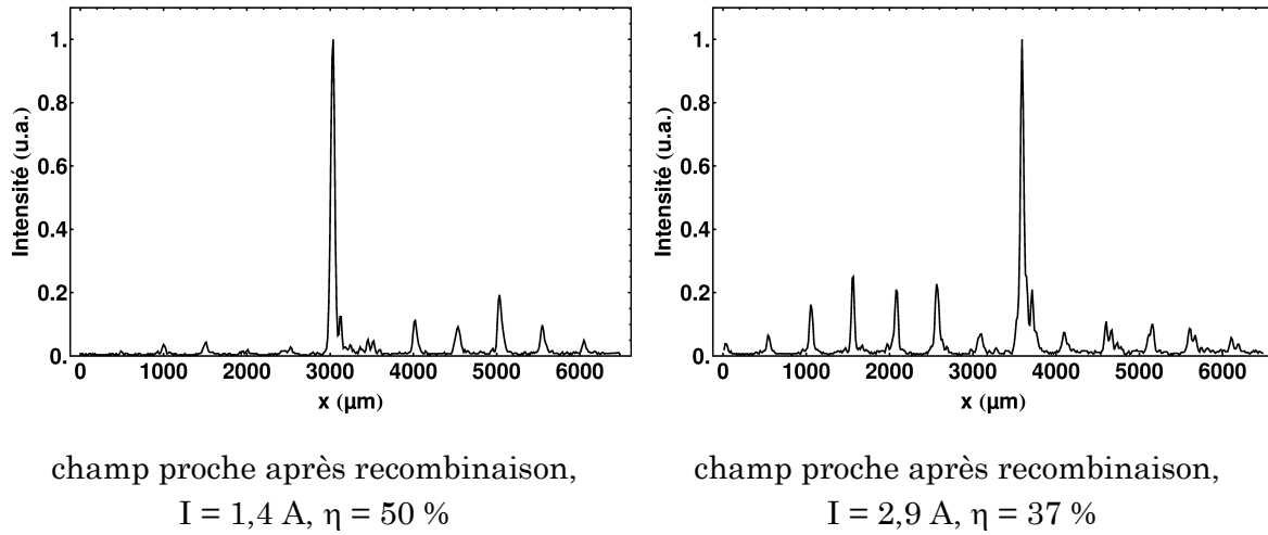
Figure IV-17 : Profils en champ proche après recombinaison, gauche : I = 1,4 \text{ A} , droite : I = 2,9 \text{ A} . 1
