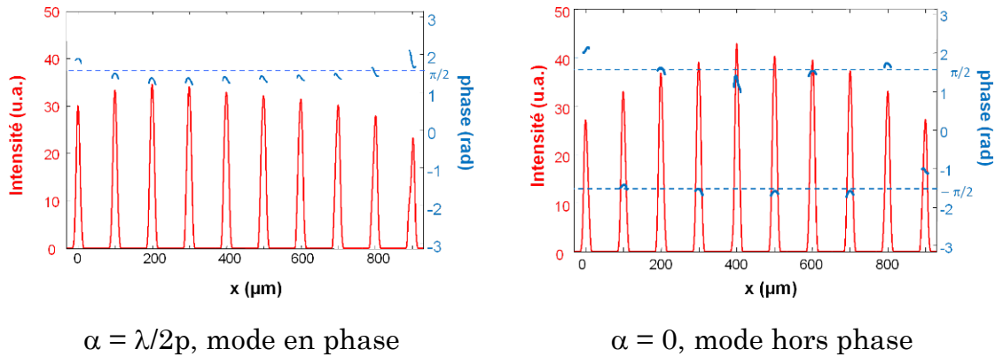
Figure II-24 : Profils en champ proche des modes hors phase et en phase – I = 3,9 \text{ A} ( = 3,2 \times I_{\text{seuil}} ), R = 40\% , 2L_{\text{ext}} = Z_T/2 .
