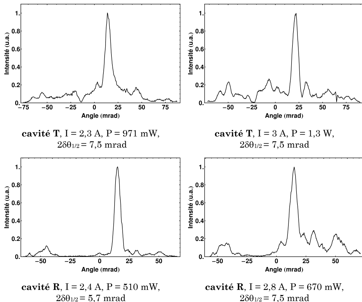
Figure III-28 : Profils en champ lointain en fonction du courant d'alimentation pour les deux cavités – haut : cavité T, bas : cavité R.
