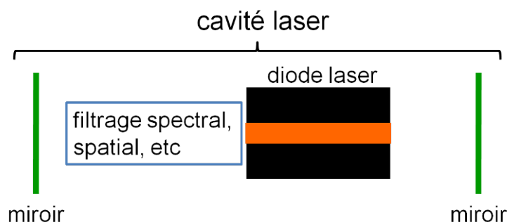
Figure I-10 : Schéma de principe d'une diode laser en cavité externe.
