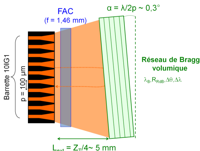
Figure III-10 : gauche – schéma de la cavité Talbot réalisée avec la barrette 10IG1 droite – photographie du prototype, FAC : lentille cylindrique de collimation de la direction verticale.
