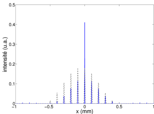
Figure IV-11 : Comparaison de la figure de diffraction du réseau de Damann (trait plein bleu) avec le profil en champ proche (pointillés gris) que l'on souhaite recombinaison.
