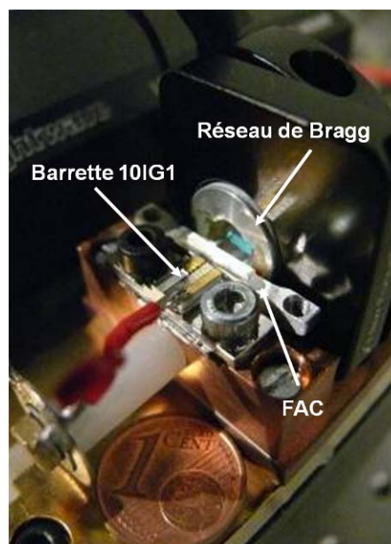
Figure III-10 : gauche – schéma de la cavité Talbot réalisée avec la barrette 10IG1 droite – photographie du prototype, FAC : lentille cylindrique de collimation de la direction verticale.
