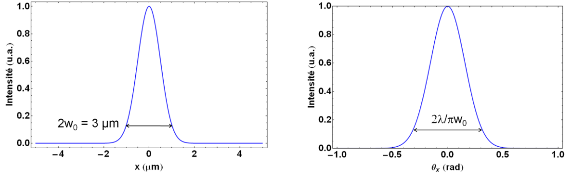
Figure I-1 : Champ proche (gauche) et champ lointain (droite) d'un faisceau gaussien – \lambda = 976 nm.
