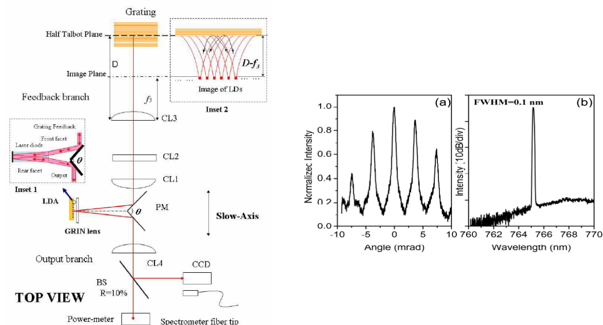
Figure I-37 – gauche : schéma expérimental de la cavité réalisée par [Liu 08] droite : Profil en champ lointain et spectre d'émission en fonctionnement cohérent – I = 50 A, P = 9 W.
