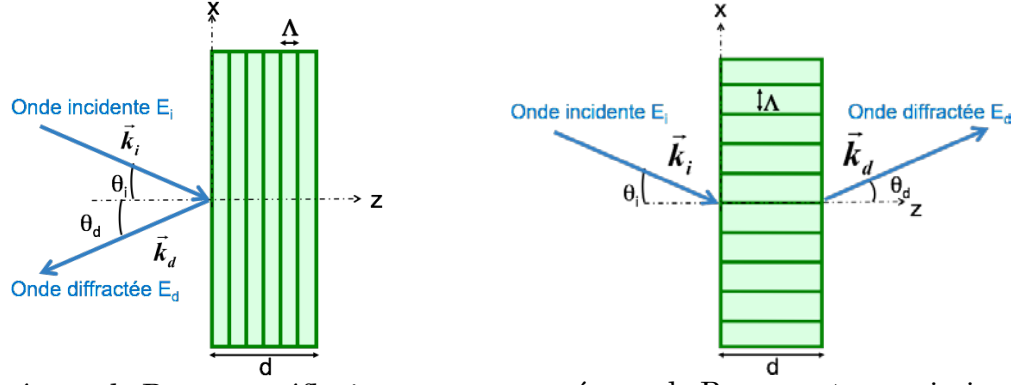
réseau de Bragg en réflexion réseau de Bragg en transmission Figure II-2 : Réseaux de Bragg volumiques considérés.
