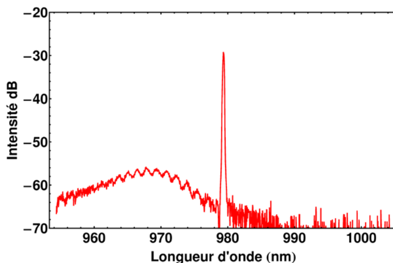
Figure III-30 : Spectre du laser en cavité R, I = 3A , P = 730 \text{ mW} , barrette 6IG1 adjacents II-1, résolution de l'analyseur de spectre 200 pm.
