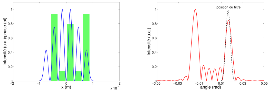
Figure II-22 : gauche – intensité (trait bleu) et phase normalisée à \pi (rectangle vert) du mode hors phase en champ proche. droite – champ lointain du mode hors phase et position du filtre – N = 6 émetteurs, 2w = 30 \mu\text{m} , p = 30 \mu\text{m} , \lambda = 976 \text{ nm} , \theta_0 = 16 \text{ mrad} , avec le réseau de Bragg en transmission défini dans le Tableau II-2.
