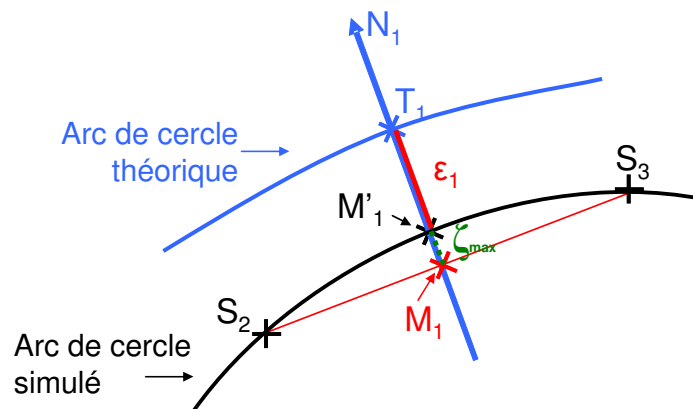
Figure II - 5 : Erreur \zeta due au palpé d'un arc de cercle simulé
