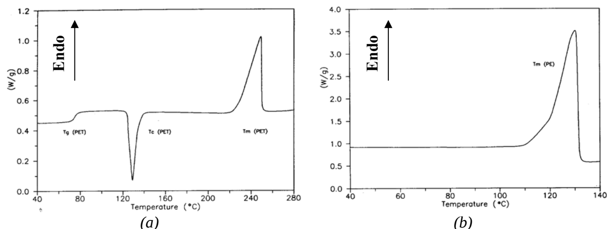
Figure 1 : Thermogrammes du PET (a) et du PEhd (b) purs : vitesse de chauffage 10°C/min
