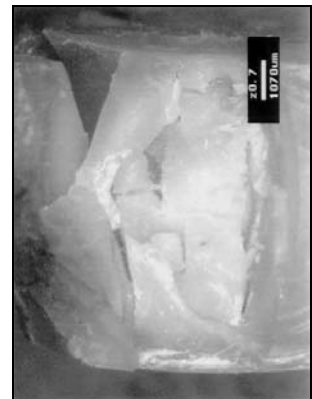
Figure 32 : Structure du type 4 : Schéma de l'échantillon après essai Photographie du plot. Destruction d'une partie du plot Effondrement dans le sens transversal
