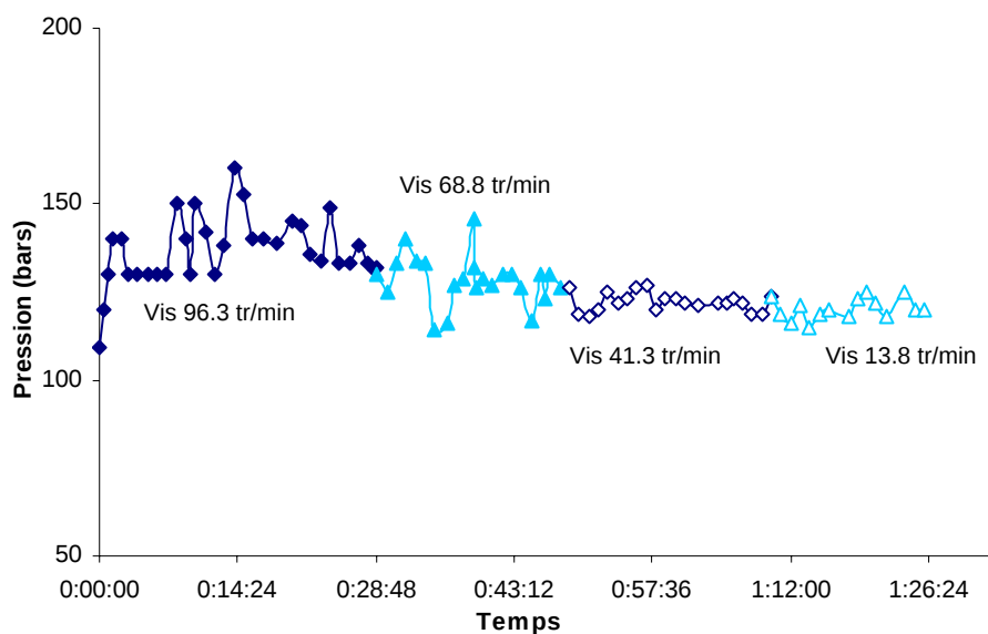
Figure 31 : Evolution de la pression en fonction du temps et de la vitesse de rotation Température de la filière froide : 90^{\circ}\text{C} Débit d'alimentation : 0.877 kg/h
