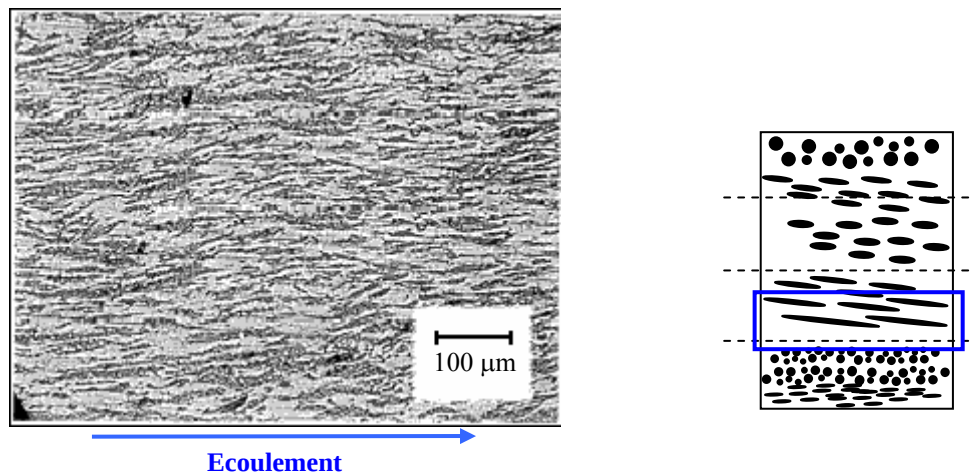
Figure 44 : Coupe longitudinale. Zone de transition (zone 2). Distribution de nodules
