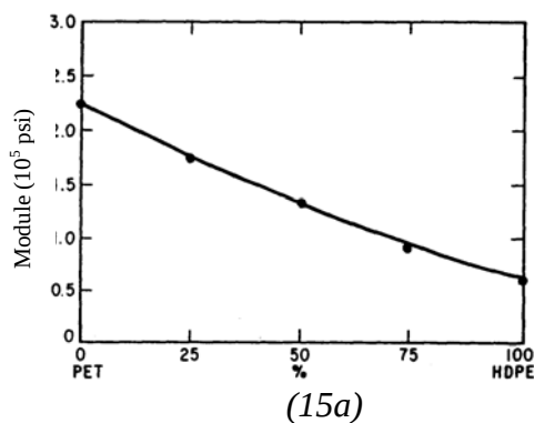
Figures 15 : Evolution du module d'élasticité (15a) et de la contrainte au seuil de plasticité (15b) en fonction de la proportion de PEhd pour des bandes 'longitudinales' de films extrudés.
