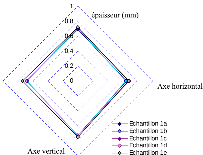
Figure 6 : Croix de répartition de l'épaisseur de matière 'plus amorphe' en mm suivant la coupe transversale pour 5 échantillons, cas du mélange 90/10
