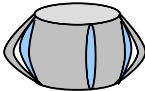
Figure 31 : Structure du type 3 . Schéma de l'échantillon après essai Photographie du plot. Décollement de la peau du plot dans le sens transversal Cœur du plot intact
