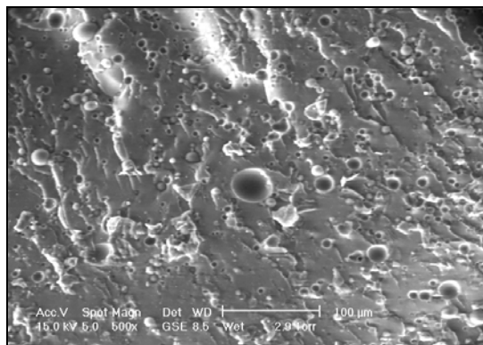
Figure 16 : Périphérie du jonc. Présence de vagues, de cavités et de nodules
