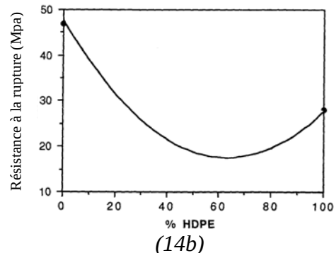
Figures 14 : Allongement (14a) et résistance à la rupture (14b) de mélanges PET/PEhd en fonction de la proportion de PEhd.
