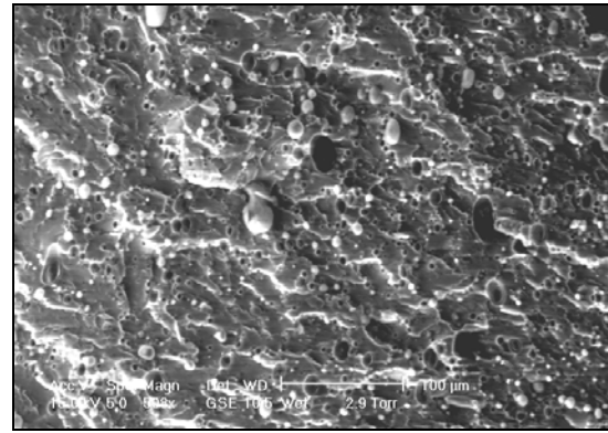
Figure 14 : Zone de transition. Symétrie autour de l'axe de la filière. Présence de gros et de petits nodules
