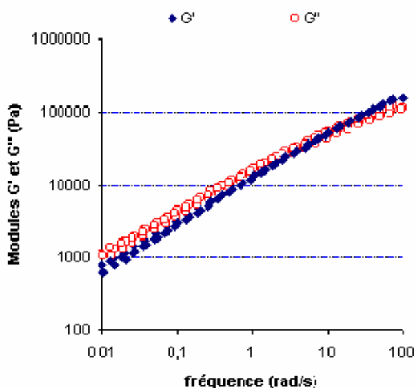
Figure 25 : Modules élastique et visqueux du PEhd dans le domaine 10^{-2} - 10^2 Hz Courbe maîtresse T_{\text{ref}} = 150^{\circ}\text{C}
