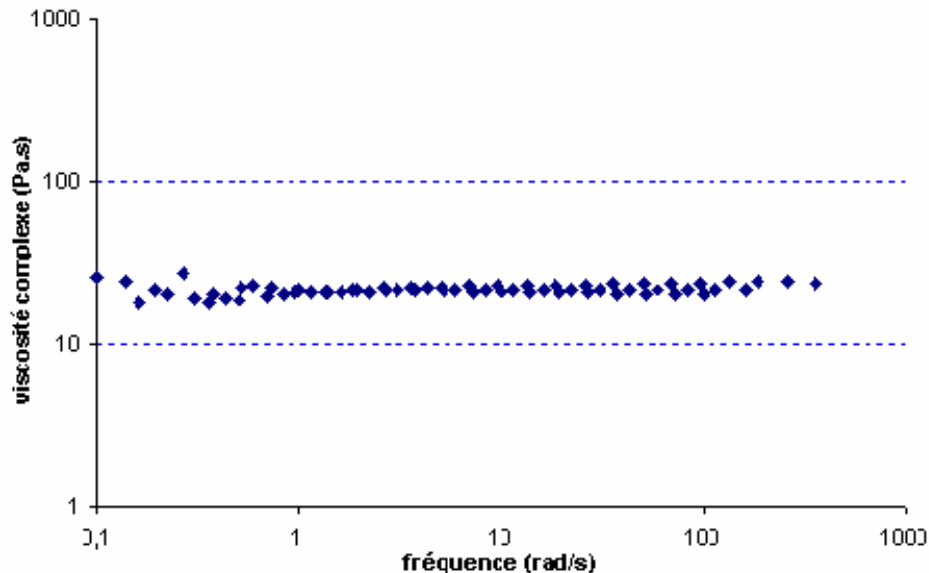
Figure 30 : Evolution de la viscosité du PET recyclé à différentes températures Courbe maîtresse T_{ref}=285^{\circ}\text{C}
