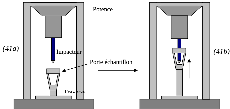
(41a) : Mise en place de l'échantillon et mise sous pression du vérin hydraulique (41b): Propulsion de la traverse et percussioin de l'échantillon par l'impacteur
