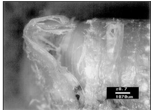
Figure 31 : Structure du type 3 . Schéma de l'échantillon après essai Photographie du plot. Décollement de la peau du plot dans le sens transversal Cœur du plot intact
