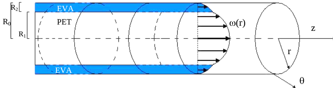
Figure 42: Configuration de l'écoulement bicouche annulaire
