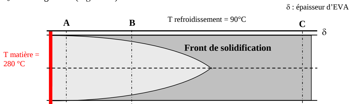
Figure 54 : Configuration de l'écoulement bicouche annulaire
