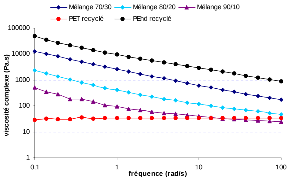
Figure 34 : Evolution de la viscosité complexe dans le domaine 10^{-1} - 10^2 rad/s pour différents mélanges à 275°C
