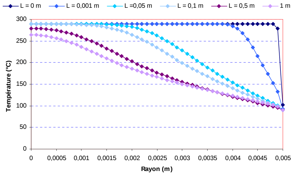
Figure 50 : Evolution du profil de température - Q_I = 1.235 \cdot 10^{-07} \text{ m}^3/\text{s}
