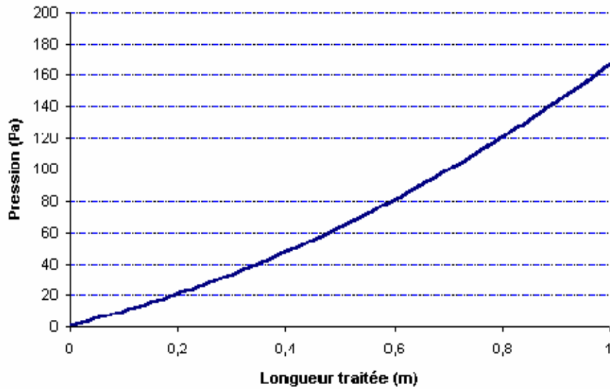
Figure 49 : Evolution du gradient de pression - Q_I = 1.235 \cdot 10^{-07} \text{ m}^3/\text{s}
