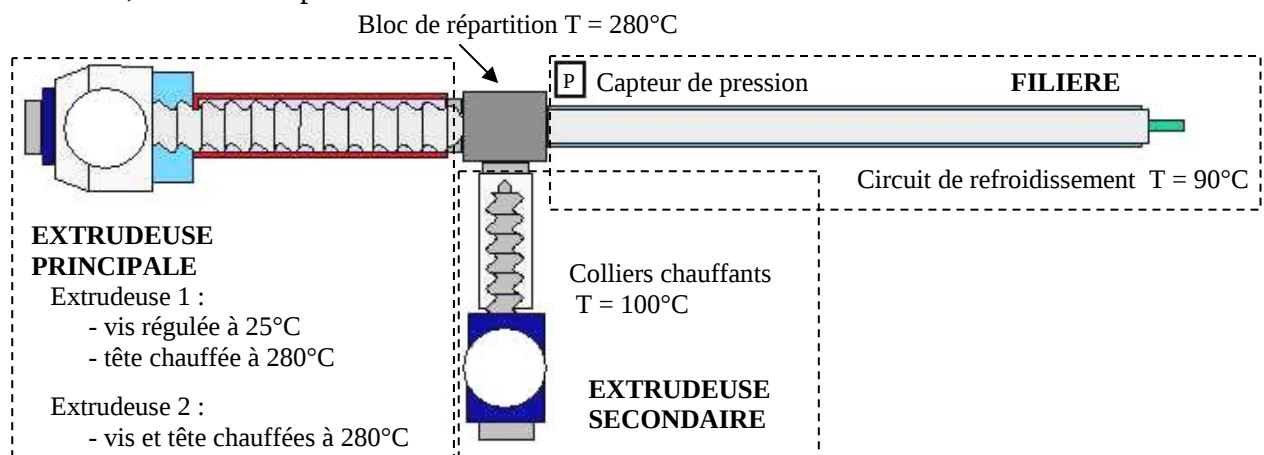
Figure 3 : Schéma de la machine SCAMIA
