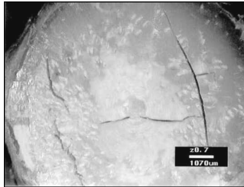
Figure 30 : Structure du type 2 : Schéma de l'échantillon après essai Photographie du plot. Fissures apparentes sur la surface de base et sur la surface latérale
