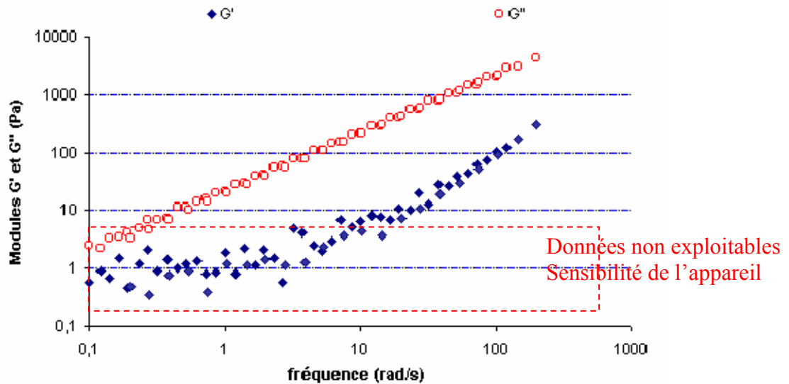
Figure 29 : Module élastique et visqueux du PET dans le domaine 10^{-2} - 10^3 Hz Courbe maîtresse T_{ref}=285^{\circ}\text{C}
