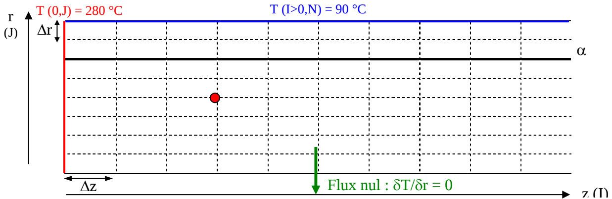
Figure 45 : Représentation du maillage nécessaire à la méthode des différences finies. Conditions aux limites
