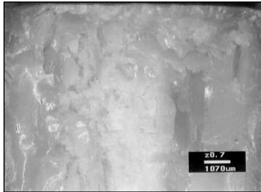
Figure 33 : Structure du type 5 : Schéma de l'échantillon après essai Photographie du plot. Surface de base du plot intacte. Eclatement 'extérieur' du plot. Apparition du coeur
