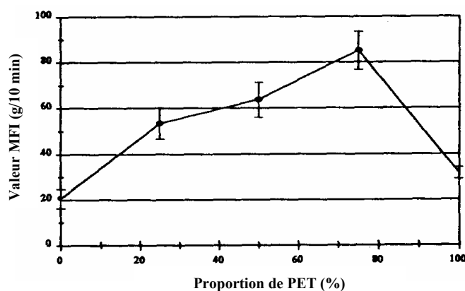
Figure 24 : Evolution de l'indice de fluidité à chaud d'un mélange PET/PEhd en fonction de la proportion de PET.
