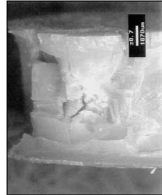
Figure 33 : Structure du type 5 : Schéma de l'échantillon après essai Photographie du plot. Surface de base du plot intacte. Eclatement 'extérieur' du plot. Apparition du coeur
