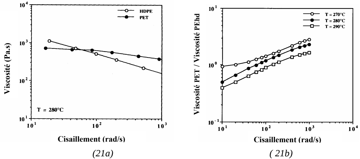
Figure 21 : Evolution de la viscosité du PET et du PEhd en fonction du taux de cisaillement à 280^\circ\text{C} (21a)
