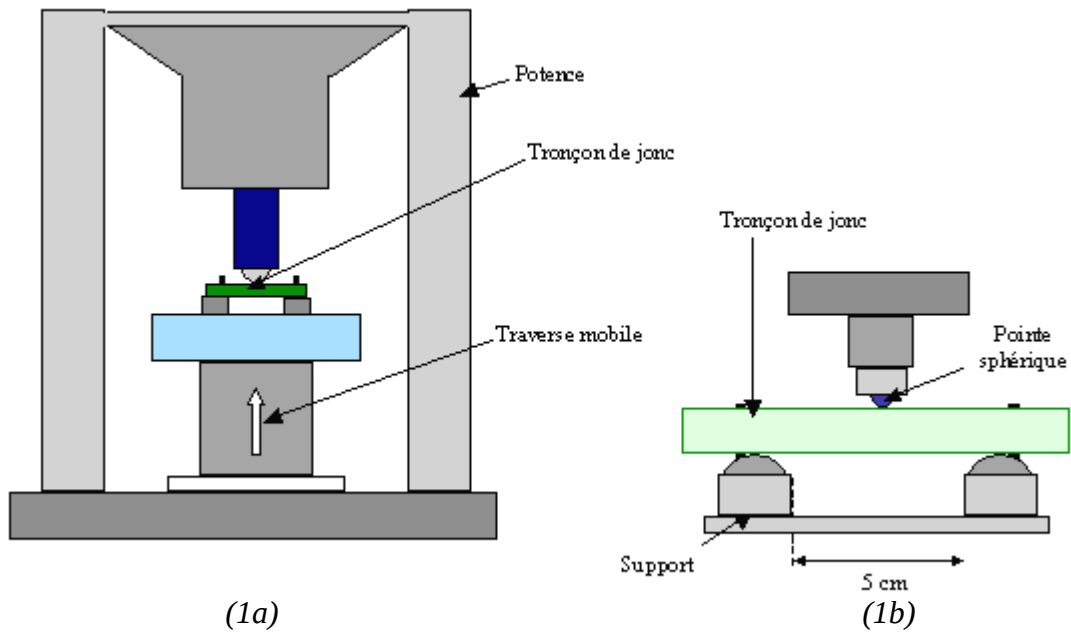
Figures 1 : Schéma de la machine DARTECH (1a) Détail de la machine - Essai de flexion 3 points (1b)
