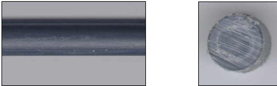
Figure 29 : Jonc de mélange 70/30 pour une vitesse de rotation de 78 tr/min
