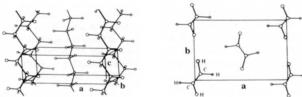
Figure 11 : la structure orthorhombique des polyéthylènes [19]
