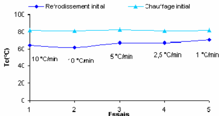
Figure 18 : Températures de fusion et de cristallisation de l'EVA grade 150
