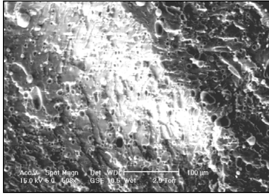
Figure 14 : Zone de transition. Symétrie autour de l'axe de la filière. Présence de gros et de petits nodules
