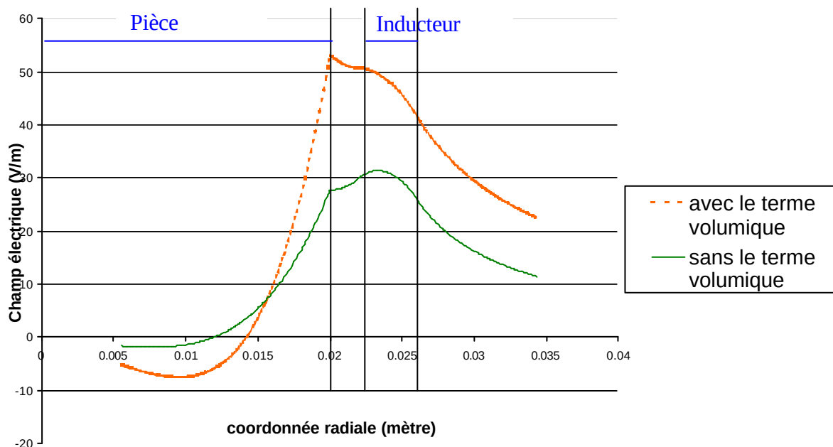
Figure 40 : Profils radiaux de champ électrique calculés à partir de modèles considérant le terme volumique supplémentaire ou non
