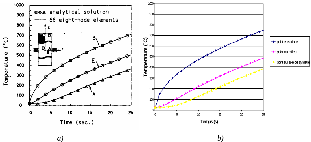
Figure 44 : Evolution temporelle de la température en surface de la pièce, sur l'axe de symétrie et entre les deux. a) solution analytique tirée de l'article de Wang [55] ; b) solution numérique
