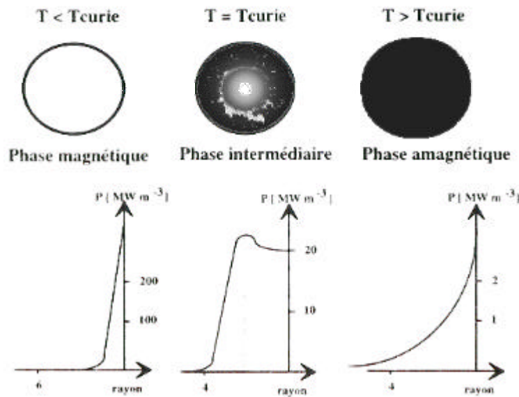
Figure 4 : Evolution de la distribution de puissance électromagnétique avec la température au passage de la température de Curie pour une billette d'acier de diamètre 120mm et une fréquence d'alimentation de 300Hz.
