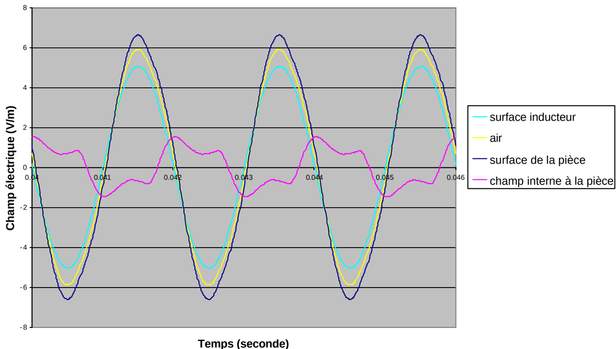
Figure 38 : Evolution temporelle du champ électrique en différents points du domaine pour une fréquence de 500Hz, un pas de temps dt=T/128 , avec la période T=0.002s .
