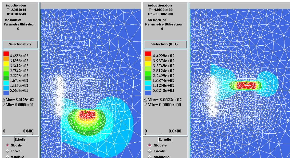
Figure 47 : Iso valeurs du champ électrique effectif pour deux positions de l'inducteur.
