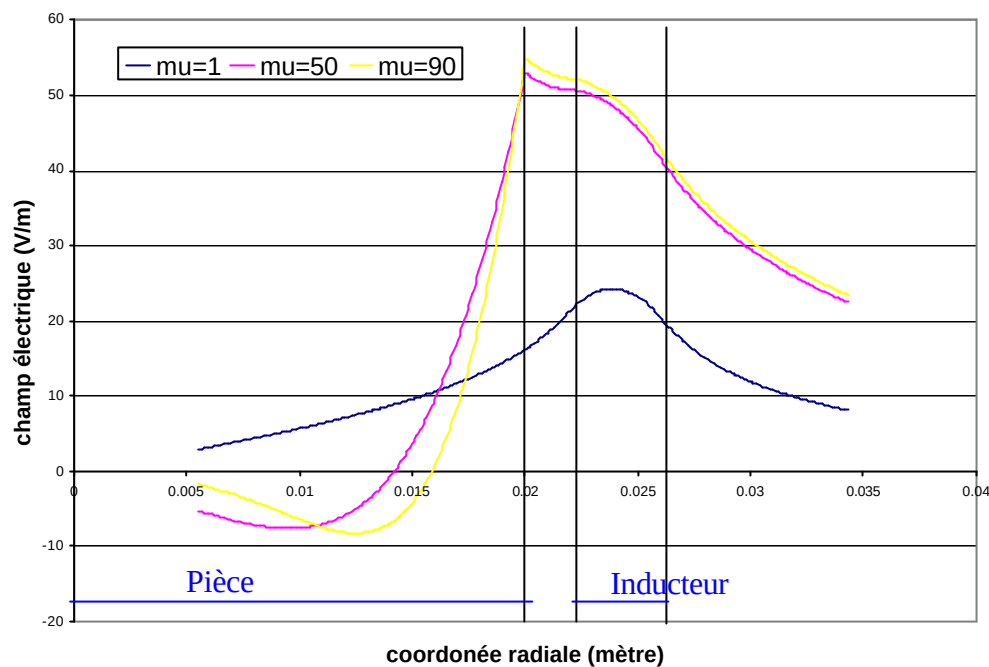
Figure 42 : Variation du profil du champ électrique calculé avec le modèle complet pour différentes perméabilités magnétiques relatives
