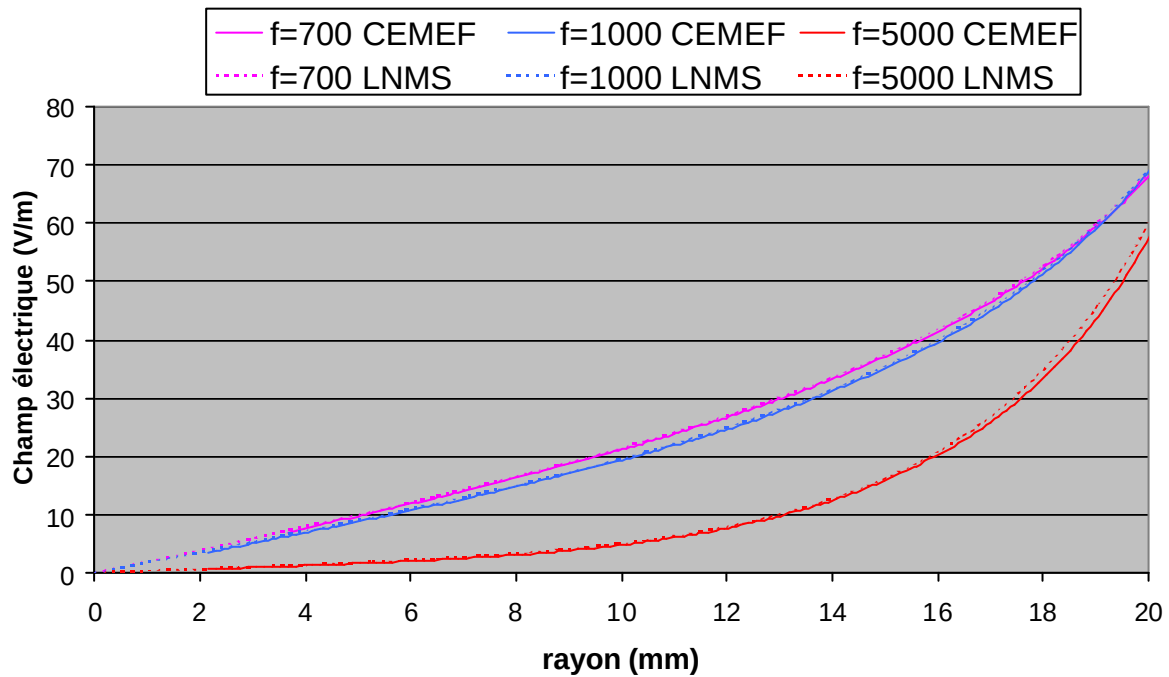
Figure 43 : Comparaison des profils du champ électrique effectif (code du Cemef) et de la norme du champ électrique complexe (code de LNMS). Les profils sont tracés dans la pièce de rayon 20mm.
