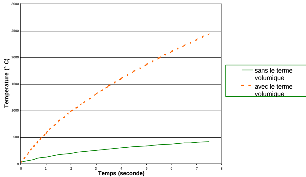
Figure 41 : Evolutions de la température en surface de la pièce calculées à partir de modèles considérant le terme volumique supplémentaire ou non
