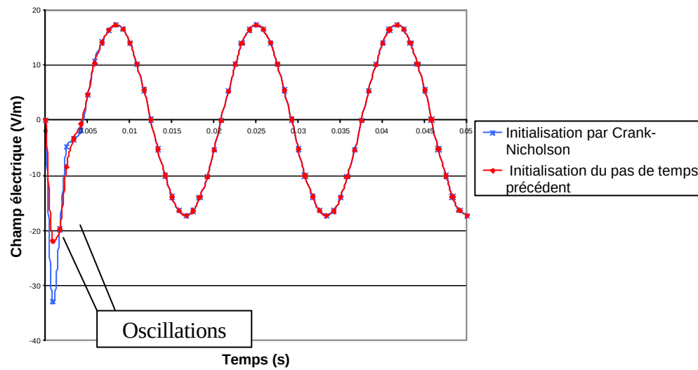
Figure 35: Evolutions temporelles du champ électrique calculées pour deux initialisations différentes du schéma d'intégration de Dupont.
