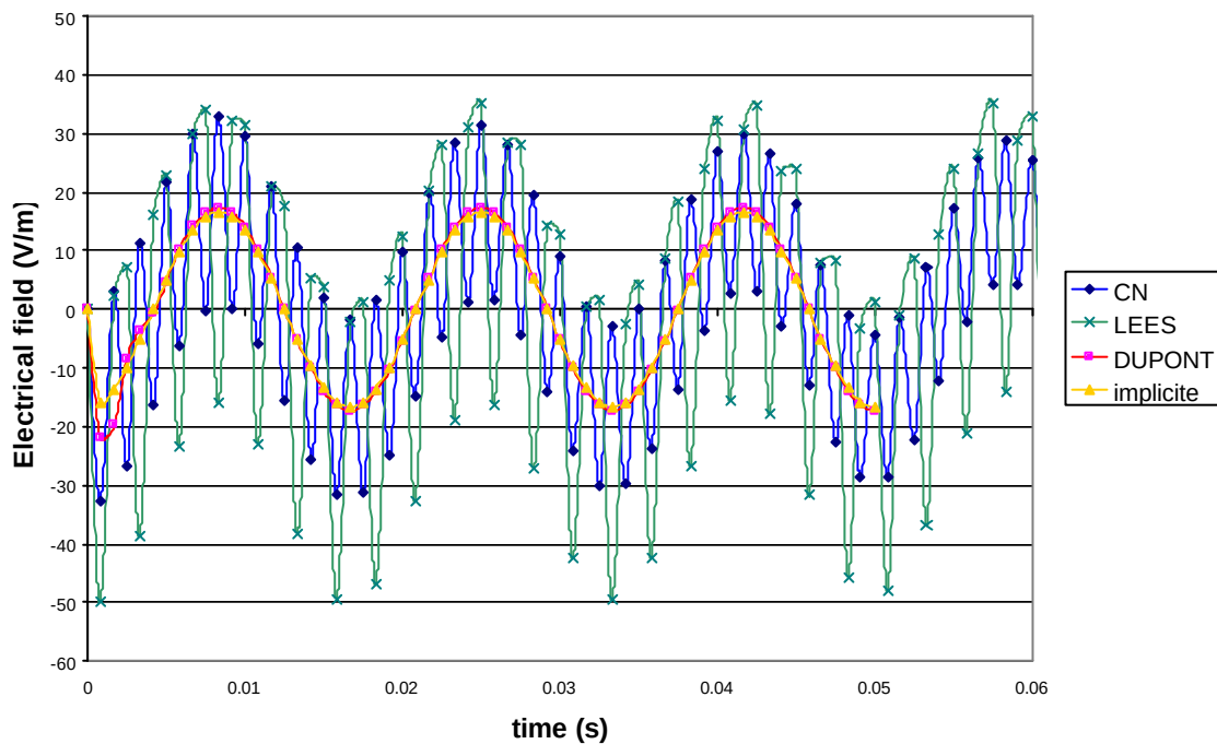
Figure 33 : Evolution temporelle du champ électrique en un point de la surface de la pièce.
