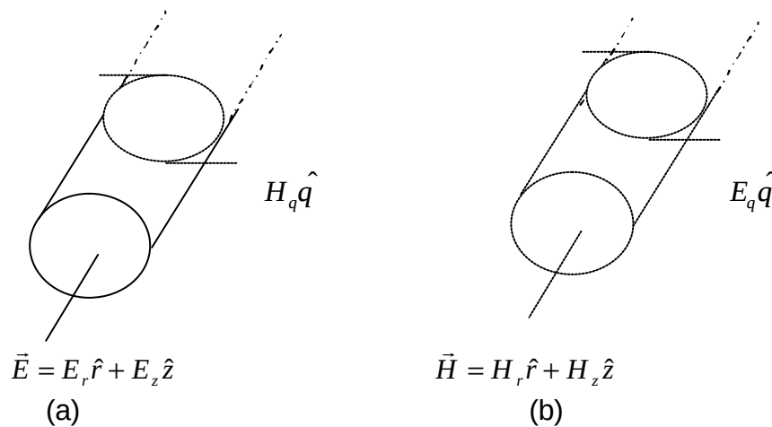
Figure 5 : Représentations des modes TE (a) et TM (b) pour une symétrie axiale.
