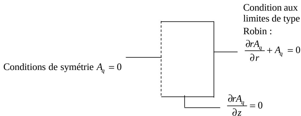
Figure 8 : Conditions aux limites de notre modèle
