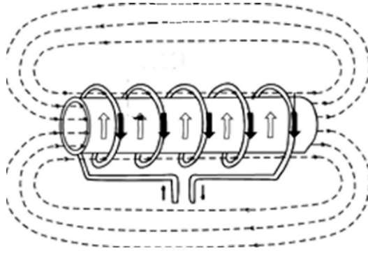
Figure 1 : Principe du chauffage par induction
