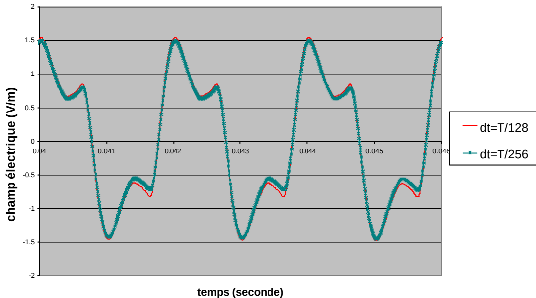
Figure 39 : Modification du profil électrique avec le pas de temps à l'intérieur de la pièce
