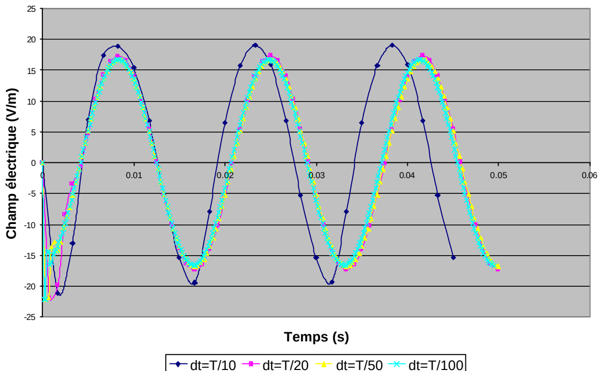
Figure 37: Evolution temporelle du champ électrique en un point de la surface de la pièce pour différents pas de temps électromagnétique, T étant la période du signal électrique.
