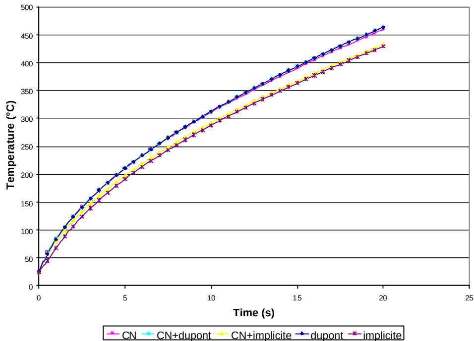
Figure 36 : Evolution temporelle de la température en surface de la pièce pour différents schémas d'intégration en temps
