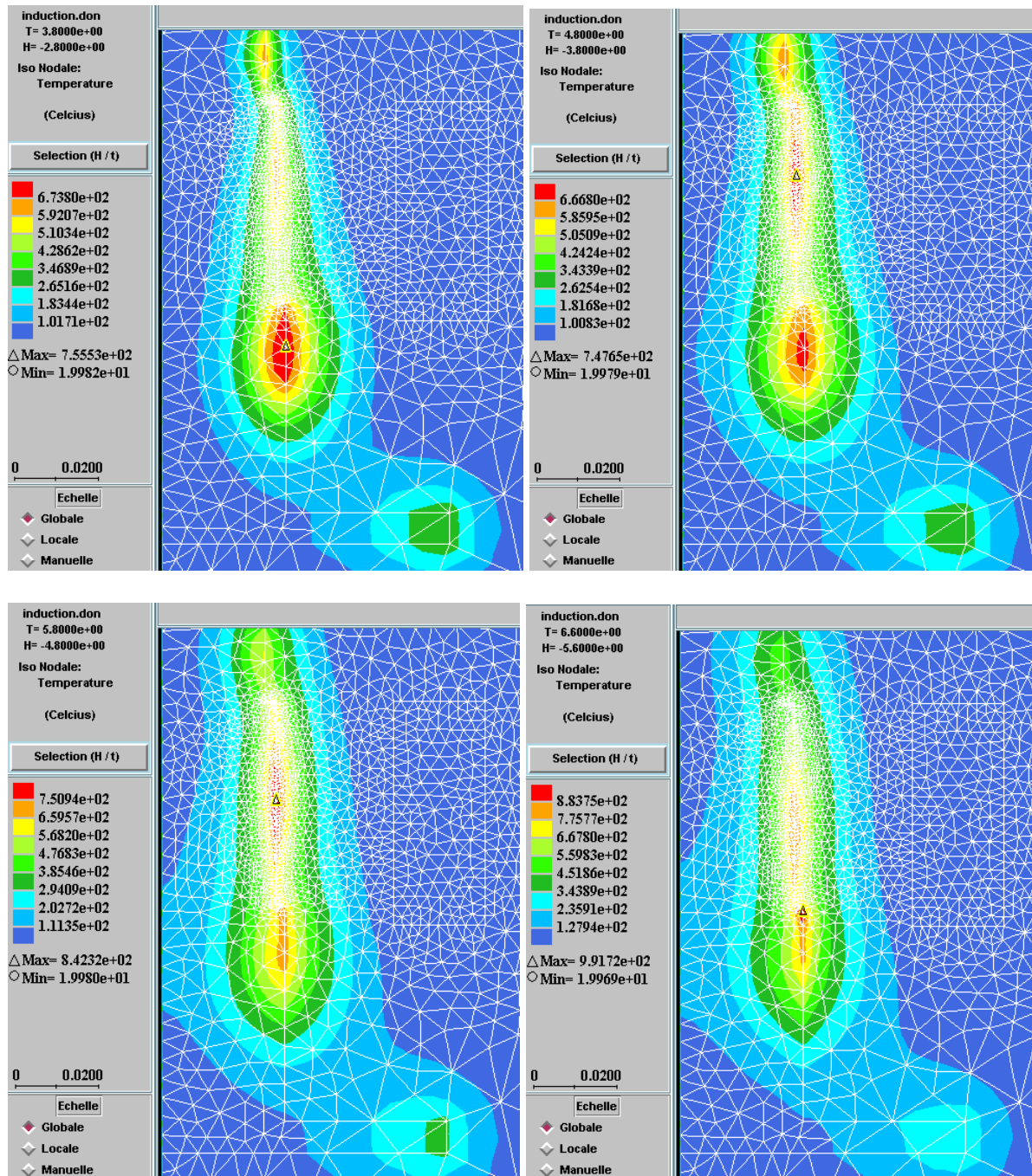
Figure 48 : Iso-valeurs des températures au cours du temps.
