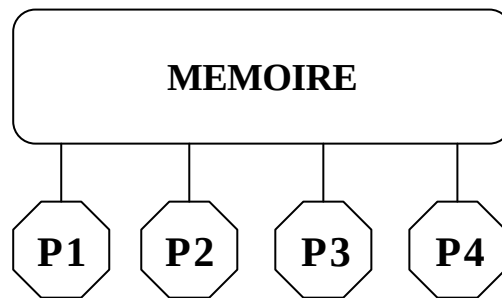
Figure 49 : Architecture à mémoire partagée sur un ordinateur à quatre processeurs
