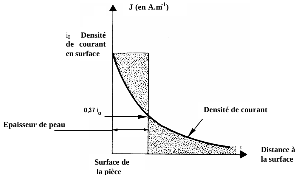
Figure 2 : Représentation de la profondeur de peau
