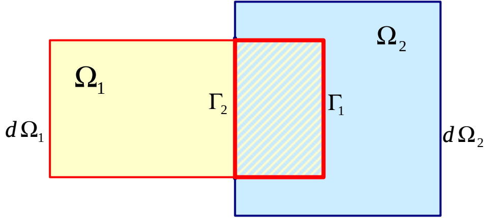
Figure 52 : Décomposition du domaine W en deux sous-domaines avec recouvrement
