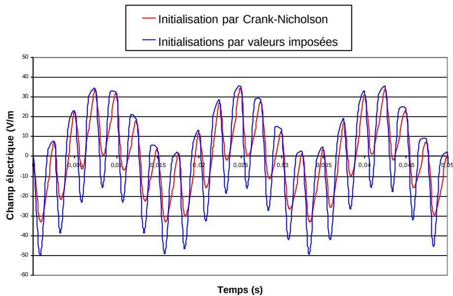
Figure 34: Evolutions temporelles du champ électrique calculées pour deux initialisations différentes du schéma d'intégration de Lees.
