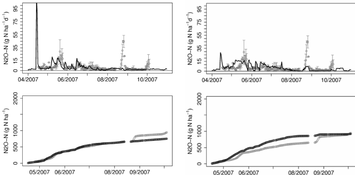
Figure A8-1: CERES-NOE (best set of parameter values)
