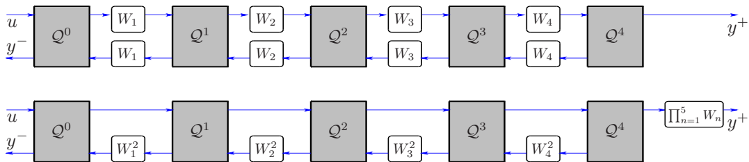
Fig. 1.11 – Factorisation des propagateurs sur la ligne inférieure. Cette réécriture du réseau permet de réduire le nombre de propagateurs et donc de diminuer la complexité de calcul.
