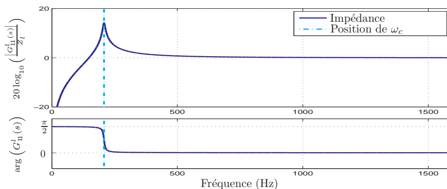
Fig. 2.10 – Impédance d'un tube semi-infini, G_{11}^l(s = 2i\pi f) pour r_l = 5 mm, \Upsilon = 15 m -2 , \varepsilon = 0.0525 m -1/2 , \zeta_l = 0 m -1 .
