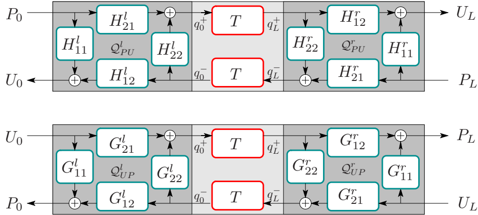
Fig. 2.9 – Décomposition des quadripôles \mathbf{Q}_{PU} and \mathbf{Q}_{UP} .
