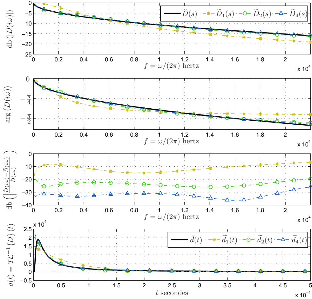
Fig. 1.15 – Résultats de l'optimisation de la fonction \tilde{D} par des fonctions de transfert de dimension finie : \tilde{D}_n est l'approximation de \tilde{D} avec n pôles. Ici \epsilon = 7.10^{-3} \text{ s}^{\frac{1}{2}} , \omega_- = 1 \text{ Hz} et \omega_+ = 22 \text{ kHz} .
