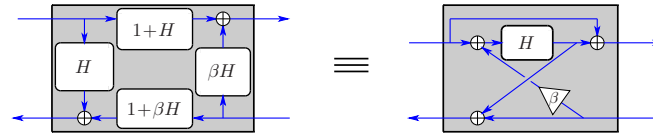
Fig. 1.10 – Factorisation de la fonction de réflexion d'une cellule de Kelly-Lochbaum. Pour les jonctions de cylindres : \beta = -1 et H(s) = k , et pour les jonctions de cônes : \beta = 1 et H(s) = R_s(s) . Alors que la structure originale fait apparaître 4 réflexions H , la forme factorisée fait apparaître une seule fonction H . Ceci a pour intérêt de diminuer la complexité de calcul.
