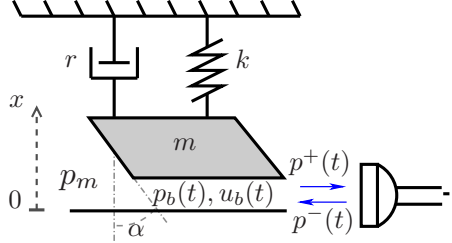
Fig. 1.8 – Schéma du modèle de lèvres
