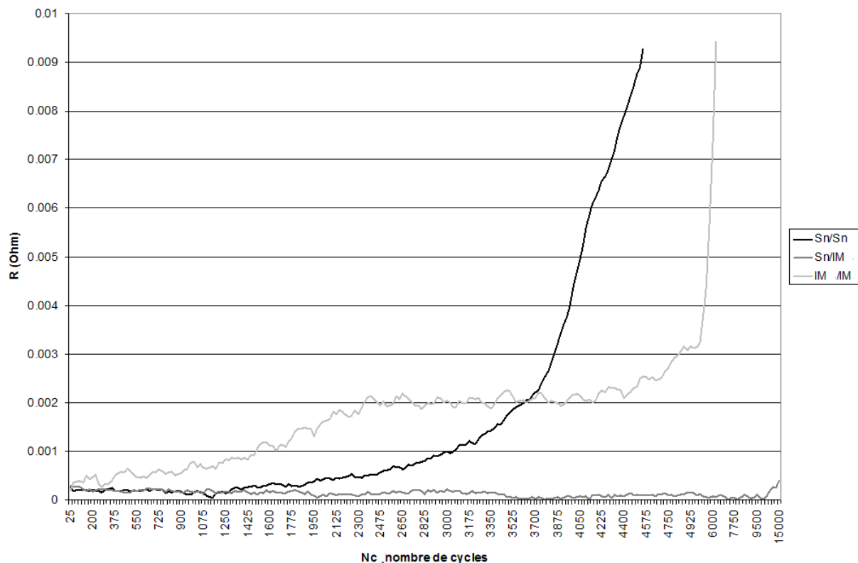
Figure 4.17 : Evolution de la résistance de contact en fonction du nombre de cycles pour les trois couples de matériaux, à 20°C et avec un débattement de 6 µm.
