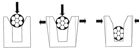
Figure 1.9 : Réalisation d'un déplacement d'isolant [1.9]
