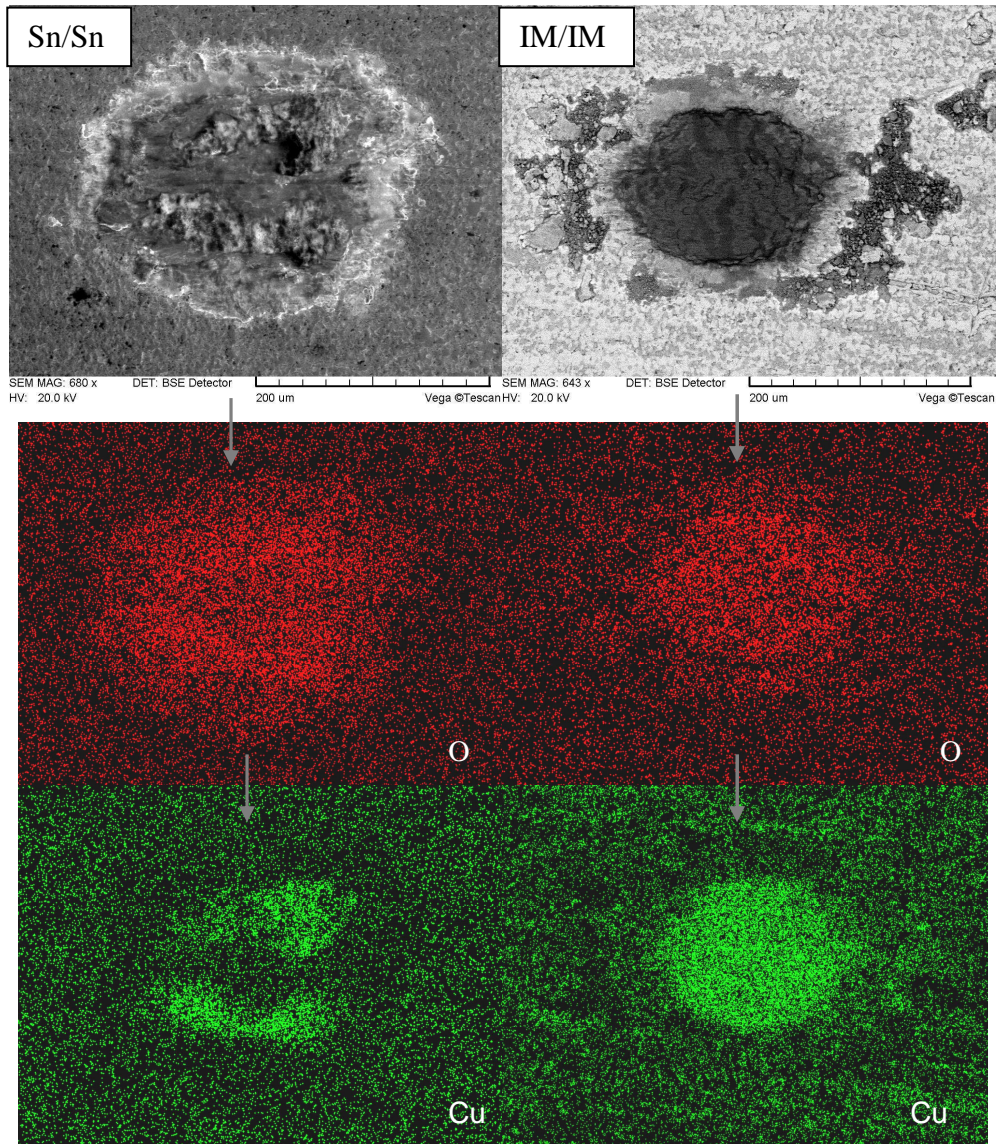
Figure 4.35 : Comparaison des traces pour le test interrompu : T= ambiante, HR = 10%, F=10Hz, \delta=6 \mu\text{m} , 15 000 cycles. A gauche image MEB en électrons rétrodiffusés puis cartographie de l'oxygène et du cuivre pour le couple Sn/Sn, à droite, couple IM/IM. Le substrat de cuivre est atteint pour les deux couples dans ces conditions
