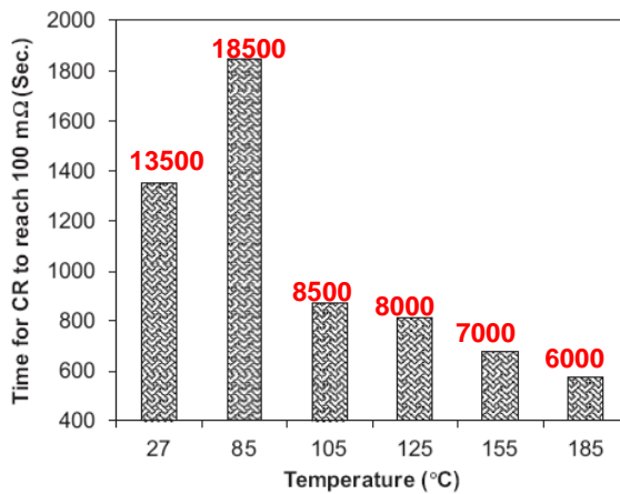
Figure 2.24 : Nombre de cycles pour atteindre le seuil de 100 mOhm à différentes températures. Les autres paramètres fixés sont : amplitude + ou - 90 µm, fréquence 10 Hz, charge normale 0,5 N, humidité relative 55% et courant imposé 0,5 A. Le nombre de cycles correspondant est indiqué en rouge [2.32]
