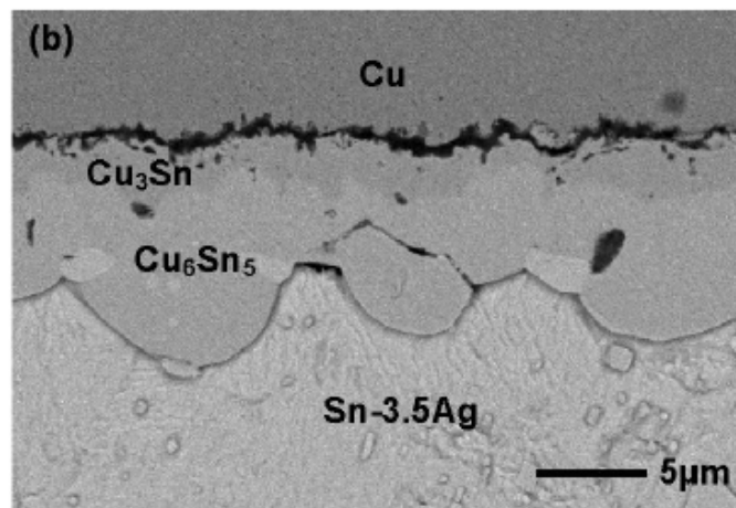
Figure 2.7 : Formation de pores à l'interface Cu/ \text{Cu}_3\text{Sn} suite à un traitement thermique de 480h à 150°C. On remarque que les interfaces ne sont pas rigoureusement planes, ceci étant certainement dû à l'effet de joints de grain et de précipités [2.17]
