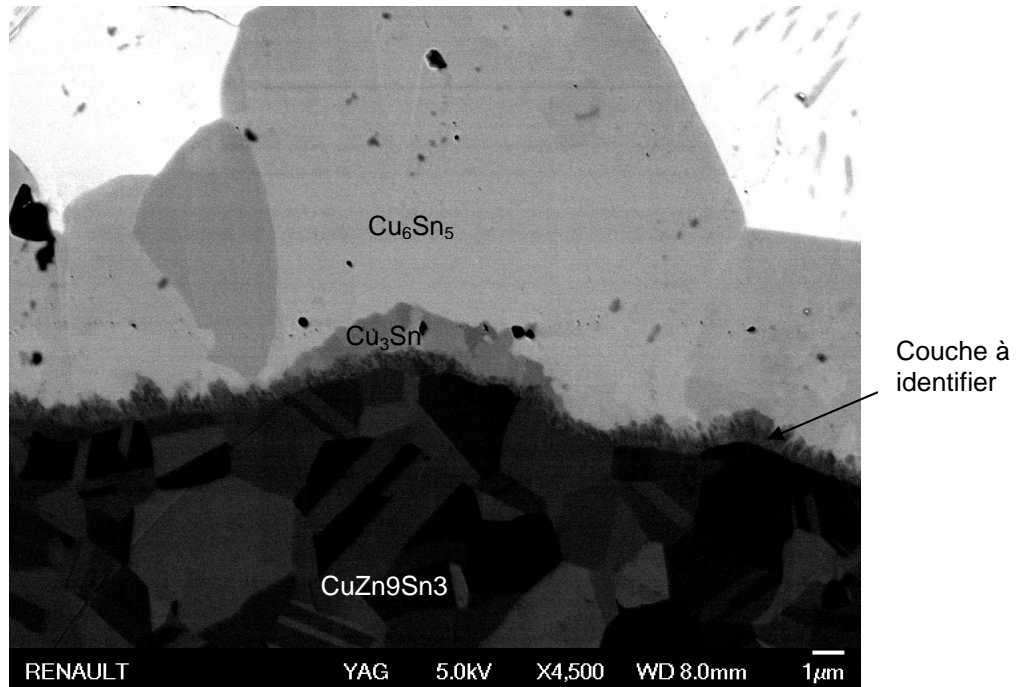
Figure 3.36 : Image MEB en électrons rétrodiffusés après polissage ionique d'un étain mat de 18 µm sur CuZn9Sn3 vieilli 1000h à 150°C
