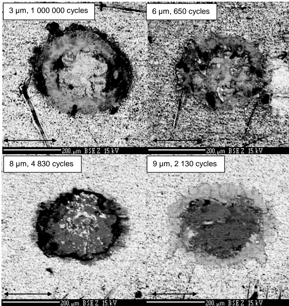
Figure 4.30 : Traces de fretting observées en fin de vie sur le couple IM/IM à 100^{\circ}\text{C} pour divers débattements
