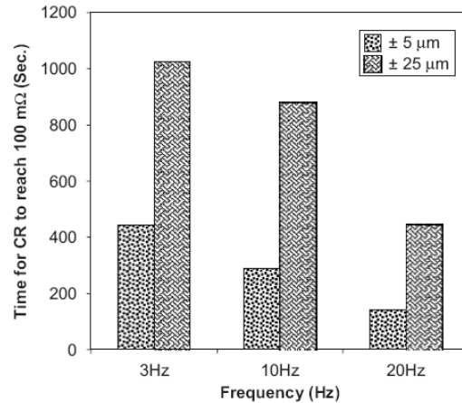
Figure 2.21 : Durée nécessaire pour atteindre la valeur de 100 mOhm pour la résistance de contact. La température est fixée à l'ambiante, l'humidité relative à 55%, la charge normale à 0,5N et le courant à 0,1A. Deux débattements sont comparés, \pm 5 et 25 \mu\text{m} [2.32]
