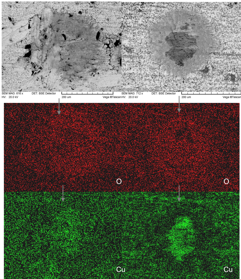
Figure 4.36 : Comparaison des traces pour le test interrompu : T= 100^{\circ}\text{C} , HR = 10\% , F=10\text{Hz} , \delta=6\ \mu\text{m} , 2 000 cycles. A gauche image MEB en électrons rétrodiffusés puis cartographie de l'oxygène et du cuivre pour le couple Sn/Sn, à droite, couple IM/IM
