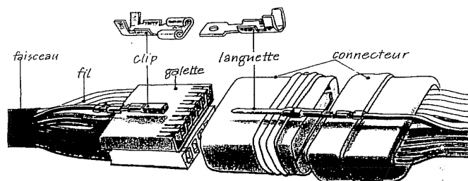
Figure 1.1 : Connecteur automobile
