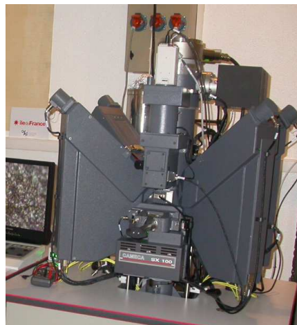
Figure 3.15 : Microsonde de Castaing SX100 utilisée pour les observations en coupe (profils et cartographies)
