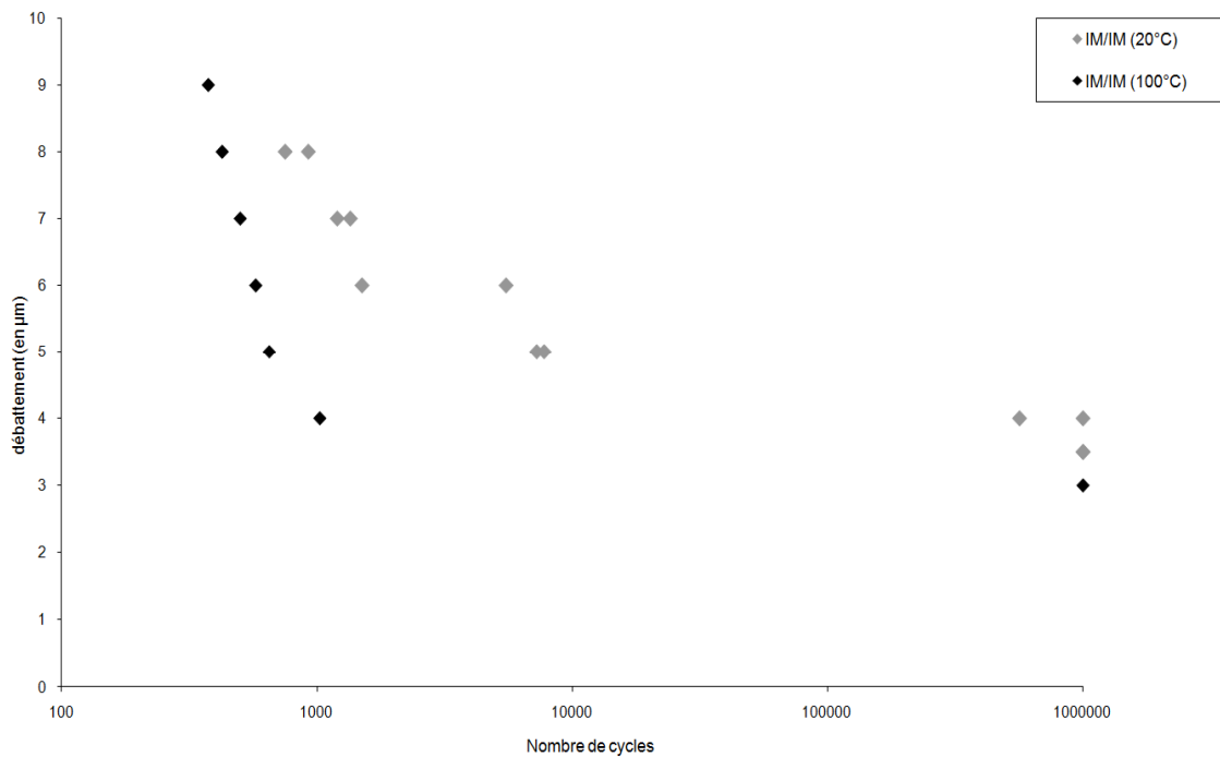
Figure 4.22 : Durée de vie du couple IM/IM à 20 et 100°C. La durée de vie à 100°C est également dégradée
