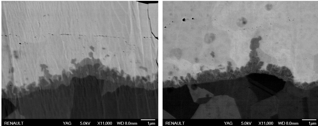
Figure 3.38 : Images MEB en électrons rétrodiffusés à fort grossissement après polissage ionique d'un étain mat de 18 \mu\text{m} sur substrat riche en zinc (laiton à gauche et chrysocale à droite) vieilli 1000h à 150°C
