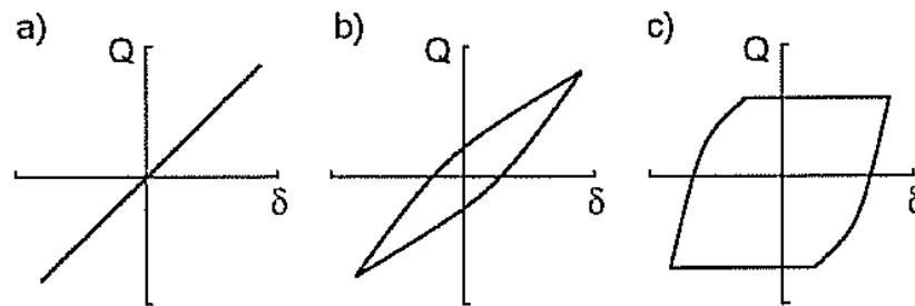
Figure 2.12 : Différents régimes de fretting [2.30]
