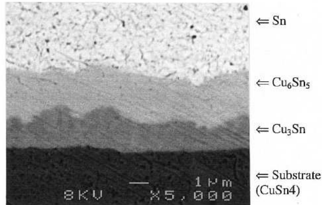
Figure 2.3 : Observation au MEB en coupe transverse, montrant l'arrangement multicouche Cu/Cu 3 Sn/Cu 6 Sn 5 /Sn (traitement de 32h à 173°C) [2.11]
