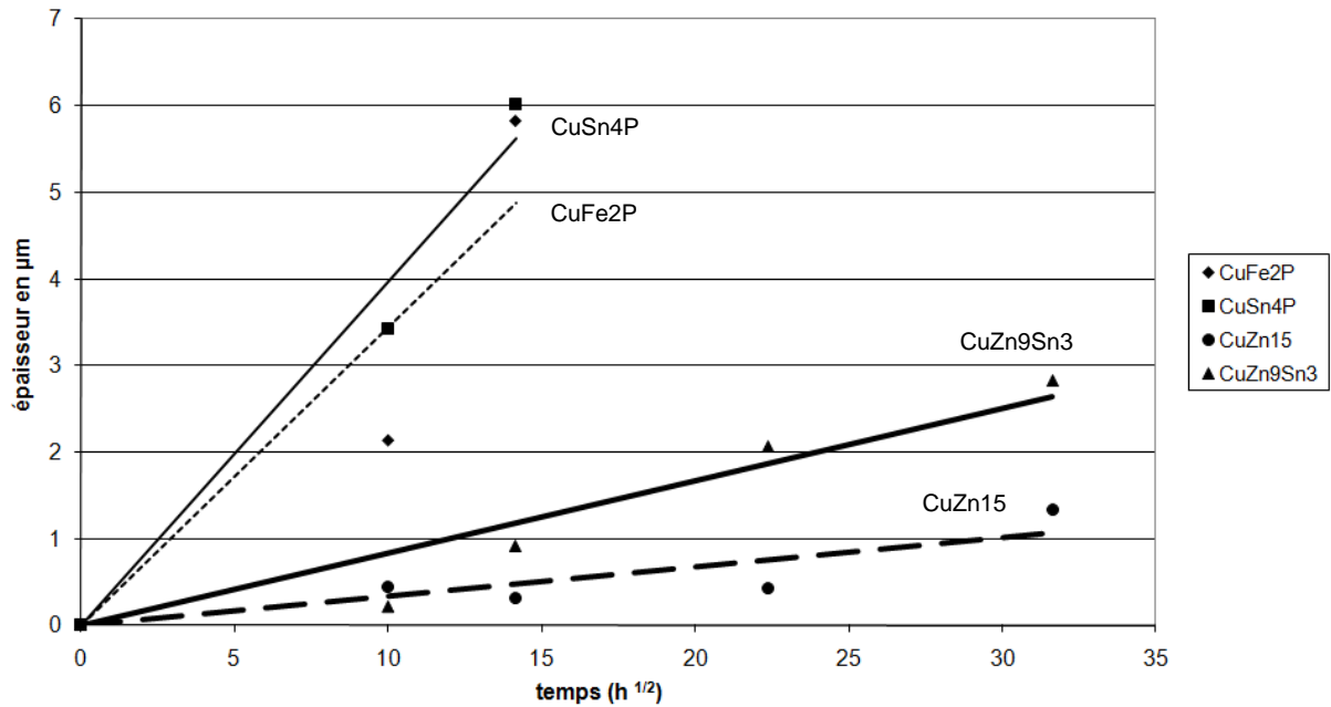
Figure 3.32 : épaisseur d'intermétallique Cu 3 Sn formé à 150°C pour chaque substrat
