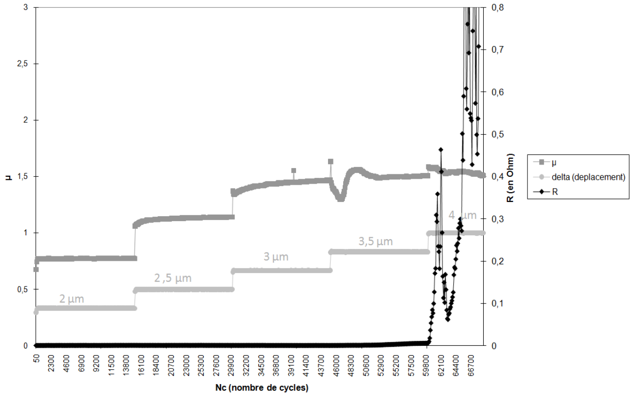
Figure 4.10 : Résultats en débattement variable pour le couple Sn/IM à 20°C
