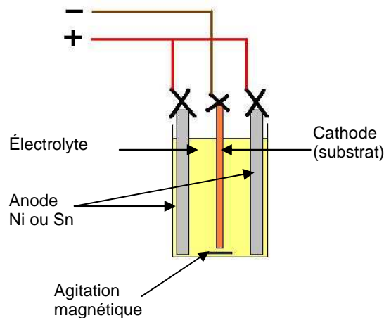
Figure 3.2 : Installation de laboratoire pour réaliser les dépôts électrolytiques de cette étude
