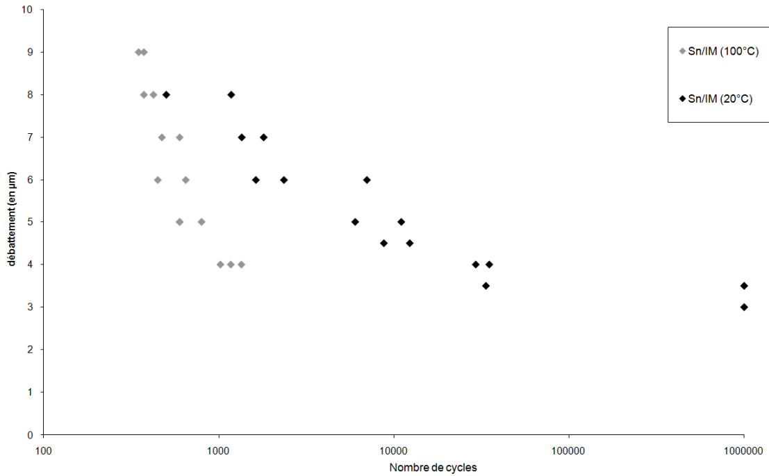
Figure 4.21 : Durée de vie du couple Sn/IM à 20 et 100°C. La durée de vie à 100°C est fortement dégradée par l'élévation de température
