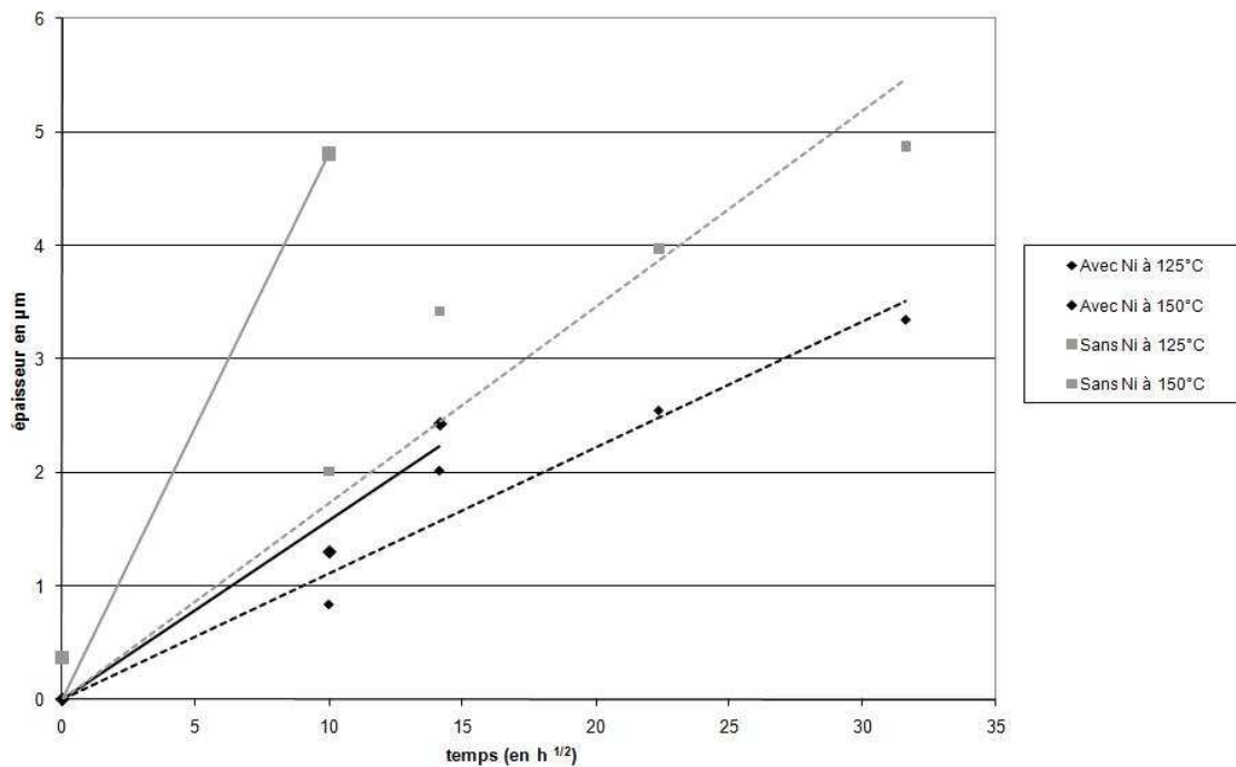
Figure 3.45 : épaisseur totale d'intermétallique formé avec et sans sous-couche nickel
