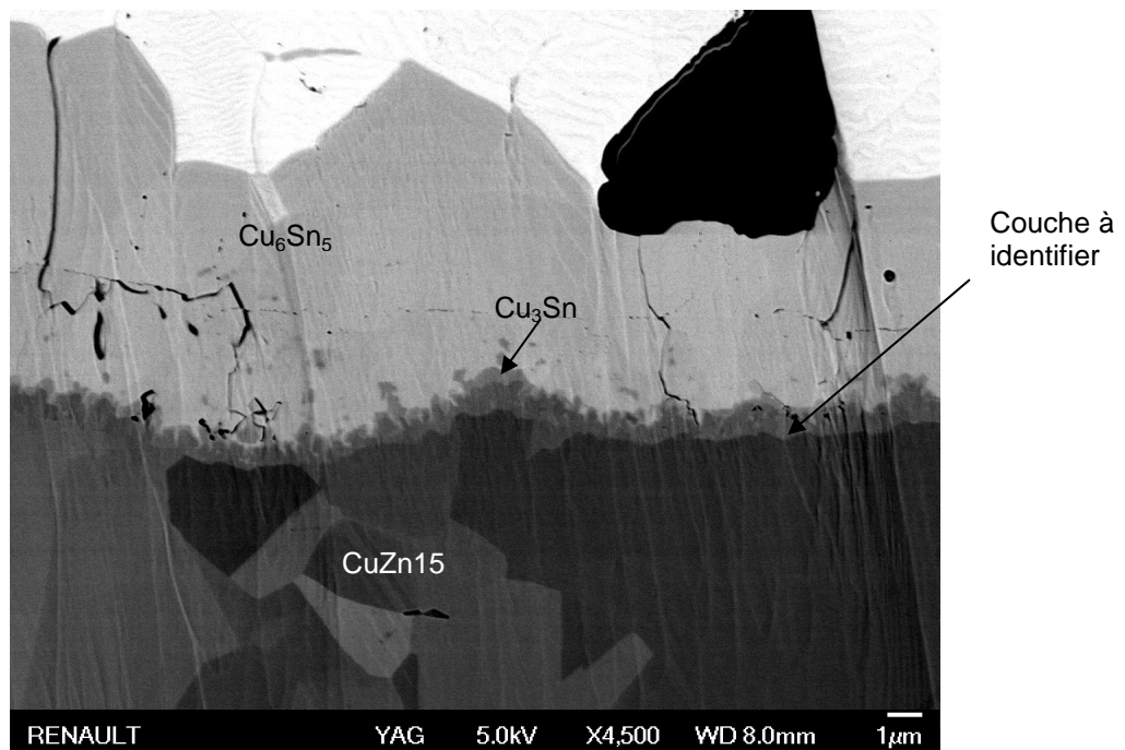
Figure 3.37 : Image MEB en électrons rétrodiffusés après polissage ionique d'un étain mat de 18 µm sur CuZn15 vieilli 1000h à 150°C
