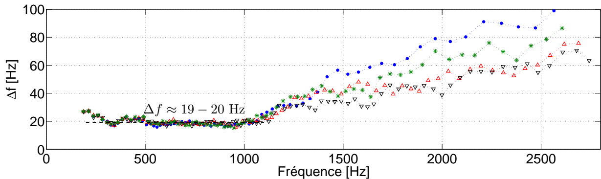
FIG. 3.25 – Espacement intermodal moyen \Delta f [Hz] de la table d’harmonie estimé aux quatre points \mathbf{A}_1 ( \bullet ), \mathbf{A}_2 ( \triangle ), \mathbf{A}_3 ( \nabla ), \mathbf{A}_5 ( * ) en fonction de la fréquence. Il est calculé par moyenne glissante sur 6 espacements intermodaux successifs. Les pointillés ( \cdots ) entre chacune des estimations sont rajoutés pour guider la lecture. Le plateau ( -- ) observé entre 500 et 1000 Hz confirme que la table se comporte dans ce domaine fréquentiel comme une plaque homogène.
