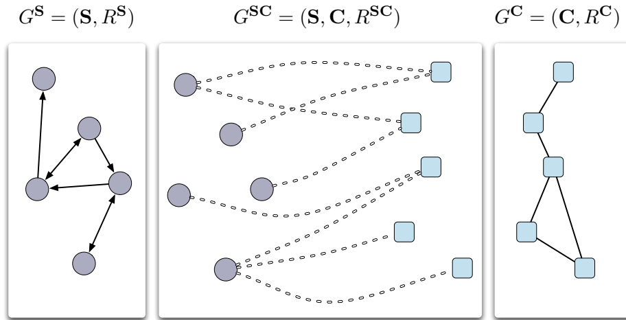
FIGURE 1.2: Les trois réseaux distincts : social ( G^S ), socio-sémantique ( G^{SC} ) et sémantique ( G^C ) dont est composé un réseau épistémique. L'ensemble des agents (désignés par S ) sont figurés par des cercles gris, tandis que l'ensemble concepts (désignés par C ) sont figurés par des carrés bleus. Les trois réseaux sont tous bien différents les uns des autres, ainsi le réseau social n'est pas une projection du réseau socio-sémantique.
