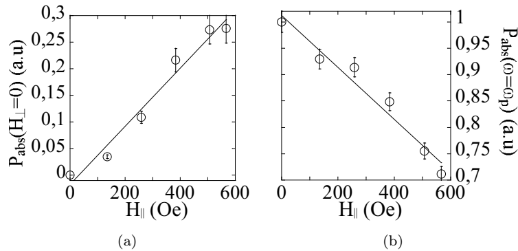
FIG. 4.22 – Evolution de la puissance micro-onde absorbée à H_{\perp} \sim 0 (gauche) et à la résonance plasma (droite) en fonction de H_{\parallel} . Ces données sont extraites de la figure 4.21. La ligne d'ajustement pour l'évolution de la puissance à la RPJ (droite) est calculée avec l'expression (4.36) avec \alpha = 8 .
