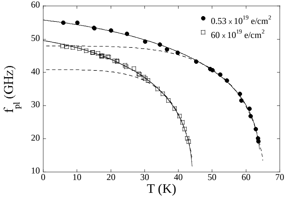
FIG. 3.10 – Fréquence plasma des échantillons MW100-5 et MW100-5b. Les lignes en pointillés représentent l'ajustement (3.25) et celles en trait plein, l'ajustement (3.26).
