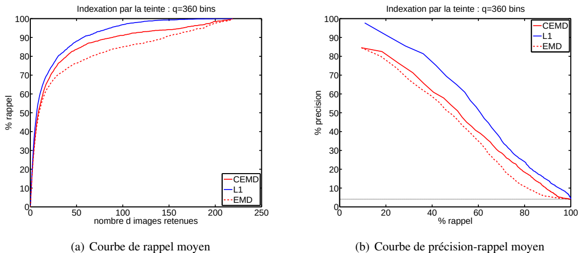
FIG. 6.16 – Courbes de précision-rappel moyen de l'indexation d'une base d'images avec changement de la balance des blancs. La distance de transport CEMD est représentée en trait rouge continu, l'EMD (correspondant à un transport sans prise en compte de la circularité de la teinte) en trait rouge interrompu, et la distance L^1 en trait bleu continu.
