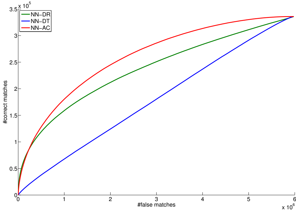
FIG. 2.9 – Courbes ROC globales obtenues en utilisant le même seuil de détection sur toute la base, avec le protocole A \rightarrow \{A'_B\} , où chaque image est mise en correspondance avec sa version dégradée A' et une autre image B . Trois critères sont testés avec la restriction au plus proche voisin : NN-AC en rouge, NN-DT en bleu et NN-DR en vert.
