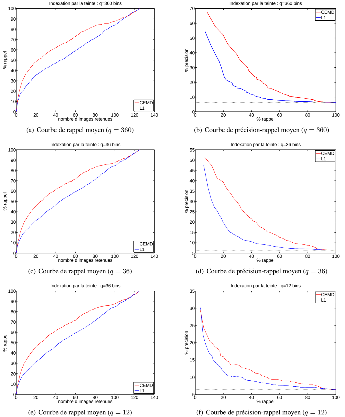
FIG. 6.7 – Indexation d'une base d'objet en prise de vue fixe selon différents réglages de la caméra. Les courbes de précision-rappel moyen sont tracées selon différentes quantifications, avec un nombre de bins égal q = 360, 36 , et 12 . Le trait rouge continu représente la distance CEMD, le trait rouge interrompu la distance EMD (transport sans tenir compte de la circularité), et le trait bleu continu la distance L^1 .
