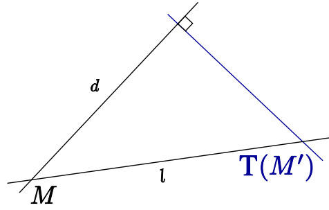
FIG. 3.7 – Illustration de l’erreur de transfert définie comme la distance l entre le point m et le point Tm' pour une transformation planaire T , et la distance d entre le point m et la droite F^T m' pour la géométrie épipolaire.
