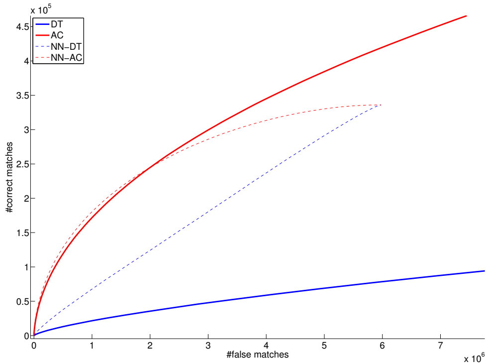
FIG. 2.12 – Courbes ROC globales obtenues en utilisant le même seuil de détection sur toute la base, avec le protocole A \rightarrow \{B^{A'}\} , où chaque image est mise en correspondance avec sa version dégradée A' et une autre image B . Deux critères sont testés avec et sans restriction au plus proche voisin. En trait continu, les critères de mise en correspondance multiple : AC en rouge et DT en bleu. En trait interrompu, les critères restreints au plus proche voisin : NN-AC en rouge et NN-DT en bleu.
