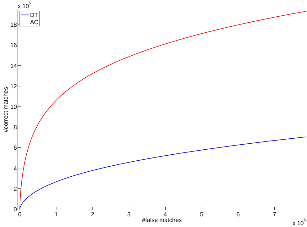
FIG. 2.11 – Courbes ROC globales obtenues avec le protocole A \rightarrow \{B^{A'+A''}\} , où l'image A' + A'' contient deux fois l'objet requête. Deux critères sont testés sans restriction au plus proche voisin : AC en rouge et DT en bleu.
