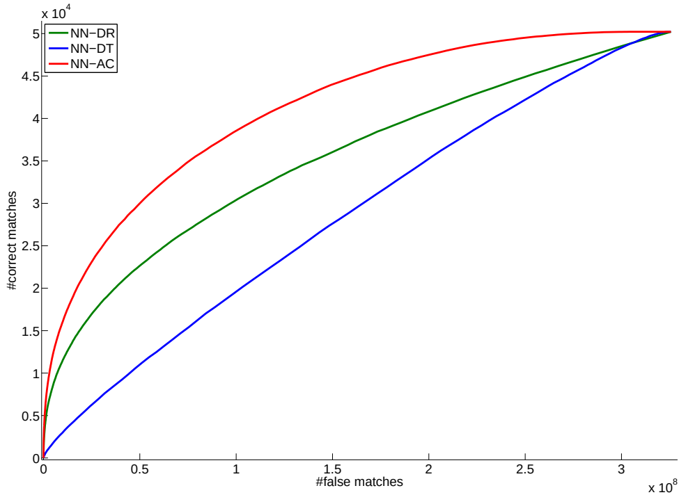
FIG. 2.10 – Courbes ROC globales obtenues en utilisant le même seuil de détection sur toute la base, avec le protocole A \rightarrow \{A'_{Base \setminus A}\} sur 100 images, où chaque image A est mise en correspondance avec sa version dégradée A' et toutes les autres images de la base de données (soit 731 images). Trois critères sont testés avec la restriction au plus proche voisin : NN-AC en rouge, NN-DT en bleu et NN-DR en vert.
