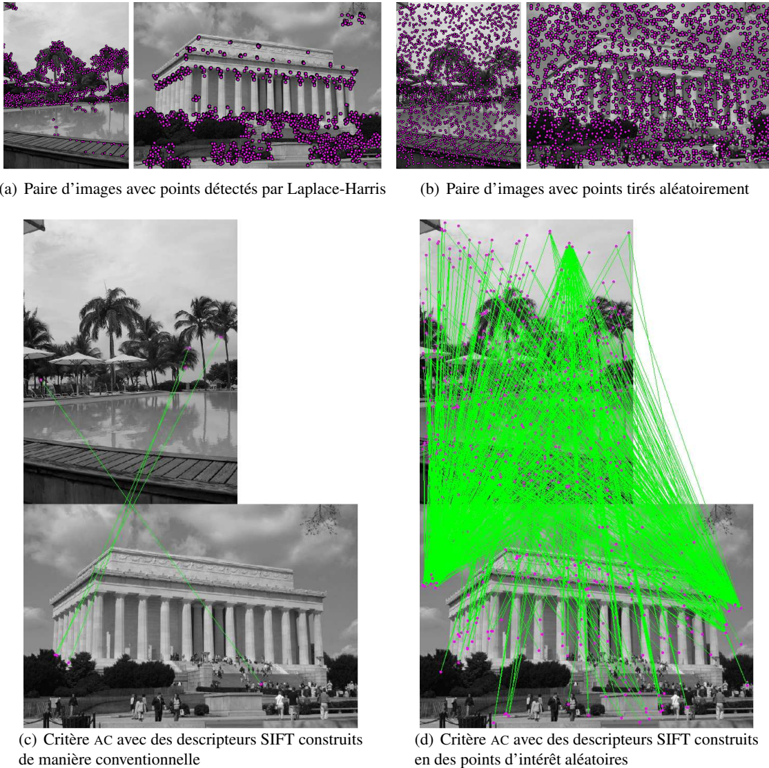
FIG. 2.3 – Illustration de l'importance du détecteur de points d'intérêt pour le critère de correspondance.
