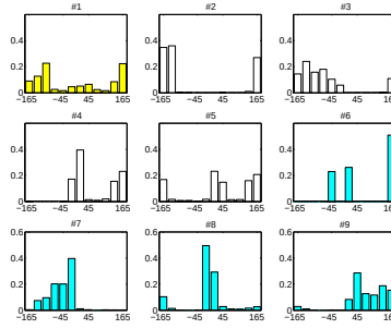
FIG. B.9 – Exemple de 9 histogrammes d’orientation du gradient extraits de chacune des régions correspondantes.
