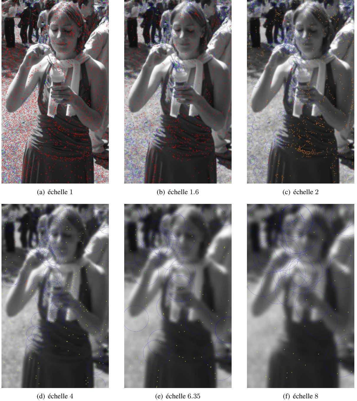
FIG. B.3 – Illustration de l'élimination des points de bord avec le critère de Harris multi-échelle. Les points rejetés sont en rouge, et les points valides sont en vert, entourés par un cercle bleu de rayon proportionnel à l'échelle de détection.
