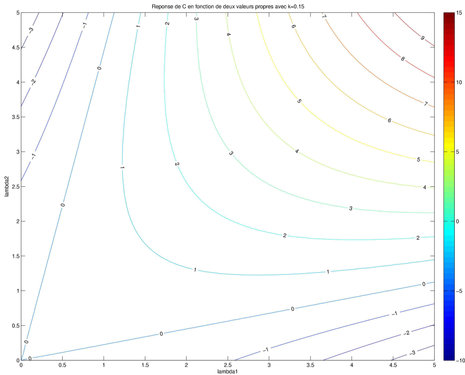
FIG. B.2 – Réponse de la mesure de ressemblance C pour k = 0.15 en fonction des valeurs propres de la matrice C_\sigma(x, y) .
