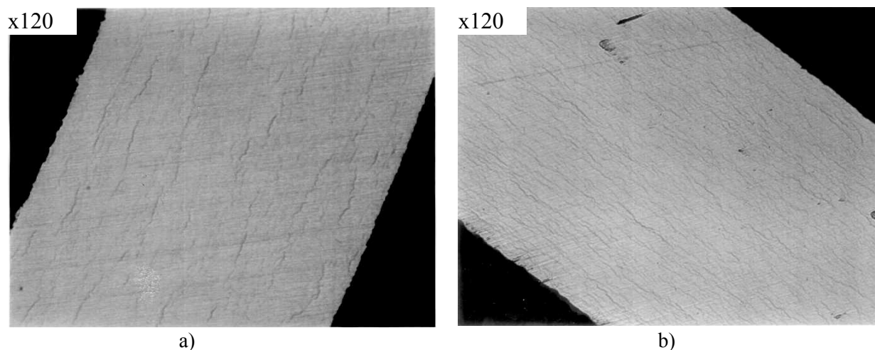
Figure IV. 28. Hydrures de zirconium sur une coupe transversale d'un tube oxydé a) en autoclave et b) sous vapeur d'eau
