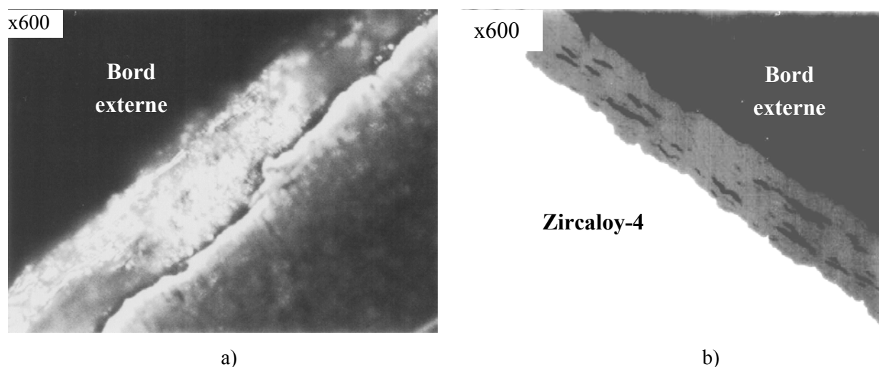
Figure IV. 30. a) ondulation de l'interface zircone/zircaloy 4 et b) porosités dans la zircone
