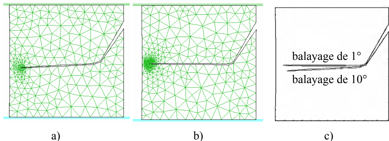
Figure III. 15. Critère TREM pour un balayage de 10° (a) de 1° (b) et comparaison des trajectoires (c)
