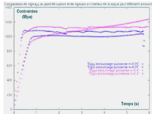
Figure IV. 23. Contraintes xx et yy en fonction de l'écroutissage
