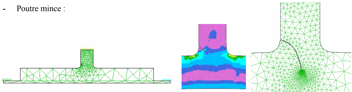
Figure III. 45. Chemin de propagation pour une poutre mince
