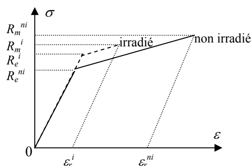
Figure IV. 5. Influence de l'irradiation sur la courbe contrainte-déformation
