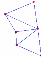
Figure A. 5. Itération finale
