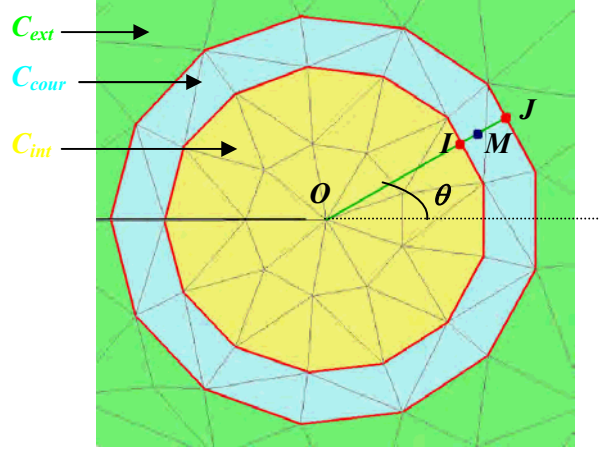
Figure II. 25. Couronnes d'intégration pour la méthode G0
