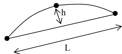
Figure A. 2. Le paramètre courbure
