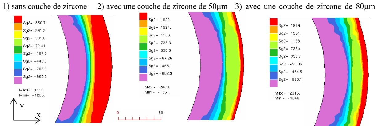
Figure IV. 42. Contrainte \sigma_{yy} en fonction de l'épaisseur de zircon
