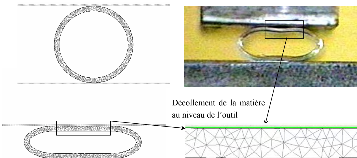
Figure IV. 12. Compactage d'un tube
