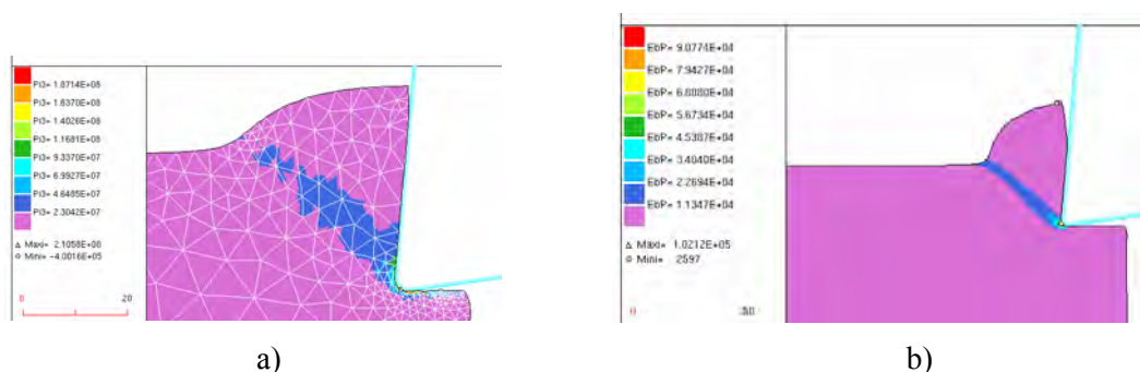
Figure III. 36. a) Taux de cisaillement et b) vitesse de déformation équivalente
