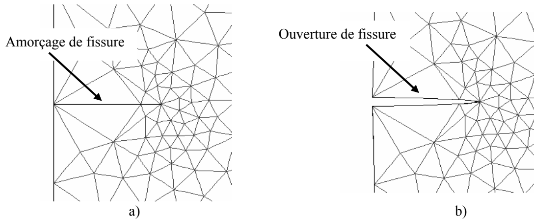
Figure III. 2. Amorce d'une fissure a) ajout d'un contour – b) dédoublement des nœuds
