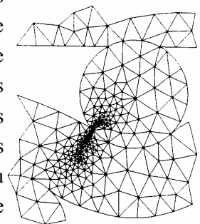
Figure I. 22. Exemple d'agglomération de nœuds
