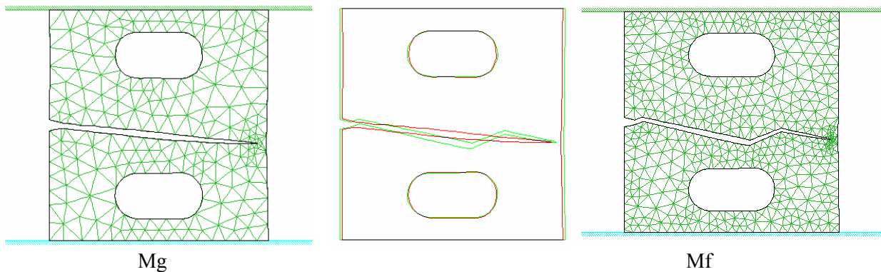
Figure D. 5. Propagation avec le critère CNM2 pour les maillages fin Mf et grossier Mg
