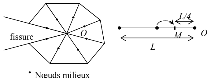
Figure II. 18. Déplacement des nœuds milieux
