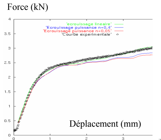
Figure IV. 13. Courbes Force/Déplacement pour trois écrouissages différents
