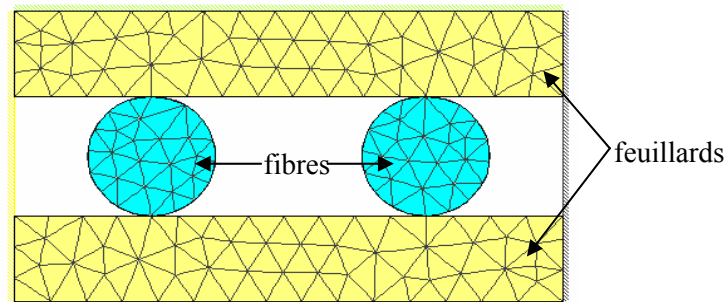
Figure I. 11. Maillage composé de deux fibres et de deux feuillards
