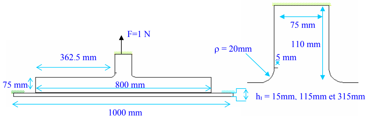
Figure III. 44. Géométrie de l'éprouvette bicouche pré-fissurée
