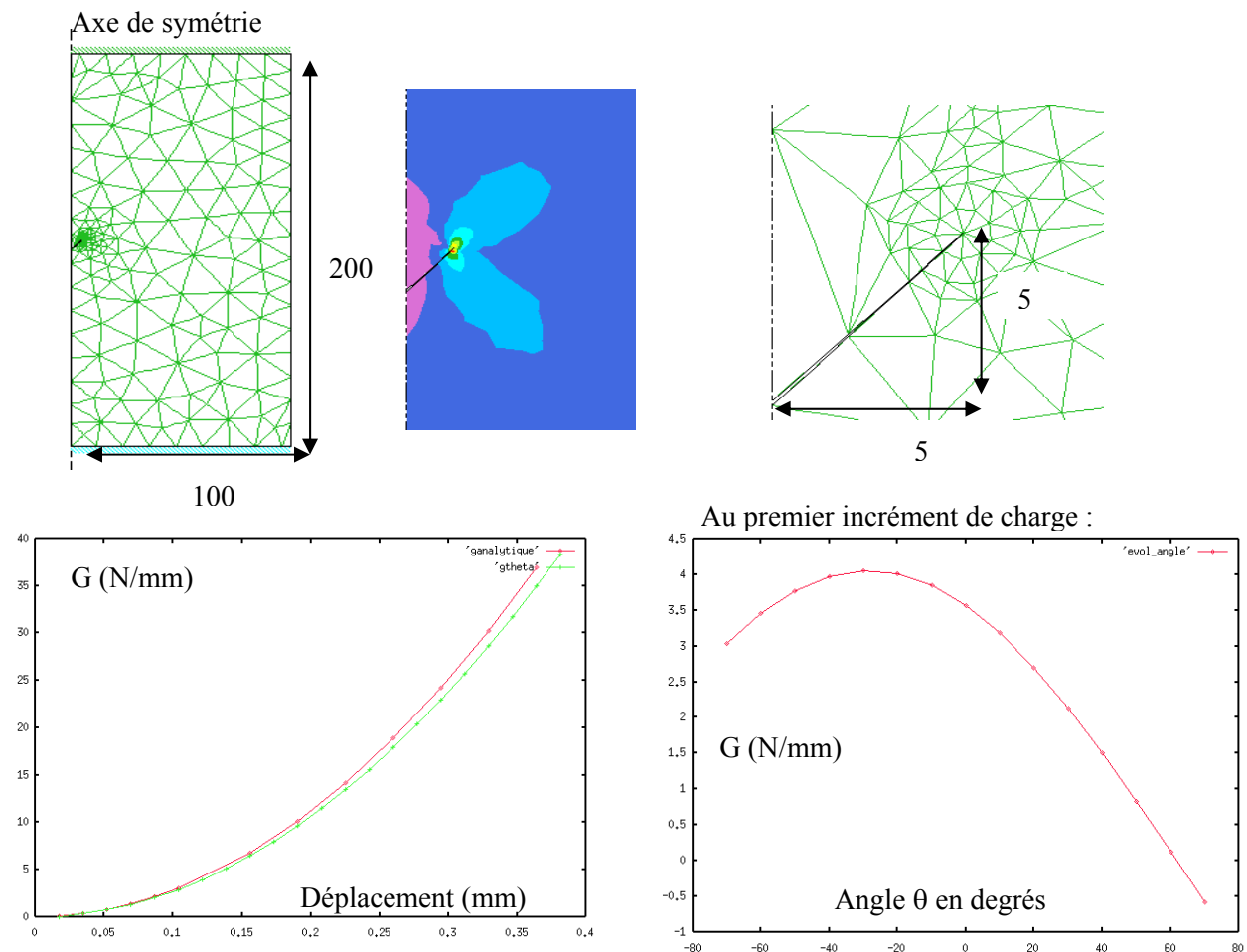
Figure II. 35. G pour une fissure inclinée à 45^\circ
