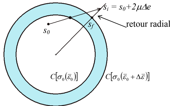
Figure I. 3. Méthode du retour radial
