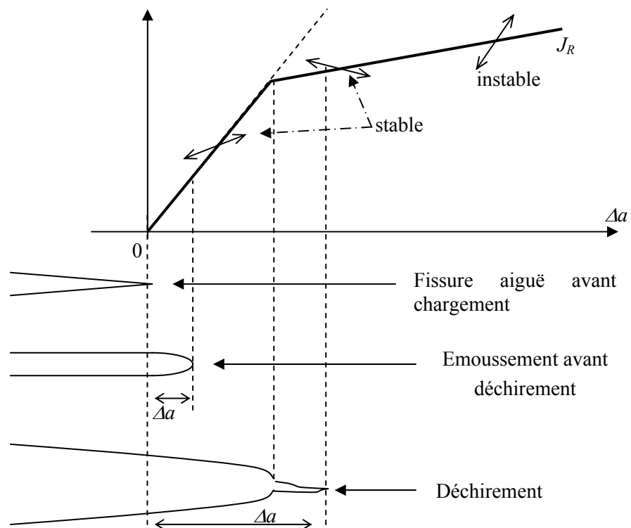
Figure C. 2. Courbe de résistance J_R=f(\Delta a) et stabilité de propagation
