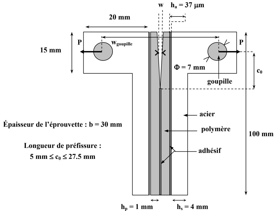
Figure I. 25. Epreuve de clivage colle/polymère/acier
