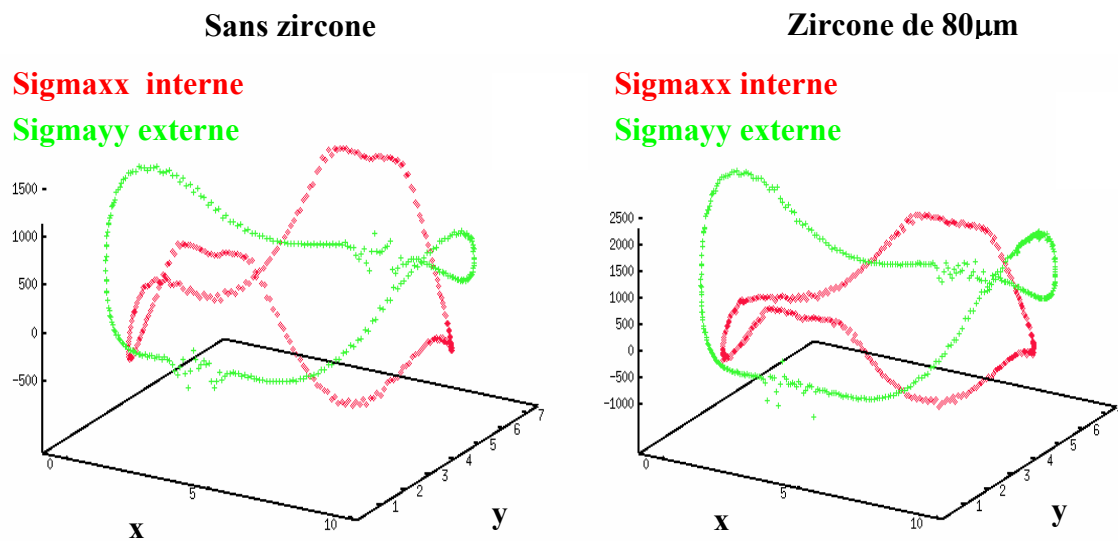
Figure IV. 44. \sigma_{xx} et \sigma_{yy} sur les contours interne et externe d'un tube non oxydé, et oxydé
