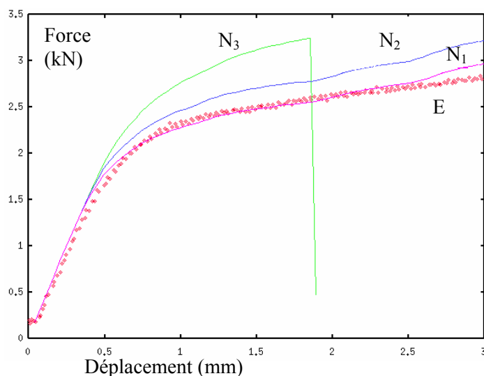
Figure IV. 9. Comparaison de la courbe Force/Déplacement expérimentale et des résultats numériques pour un essai de compactage d'un tube simple
