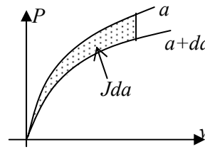
Figure II. 8. Détermination de J par la méthode de la complaisance
