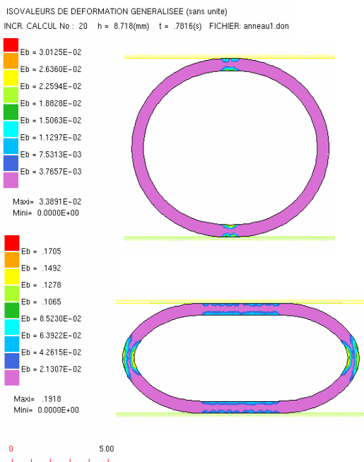
Figure IV. 18 Evolution de la déformation généralisée au cours du compactage
