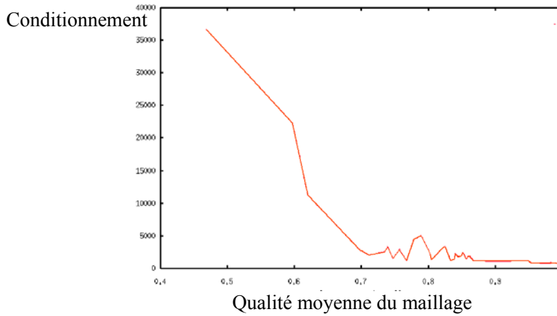
Figure I. 29. Influence de la qualité moyenne du maillage sur le conditionnement
