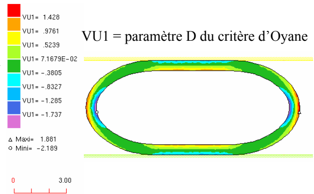
Figure III. 6. Endommagement selon le critère d'Oyane pour le compactage d'un tube
