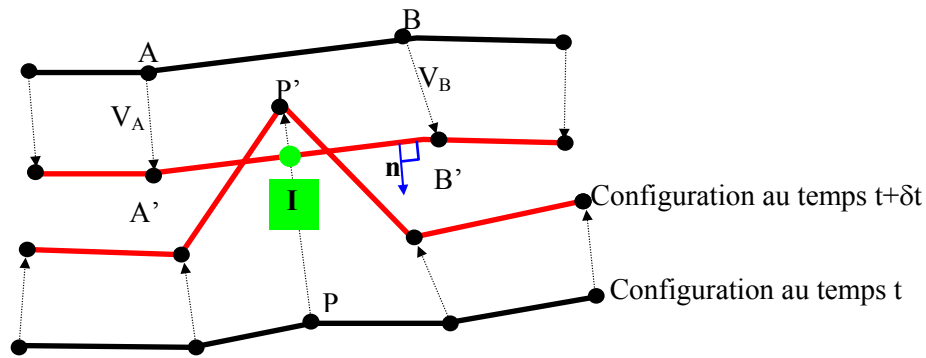
Figure III. 40. Pénétration d'un nœud appartenant à une fissure
