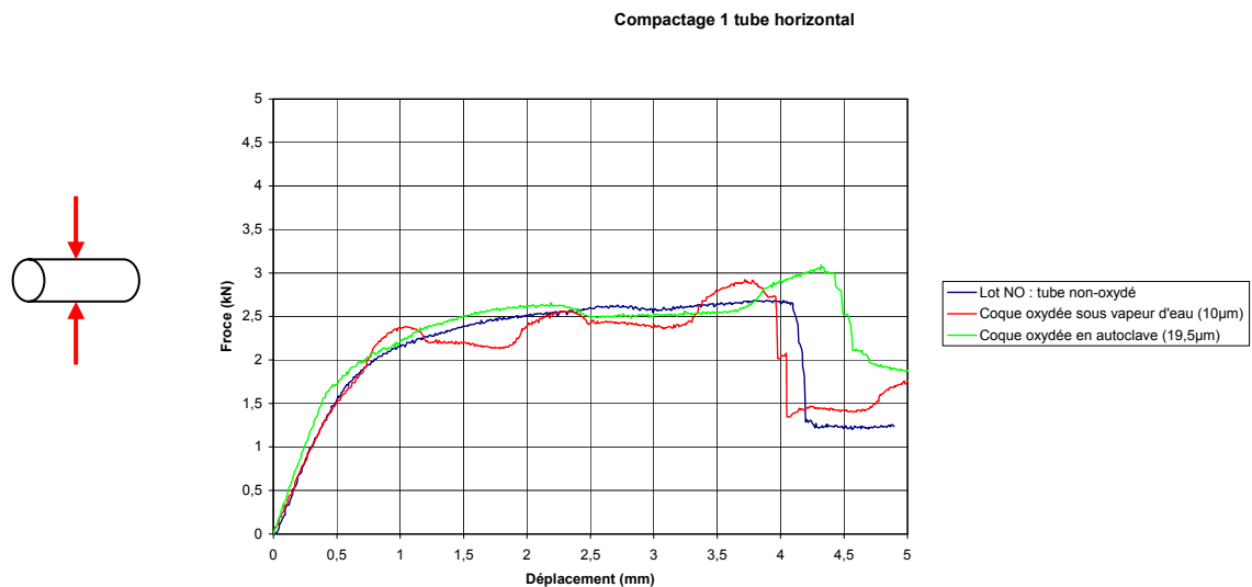
Figure IV. 32. Comparaison des courbes Force/Déplacement pour un essai de compactage horizontal
