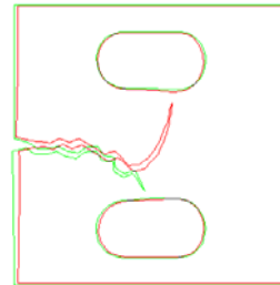
Figure D. 8. Propagation avec le critère CNM3
