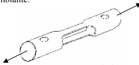
Figure IV. 6. Eprouvette de traction dans le sens longitudinal.
