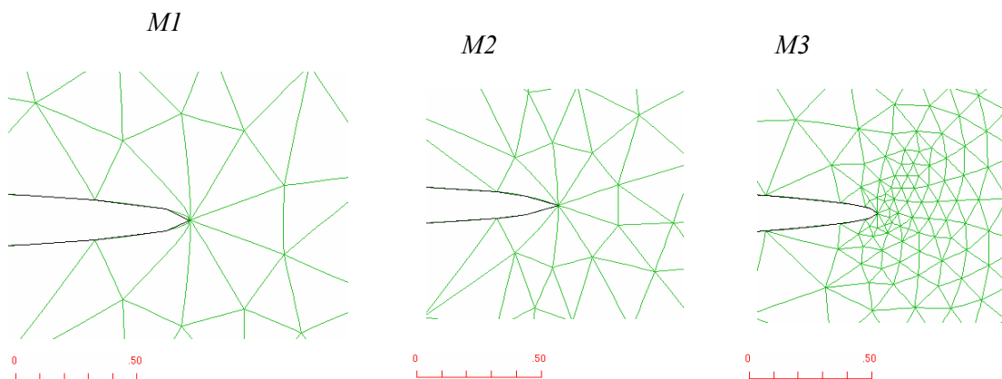
Figure II. 22. Différentes finesses de maillage en pointe de fissure
