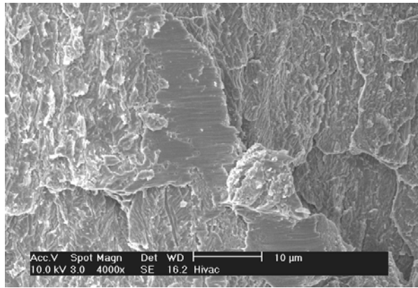
Figure IV. 36. Zone centrale : Domaine ductile avec des phases fragiles
