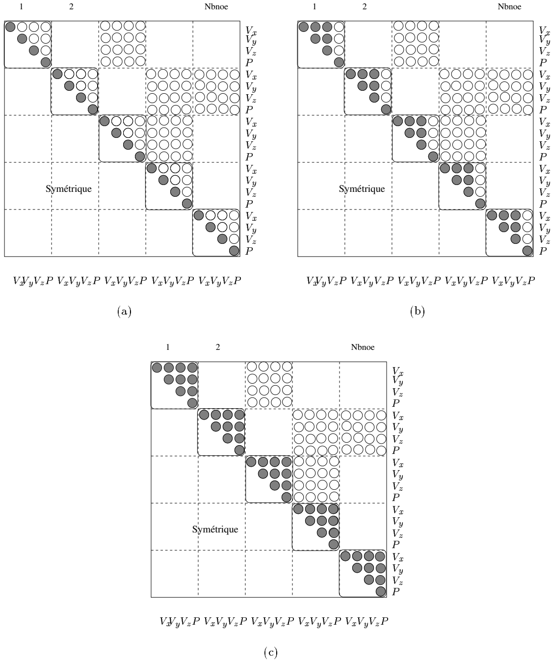
FIG. 3.2 – Termes de la matrice concernés par le préconditionneur (a) préconditionneur diagonal, (b) Préconditionneur bloc vitesse et valeur absolue de la diagonale, (c) Préconditionneur bloc vitesse pression
