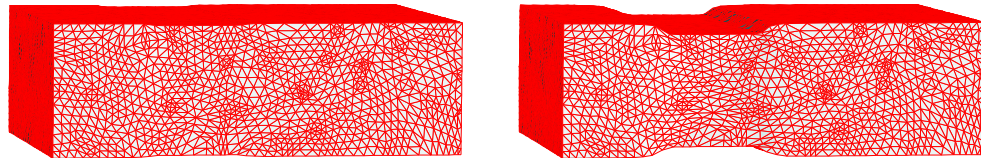
FIG. 3.33 – Déformation du lopin après 7 et 60 incréments sur le cas de martelage
