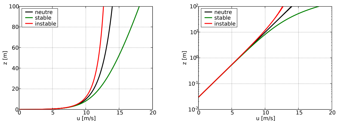
FIG. 1.2 – Profils verticaux de la vitesse du vent établis avec la loi logarithmique pour différentes conditions de stabilité.
