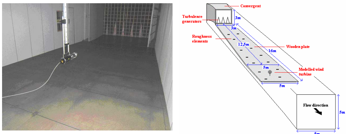
FIG. 9.5 – Veine de retour de la soufflerie « Malavard » (España et al. , 2008).
