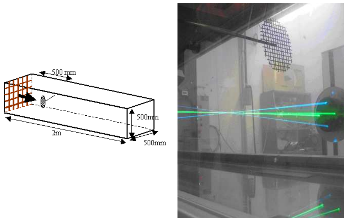
FIG. 9.4 – Soufflerie à veine ouverte (España et al. , 2008).
