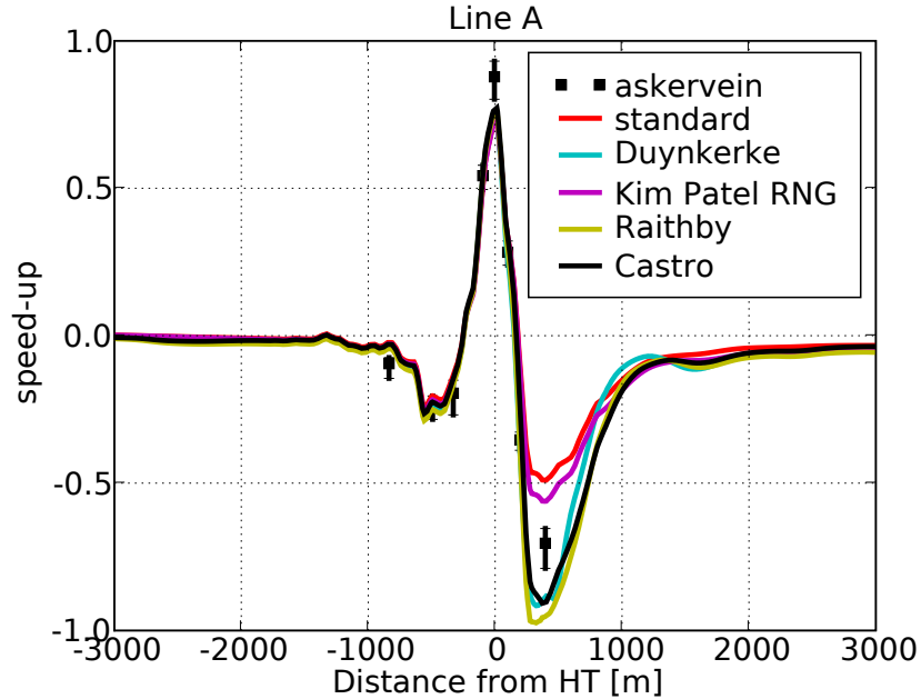
FIG. 4.19 – Sensibilité aux constantes du modèle k - \epsilon . Survitesse le long de la ligne A.
