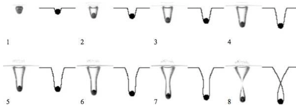
FIG. 2.14 – Comparaison entre des images obtenues à la caméra rapide et des profils numériques de cavité, pour l’impact dans l’eau d’une bille de verre ( d = 11,5 mm, V_0 = 2,4 m/s, \rho_s = 2500 kg/m 3 ). Intervalle entre deux images consécutives : 3,65 ms. Figure extraite de [42].
