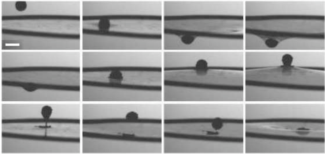
FIG. 4.7 – Chronophotographie du rebond d'une goutte de glyc rol enrob e de lycopodes sur un film de savon. La barre blanche repr sente 5 mm et l'intervalle entre deux images cons cutives est de 8 ms. (Clich s Elsa Bayart)
