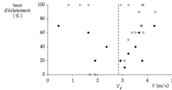
FIG. 4.21 – Taux d'éclatement des films en fonction de la vitesse d'impact pour des billes de verre de 6 mm de diamètre nues ( \circ ) ou enrobées d'huile ( \bullet ) et des billes de polypropylène superhydrophobes de 4,8 mm de diamètre ( \times ). Au-delà de la vitesse V_d \simeq 2,8 m/s, les billes de verre se comportent de la même manière, qu'elles soient ou non couvertes d'huile.
