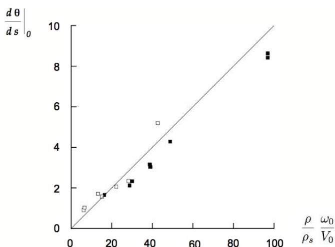
FIG. 3.11 – Pente à l’origine de \theta(s) , en fonction du paramètre \frac{\rho}{\rho_s} \frac{\omega_0}{V_0} . Les données expérimentales (■) sont comparées aux résultats de Truscott et Tchet (□).
