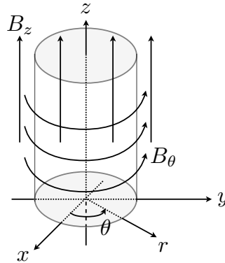
FIGURE 2.2 – Configuration « pinch »
