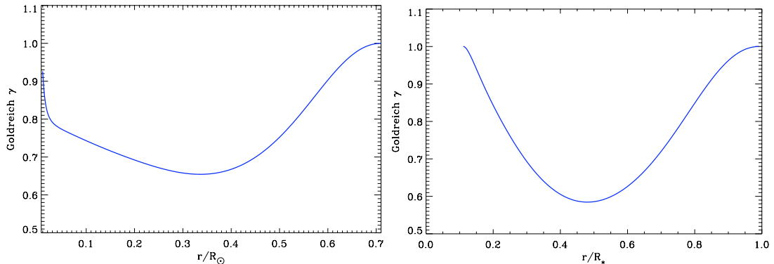
FIGURE 5.4 – Paramètre de Golreich ; (à gauche) dans le cas solaire et (à droite) dans celui de l'étoile de type Ap.
