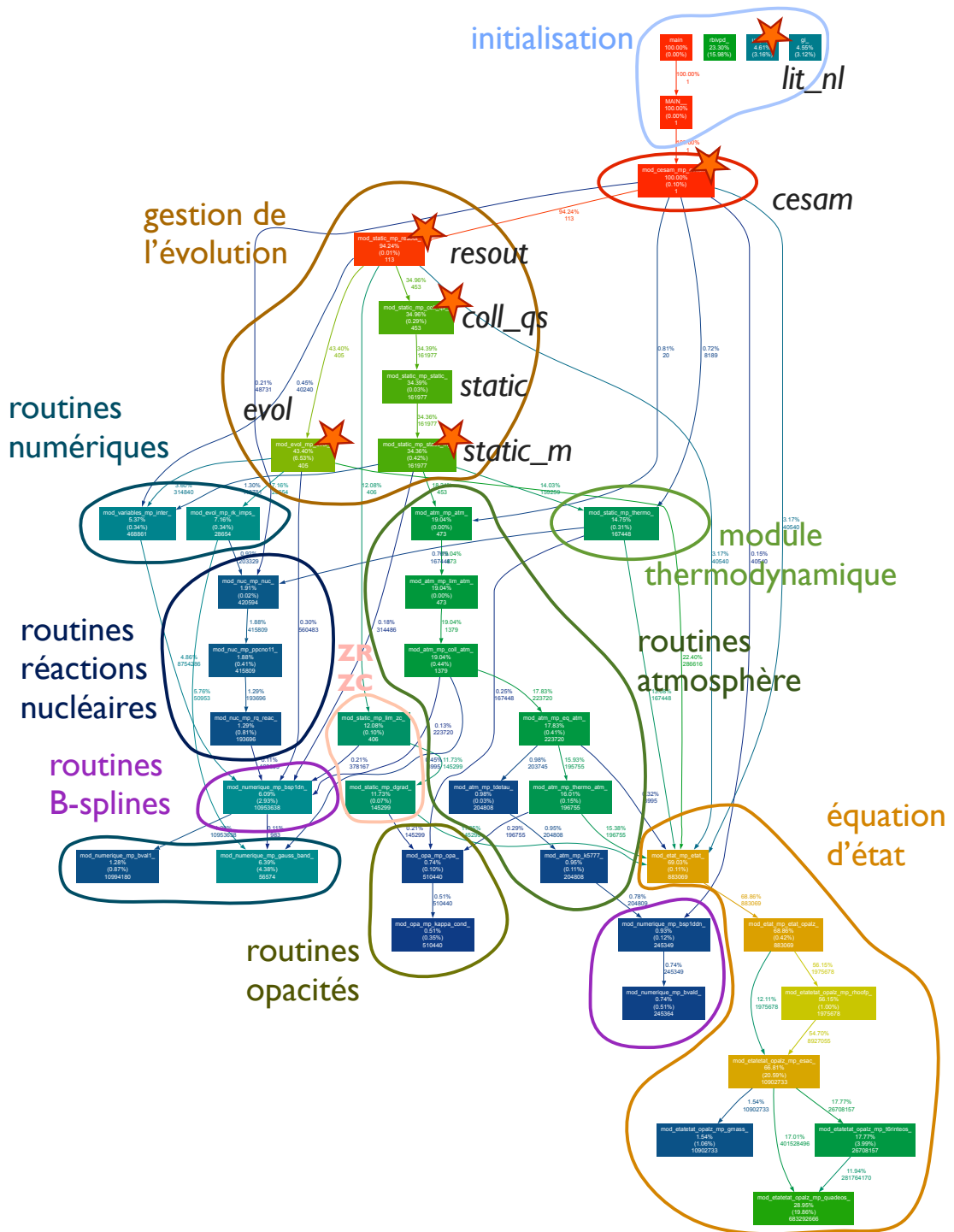
FIGURE 6.4 – Architecture du code CESAM mettant en lueur les différentes routines et leurs interconnexions. Celles ayant été modifiées pour inclure les effets du champ magnétique sont marquée d'une astérisque.
