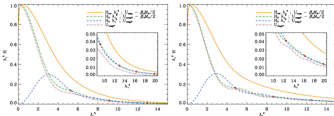
FIGURE 3.7 – Hélicités poloidale, toroïdale et totale (normalisée) du champ magnétique le cas (a, à gauche) du Soleil et (b, à droite) d'une étoile Ap.
