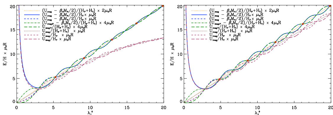
FIGURE 3.8 – Rapports \mathcal{E}_{\text{mag}}/\mathcal{H} poloidaux, toroïdaux et globaux avec prise en compte ou non de la contribution non force-free dans les cas (a, à gauche) du Soleil et (b, à droite) d'une étoile Ap.
