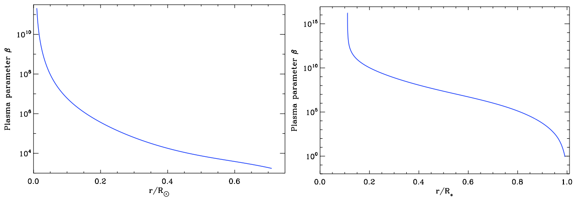
FIGURE 5.6 – Paramètre plasma \beta ; (à gauche) dans le cas solaire et (à droite) dans celui de l'étoile de type Ap.
