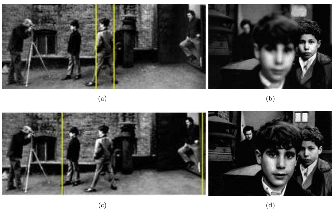
FIGURE A.7 – Influence de l'ouverture du diaphragme sur la profondeur de champs : dans (a) et (b), on utilise une ouverture f = 1/2 et la profondeur de champs est faible, dans (c) et (d) on utilise une ouverture f = 1/16 et la profondeur de champs est importante.
