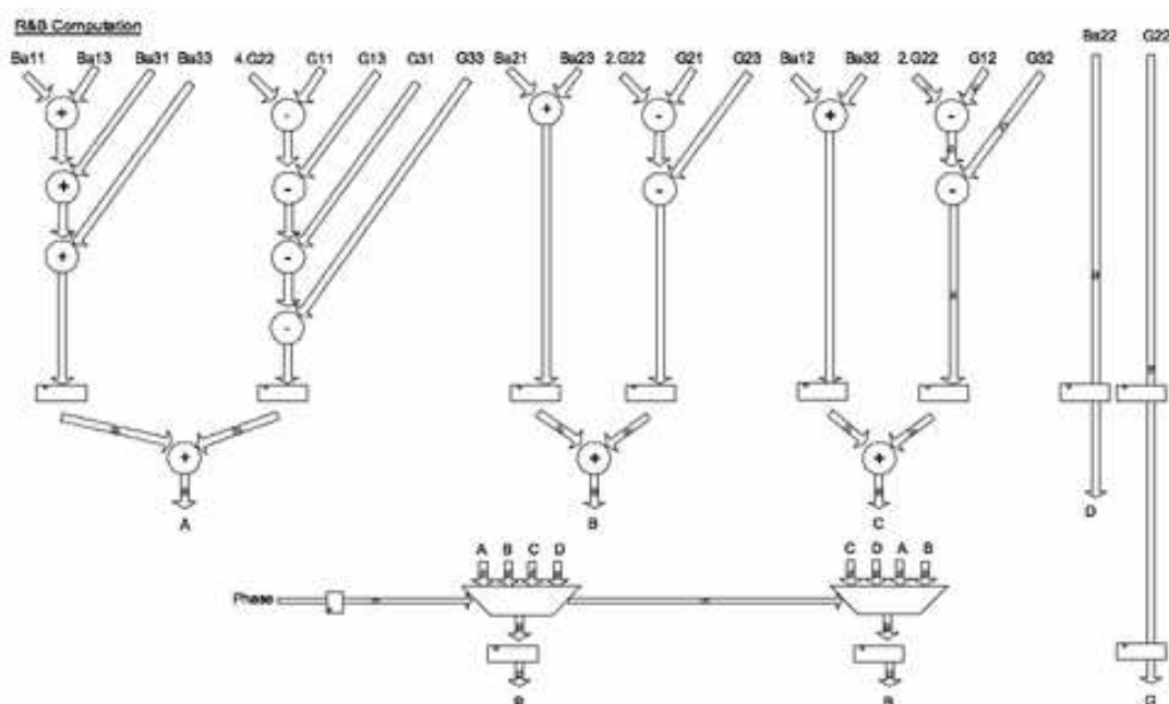
FIGURE 10.12 – Architecture du composants de calculs des pixels rouges et bleus
