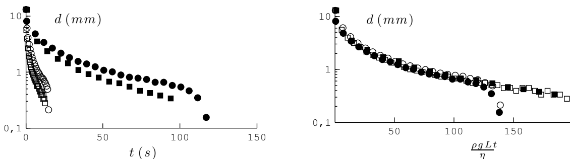
FIGURE 6.14 – Diamètre d du filament en fonction du temps (graphe de gauche) et en fonction de t/\tau_g . D = 13 mm, \eta = 12 Pa·s (symboles vides) ou \eta = 97 Pa·s (symboles pleins) et L = 14 mm ( \circ ) ou L = 22 mm ( \square ). Le drainage est beaucoup plus lent que prévu : il devrait avoir lieu sur un temps caractéristique \tau_g , qui est de l'ordre de la seconde pour l'huile la plus visqueuse.
