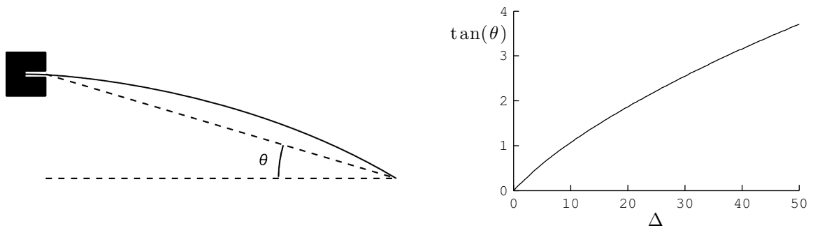
FIGURE B.3 – Méthode de mesure de la rigidité des racloirs : le racloir est encastrié horizontalement, et on observe la hauteur z_f de son extrémité libre. La courbe de droite permet de relier cette hauteur au nombre sans dimension \Delta = \frac{\rho_s g L^3}{B} , ce qui permet de déterminer B .
