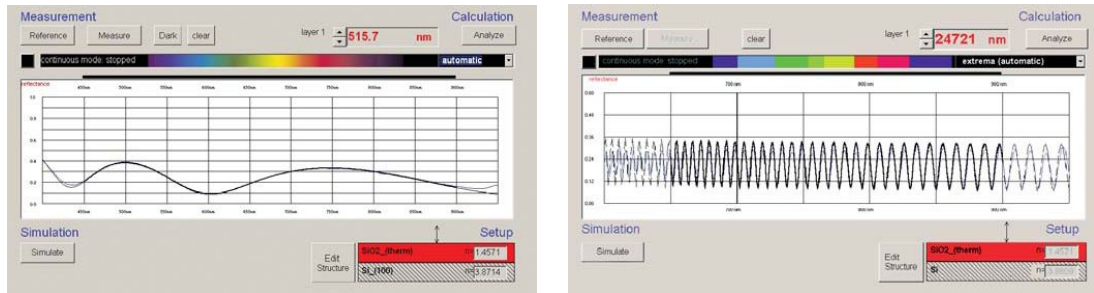
FIGURE 1.3 – Exemple de spectres obtenus : les graphes présentent le coefficient de réflexion de r l'échantillon en fonction de la longueur d'onde. A gauche : e_d = 0,5 \mu\text{m} . A droite : e_d = 25 \mu\text{m} .
