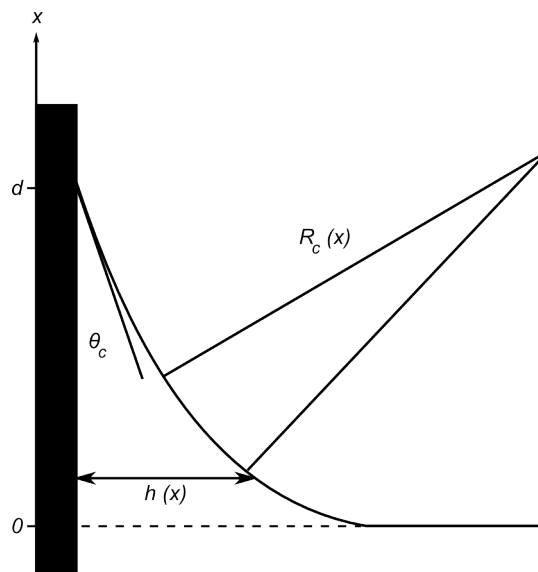
FIGURE 1.5 – Le ménisque statique connecte le bain de liquide horizontal à la surface solide, sur laquelle le liquide arrive avec un angle de contact \theta_c propre au couple liquide/solide considéré.
