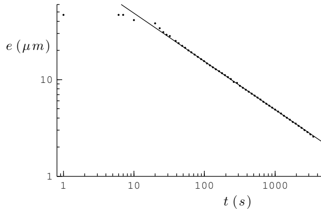
FIGURE 3.1 – Drainage d'un film d'huile silicone de viscosité \eta = 19,5 mPa·s sur un substrat lisse. La droite a pour équation e = \sqrt{\frac{\eta x_f}{\rho g t}} , avec x_f = 1,2 cm.
