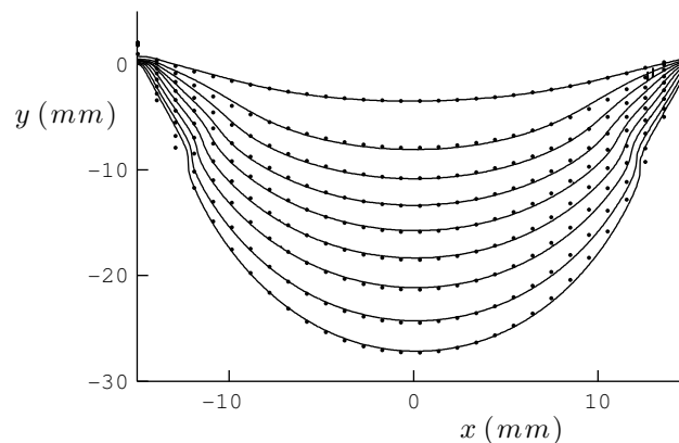
FIGURE 7.3 – Formes du filament de la figure 7.2 (traits pleins), et ajustements par une forme de chaînette (points) : y = a \cosh\left(\frac{x}{a}\right) + c .
