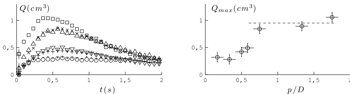
FIGURE 6.7 – Expériences d'entraînements avec D = 12 mm, \eta = 12 Pa·s, V = 19,1 mm/s et différentes profondeurs de bain p : 2 mm ( \circ ), 4 mm ( \cdot ), 6 mm ( + ), 7 mm ( \Delta ), 9 mm ( \nabla ), 16 mm ( \times ), 21 mm ( \square ).
