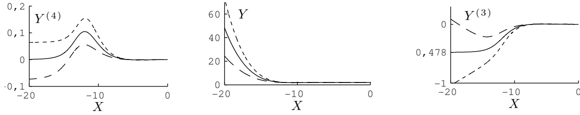
FIGURE 4.16 – Forme du raclor dynamique pour trois valeurs de Y(0) (figure centrale). La courbe en traits pleins présente Y(0) = 0,0012 , qui est comme l'illustre la première figure la valeur pour laquelle Y_{XXXX} \xrightarrow{X \rightarrow -\infty} 0 . La dérivée troisième du profil tend alors vers une constante (égale à -0,4780 ) lorsque X \rightarrow -\infty (figure de droite). Les autres courbes correspondent à Y(0) = 0,0017 (tirets courts) et Y(0) = 0,0007 (tirets longs).
