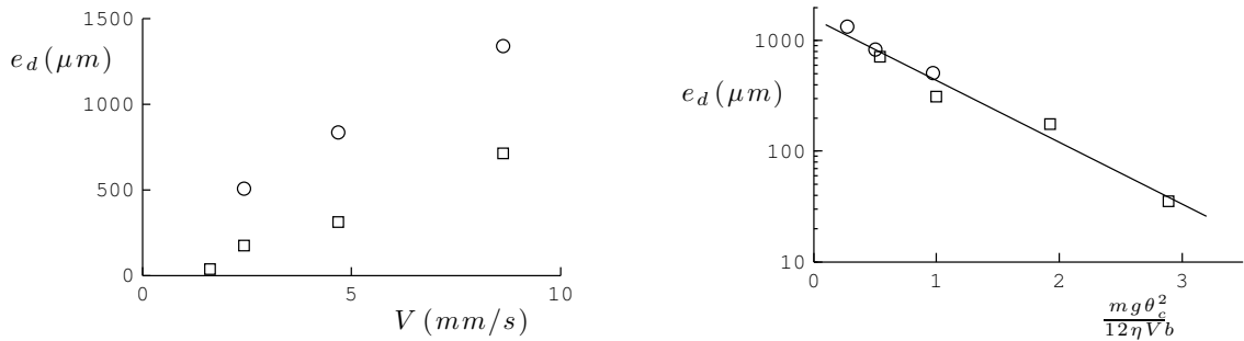
FIGURE 5.3 – À gauche : épaisseur de liquide déposée en fonction de la vitesse de tirage V , pour deux épaisseurs de racloirs : h = 1,5 mm ( \circ ) et h = 3 mm ( \square ). Les autres paramètres sont : \theta_c = 26,6^\circ ( y_0 = 25 mm et L = 50 mm), \eta = 17,4 Pa·s et b = 3 cm. À droite : ces mêmes expériences se superposent lorsqu'on adimensionne la vitesse. Un ajustement exponentiel de la forme e_d = e_M \exp(-ax) (traits pleins) fournit : e_M = 1,6 mm et a = 1,3 .
