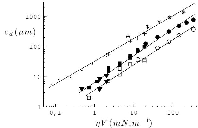
FIGURE 4.10 – Épaisseur déposée en fonction de \eta V , pour b = 3 cm, \eta = 0,1 Pa · s ( \nabla et \cdot ), \eta = 0,98 Pa · s ( \square et + ) et \eta = 17,4 Pa · s ( \circ et * ). Les grands symboles ( \circ , \square , \nabla ) sont pour L = 4 cm, les symboles pleins correspondant à un racloir de rigidité B = 4,2 \cdot 10^{-3} N · m et les symboles vides à B = 14,3 \cdot 10^{-3} N · m. Les petits symboles ( \cdot , + , * ) représentent L = 6 cm et B = 4,2 \cdot 10^{-3} N · m. Les lois de puissance représentées sont d'exposant 0,75, 0,88 et 0,83.
