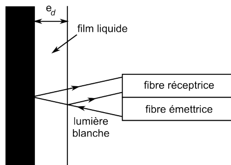
FIGURE 1.2 – Schéma de la sonde du réflectomètre. Un faisceau de lumière blanche est envoyé sur le film liquide. La lumière réfléchie est récupérée à l'aide d'une fibre optique et analysée par un interféromètre.
