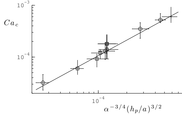
FIGURE 2.12 – Valeurs de Ca_c mesurées sur les surfaces étudiées, en fonction de \alpha^{-3/4}h_p^{1/2}a^{-1/2} , pour p = 10 \mu\text{m} ( \square ), p = 20 \mu\text{m} ( \circ ) et p = 28 \mu\text{m} ( + ). Les valeurs de \alpha ont également été mesurées à partir des expériences de dépôt. La droite a pour équation y = 1,06x .
