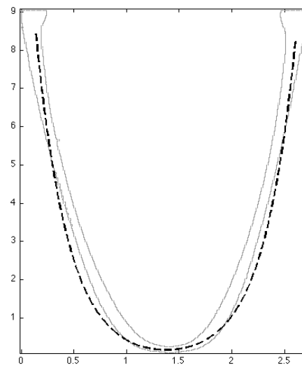
FIGURE 7.15 – À gauche : chaînette visqueuse d'huile silicone ( \eta = 9,7 \text{ Pa} \cdot \text{s} , L = 24 \text{ mm} et D = 2,3 \text{ mm} ), aux grandes déformations. À droite : on superpose à la forme de ce filament visqueux (en gris) la forme d'une chaînette (pointillés noirs) ayant les mêmes dimensions (les axes sont en centimètres).
