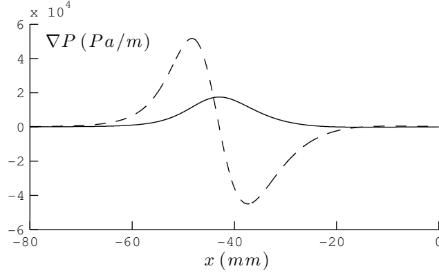
FIGURE 4.19 – La courbe en tirets correspond au gradient de pression longitudinal sous le raclor ( Bh_{xxxx} ), calculé par le modèle présenté pour \eta = 1 \text{ Pa}\cdot\text{s} , V = 10 \text{ mm/s} , B = 4 \cdot 10^{-3} \text{ N}\cdot\text{m} et L = 4 \text{ cm} . La courbe en traits pleins représente le gradient de pression transverse estimé Bh_{xxxx}/b , pour b = 3 \text{ cm} . On remarque que ces deux termes sont du même ordre de grandeur.
