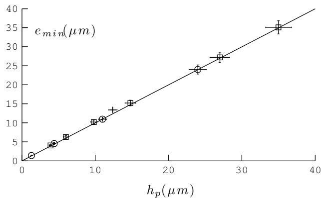
FIGURE 2.3 – Épaisseur minimale de liquide entraînée e_{min} en fonction de la hauteur des piliers h_p , pour des surfaces de pas p = 10 \mu\text{m} ( \square ), p = 20 \mu\text{m} ( \circ ) ou p = 28 \mu\text{m} ( + ). La droite représente e_{min} = h_p .
