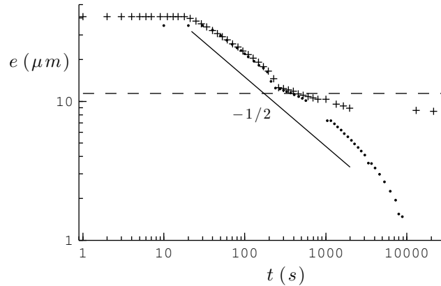
FIGURE 3.15 – Expérience de drainage pour p = 66 \mu\text{m} , h_p = 11,4 \mu\text{m} , \eta = 19,5 \text{ mPa} \cdot \text{s} . + : mesure en x = 4 \text{ mm} , valeur pour laquelle l'épaisseur en fin de drainage vaut 7 \mu\text{m} (cf. figure 3.14). • : mesure en x = 2 \text{ cm} > x_{max} , l'épaisseur finale est alors nulle. La ligne horizontale représente h_p , tandis que la droite en trait plein décrit une loi de puissance en t^{-1/2} , caractéristique du drainage sur une surface lisse.
