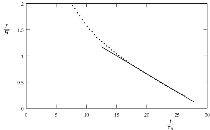
FIGURE 7.14 – L/H en fonction du temps adimensionné t/\tau_g . Le liquide utilisé est de l'huile silicone de viscosité 9,7 \text{ Pa} \cdot \text{s} . Les dimensions initiales du filament sont L = 24 \text{ mm} et D = 2,3 \text{ mm} .
