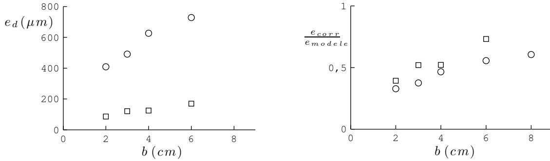
FIGURE 4.18 – Épaisseur de liquide déposé pour différentes largeurs de dépôt b . L = 4 cm (○) ou L = 2 cm (□), toujours dans la configuration de "mouillage total" ( \tilde{y}_0 = \tilde{y}_m , soit y_0 = 18,4 mm et y_0 = 9,2 mm, respectivement). Les autres paramètres de l'expérience sont \eta = 17,4 Pa·s, V = 8,2 mm/s, B = 4,2 \cdot 10^{-3} N·m. Dans le graphe de droite, l'épaisseur a été corrigée pour tenir compte de la différence entre la largeur de la plaque de dépôt et la largeur du racloir, et adimensionnée par l'épaisseur prédite par le modèle (1,5 mm pour L = 4 cm et 260 \mu m pour L = 2 cm).
