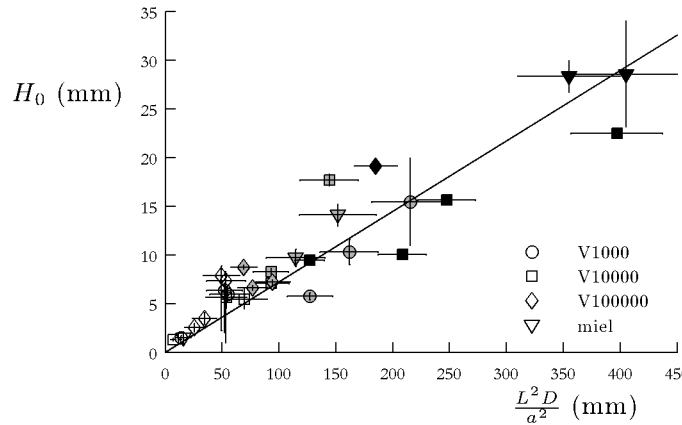
FIGURE 7.18 – L'équilibre entre forces capillaires et poids du filament détermine la hauteur d'équilibre du U.
