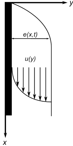
FIGURE 3.2 – Schéma du film liquide
