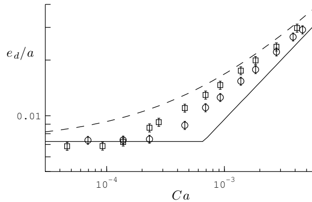
FIGURE 2.4 – Expérience de dépôt sur deux surfaces ne différant que par leur pas. \square : h_p = 9,8\ \mu\text{m} , p = 10\ \mu\text{m} . \circ : h_p = 11\ \mu\text{m} , p = 20\ \mu\text{m} . Les tirets et la courbe pleine correspondent respectivement à e_d = h_p + e_{LLD} et e_d = \max(e_{LLD}, h_p) .
