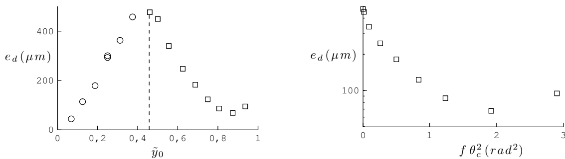
FIGURE 5.6 – À gauche : épaisseur e_d déposée par un racloir flexible en fonction de \tilde{y}_0 . Dans cette expérience, V = 8,2 \text{ mm/s} , B = 4,2 \cdot 10^{-3} \text{ N} \cdot \text{m} , L = 4 \text{ cm} et \eta = 17,4 \text{ Pa} \cdot \text{s} . Les pointillés représentent \tilde{y}_0 = \tilde{y}_m . À droite : les données pour y_0 > y_m sont tracées en fonction de f \theta_c^2 (les autres correspondent à \theta_c = 0 ), dans un diagramme semilogarithmique. On n'observe pas la décroissance en \exp(-f \theta_c^2) attendue pour un racloir rigide.
