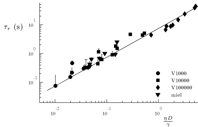
FIGURE 7.11 – Temps de rupture \tau_r des U en fonction du temps caractéristique du drainage capillaire \tau_\gamma = \eta D / \gamma . Les différents symboles correspondent aux différents liquides utilisés (huiles V1000, V10000 et V100000 de viscosités respectives 0,97 Pa · s, 9,7 Pa · s et 97 Pa · s, et miel de viscosité 5 Pa · s). La droite indique la variation linéaire \tau_r = 7,5 \tau_\gamma .
