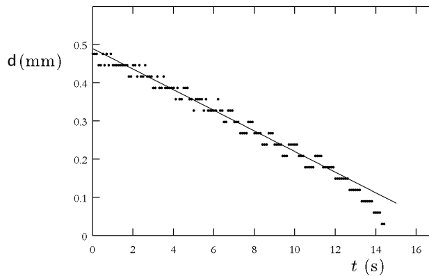
FIGURE 7.10 – Diamètre d du filament en fonction du temps, pour un filament d'huile silicone de viscosité 97 \text{ Pa}\cdot\text{s} . Le diamètre initial du filament vaut 0,5 \text{ mm} et sa longueur 12 \text{ mm} . La droite correspond à une décroissance linéaire à la vitesse de 27 \mu\text{m/s} .
