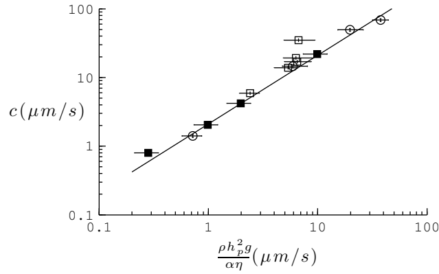
FIGURE 3.7 – Vitesse de translation du film mesurée c en fonction de la prédiction du modèle à deux couches (équation 3.4). \alpha est tiré des expériences de dépôt (partie 2.4, page 34). La droite a pour équation y = 2,1x . Les mesures ont été réalisées avec de l'huile de viscosité \eta = 19 \text{ mPa} \cdot \text{s} sur des surfaces de pas p = 10 \mu\text{m} ( \square ) et p = 20 \mu\text{m} ( \circ ) et différentes hauteurs de piliers h_p . Les symboles pleins représentent les mesures réalisées pour p = 10 \mu\text{m} , h_p = 10,2 \mu\text{m} et des viscosités \eta = 9,5 \text{ mPa} \cdot \text{s} , \eta = 48 \text{ mPa} \cdot \text{s} , \eta = 97 \text{ mPa} \cdot \text{s} , \eta = 340 \text{ mPa} \cdot \text{s} .
