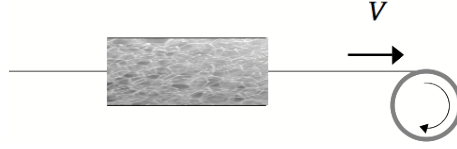
FIGURE D.2 – Schéma du montage de dépôt de mousse sur une fibre.
