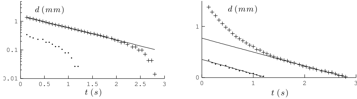
FIGURE 6.12 – Diamètre d du filament en fonction du temps, pour D = 2 mm, \eta = 12 Pa·s, et deux longueurs d'extraction : L = 14 mm (●) et L = 5 mm (+). Les courbes en trait plein montrent une décroissance exponentielle de d (graphe de gauche) avec un temps caractéristique de 0.7 s ou une décroissance linéaire (graphe de droite), avec des vitesses de -0,28 mm/s ( L = 14 mm) et -0,27 mm/s ( L = 5 mm).
