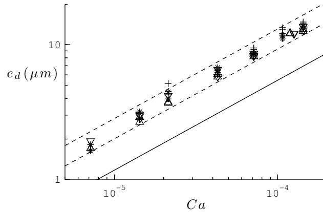
FIGURE 1.12 – Expériences de "dip-coating" réalisées avec de l'eau sur une lame de verre. Les symboles correspondent à différents traitements de la lame de microscope : neuve ( \bullet ), nettoyée à l'acétone ( + ), polie à l'aide d'une solution d'oxyde de Cérium ( \Delta ), nettoyée au mélange "piranha" ( \nabla ). La droite en trait plein représente la loi de LLD, et les tirets une épaisseur supérieure d'un facteur 1,7 et 2,4 à cette loi.
