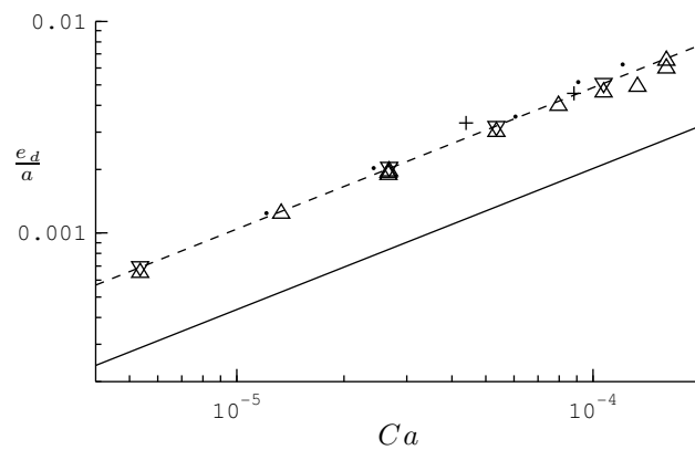
FIGURE 1.13 – Expériences de dépôt pour différents couples liquide/solide : mélange eau-glycérol à 60% en masse de glycérol ( \eta = 8,1 \text{ mPa} \cdot \text{s} , \gamma = 67 \text{ mN/m} ) sur lame de microscope neuve ( \bullet ), dodécane ( \eta = 1,35 \text{ mPa} \cdot \text{s} , \gamma = 25 \text{ mN/m} ) sur lame de microscope neuve ( \Delta ) et sur wafer en Silicium ( \nabla ), éthylèneglycol ( \eta = 1,1 \text{ mPa} \cdot \text{s} , \gamma = 48 \text{ mN/m} ) sur lame de microscope polie ( + ). La droite en trait plein représente la loi de LLD, et les tirets une épaisseur supérieure d'un facteur 2,4 à cette loi.
