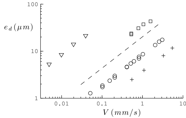
FIGURE 1.4 – Épaisseur e_d déposée en fonction de la vitesse de tirage V , pour des huiles de viscosités 2,7 \text{ mPa} \cdot \text{s} (+), 9,5 \text{ mPa} \cdot \text{s} (o), 96,5 \text{ mPa} \cdot \text{s} (□), et 980 \text{ mPa} \cdot \text{s} (▽). La courbe tiretée représente une loi de puissance d'exposant 2/3 .
