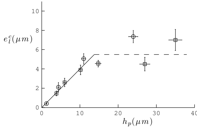
FIGURE 3.8 – Hauteur du film libre e_l^c juste avant la marche d'épaisseur, en fonction de h_p , pour des surfaces de pas p = 10 \mu m ( \square ) et p = 20 \mu m ( \circ ). e_l^c est proportionnel à h_p tant que h_p < 15 \mu m , puis sature à environ 5,5 \mu m pour p = 10 \mu m (tirets). La droite a pour équation e_l^c = 0,4 h_p .
