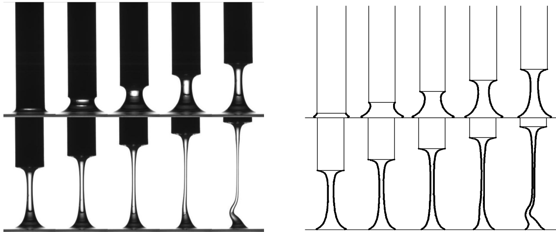
FIGURE 6.3 – Chronophotographie d'une expérience d'entraînement : D = 13 mm, V = 25 mm/s, \eta = 12 Pa·s. L'intervalle entre deux images est de 0,2 s. Le volume de liquide entraîné est maximal aux alentours de la troisième image, soit pour t \approx 0,5 s. L'image de droite présente les profils de filaments obtenus à partir des photos.
