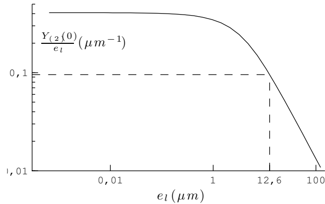
FIGURE A.3 – Y^{(2)}(0)/e_l en fonction de e_l , pour \alpha = 10 et h_p = 10 \mu\text{m} . e_{min} vaut alors 6 \cdot 10^{-7} \mu\text{m} et X_0 2,8 \cdot 10^5 . La droite horizontale représente le membre de droite de l'équation A.3 pour Ca = 10^{-3} , ce qui correspond à une épaisseur entraînée e_l = 12,6 \mu\text{m} .
