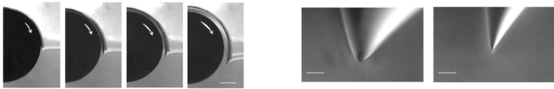
FIGURE 3 – À gauche : déformation de l'interface d'un bain d'huile silicone de viscosité \eta = 0,97\text{ Pa}\cdot\text{s} pour différentes vitesses de cylindre ( 6\text{ cm/s} , 10\text{ cm/s} , 17\text{ cm/s} , et 30\text{ cm/s} ). La barre dans la dernière image représente 1\text{ cm} . À droite : photographie de la singularité (la barre indique 200\text{ }\mu\text{m} ), pour des vitesses V = 14\text{ cm/s} et V = 22\text{ cm/s} . Image tirée de [55].
