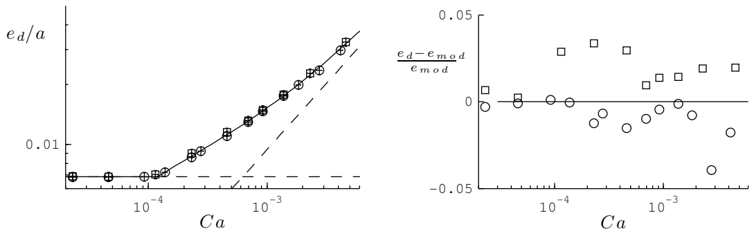
FIGURE 2.9 – À gauche : épaisseur normalisée ( e_d/a ) déposée sur une surface texturée ( p = 10 \mu\text{m} , h_p = 10,2 \mu\text{m} ), en fonction de Ca . La courbe en traits pleins est le meilleur ajustement par le modèle à deux couches, obtenu pour \alpha = 9,5 . Les courbes tiretées représentent respectivement la hauteur des piliers et la théorie de LLD. À droite : résidus normalisés. Les différents symboles indiquent la viscosité de l'huile utilisée : \eta = 19 mPa·s (o) et 97 mPa·s (□).
