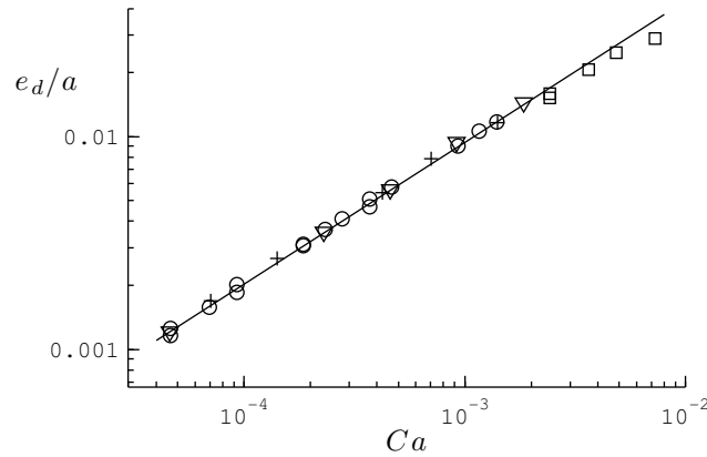
FIGURE 1.7 – e_d/a en fonction de Ca . La droite a pour équation e_d/a = 0,94 Ca^{2/3} . Huiles de viscosités 2,7 mPa·s (+), 9,5 mPa·s (○), 97 mPa·s (□), et 980 mPa·s (▽).
