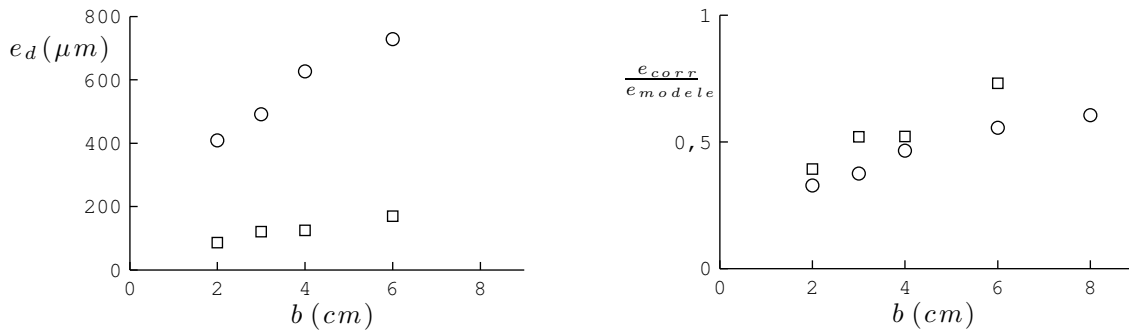
FIGURE 4.18 – Épaisseur de liquide déposé pour différentes largeurs de dépôt b . L = 4 cm (○) ou L = 2 cm (□), toujours dans la configuration de "mouillage total" ( \tilde{y}_0 = \tilde{y}_m , soit y_0 = 18,4 mm et y_0 = 9,2 mm, respectivement). Les autres paramètres de l'expérience sont \eta = 17,4 Pa·s, V = 8,2 mm/s, B = 4,2 \cdot 10^{-3} N·m. Dans le graphe de droite, l'épaisseur a été corrigée pour tenir compte de la différence entre la largeur de la plaque de dépôt et la largeur du racloir, et adimensionnée par l'épaisseur prédite par le modèle (1,5 mm pour L = 4 cm et 260 \mu m pour L = 2 cm ).
