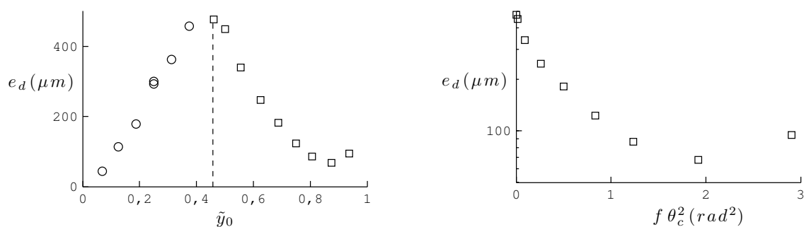
FIGURE 5.6 – À gauche : épaisseur e_d déposée par un racloir flexible en fonction de \tilde{y}_0 . Dans cette expérience, V = 8,2 mm/s, B = 4,2 \cdot 10^{-3} N · m, L = 4 cm et \eta = 17,4 Pa · s. Les pointillés représentent \tilde{y}_0 = \tilde{y}_m . À droite : les données pour y_0 > y_m sont tracées en fonction de f \theta_c^2 (les autres correspondent à \theta_c = 0 ), dans un diagramme semilogarithmique. On n'observe pas la décroissance en \exp(-f \theta_c^2) attendue pour un racloir rigide.
