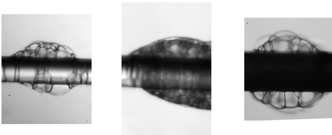
FIGURE D.5 – Photographie des paquets émis lors de l’enduction d’une fibre de Nylon. De gauche à droite : V = 40 mm/s et b = 40 \mu\text{m} , V = 200 mm/s et b = 40 \mu\text{m} , V = 100 mm/s et b = 75 \mu\text{m} .
