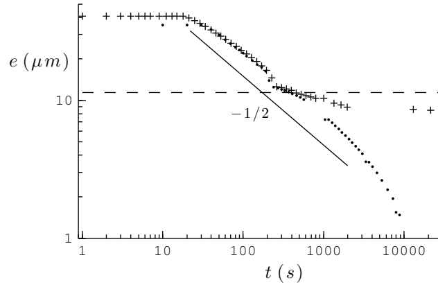
FIGURE 3.15 – Expérience de drainage pour p = 66 \mu\text{m} , h_p = 11,4 \mu\text{m} , \eta = 19,5 \text{ mPa} \cdot \text{s} . + : mesure en x = 4 \text{ mm} , valeur pour laquelle l'épaisseur en fin de drainage vaut 7 \mu\text{m} (cf. figure 3.14). • : mesure en x = 2 \text{ cm} > x_{\text{max}} , l'épaisseur finale est alors nulle. La ligne horizontale représente h_p , tandis que la droite en trait plein décrit une loi de puissance en t^{-1/2} , caractéristique du drainage sur une surface lisse.
