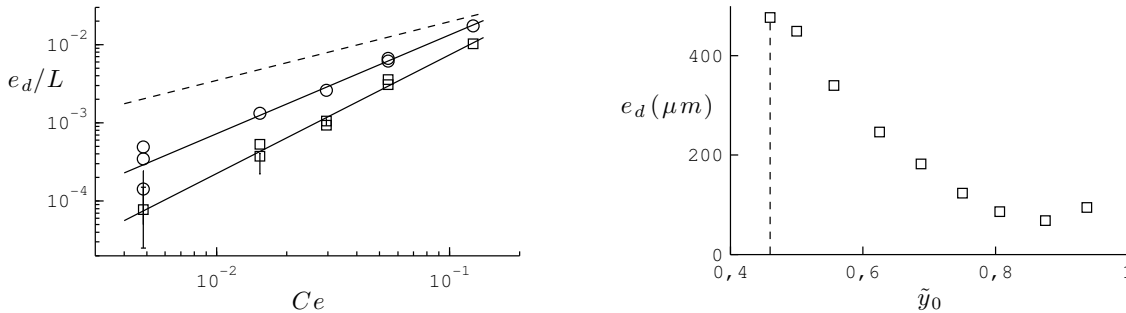
FIGURE 4.23 – Épaisseur de liquide déposée dans le régime de "mouillage partiel", pour B = 4,2 \cdot 10^{-3} \text{ N}\cdot\text{m} , L = 4 \text{ cm} , \eta = 17,4 \text{ Pa}\cdot\text{s} . À gauche : effet de V (de 0,7 \text{ mm/s} à 19 \text{ mm/s} ) sur l'épaisseur déposée pour y_0 = 25 \text{ mm} ( \circ , soit \tilde{y}_0 = 0,63 ) et y_0 = 30 \text{ mm} ( \square , soit \tilde{y}_0 = 0,75 ). La courbe en pointillés décrit le dépôt dans le cas mouillant, tandis que les ajustements en lois de puissance représentés sont d'exposants 1,3 et 1,5. À droite : e_d en fonction de \tilde{y}_0 , pour V = 8 \text{ mm/s} . Les pointillés figurent le cas mouillant.
