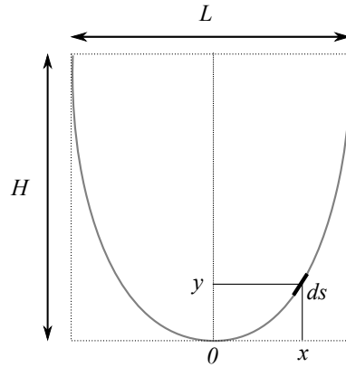
FIGURE 7.16 – Schéma de la "chaînette visqueuse".
