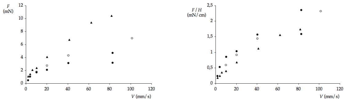
FIGURE D.11 – à gauche : force F exercée par la mousse sur un fil de 200\ \mu\text{m} de diamètre, en fonction de la vitesse de tirage V . On réalise l'expérience avec des tubes de longueur H = 2 cm (●), H = 3 cm (○) et H = 6 cm (▲). À droite : les mêmes mesures se superposent lorsque l'on trace F/H en fonction de la vitesse.
