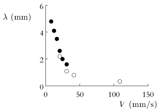
FIGURE D.6 – Longueur d’onde d’émission des paquets, en fonction de la vitesse de tirage, pour une fibre de Nylon de 200 \mu\text{m} (○) ou 700 \mu\text{m} (●) de diamètre.
