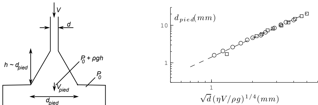
FIGURE 6.18 – À gauche : schéma du pied du filament. À droite : d_{\text{pied}} en fonction du membre de droite de l'équation 6.3. Notez que d et V sont mesurés directement dans ces expériences. D = 13 mm, \eta = 12 Pa·s, L = 12 mm ( \circ ) ou L = 22 mm ( \square ). Les tirets représentent une loi de puissance d'exposant 1,7.
