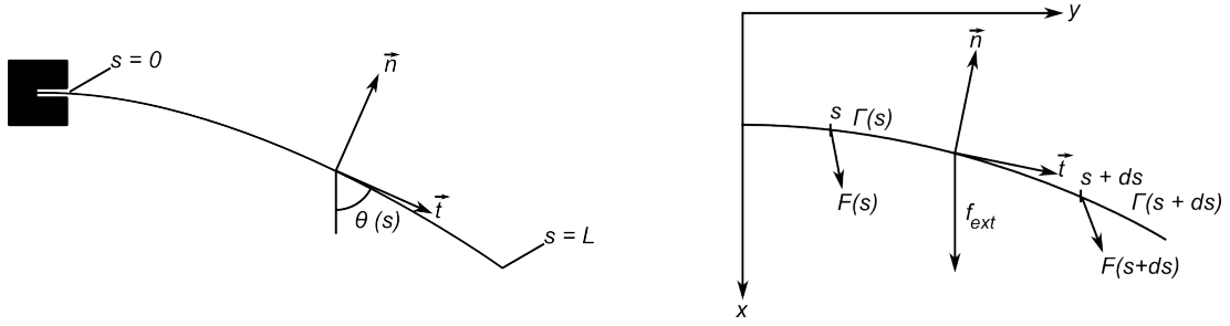
FIGURE B.1 – Notations utilisées pour exprimer l'équilibre mécanique d'une poutre. \vec{F}(s) et \Gamma(s) sont la force et le couple exercés en un point de la poutre par la portion de poutre située "à sa droite".
