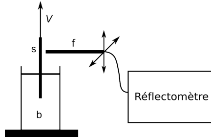
FIGURE 1.1 – Schéma de l'expérience de dip-coating. Le solide à enduire ( s ), est fixe, et c'est le bain de liquide ( b ) qui se déplace à la vitesse V ( 1 \mu\text{m} \cdot \text{s}^{-1} < V < 1 \text{cm} \cdot \text{s}^{-1} ). L'épaisseur de liquide déposée est mesurée par interférométrie, à l'aide de la fibre optique ( f ).
