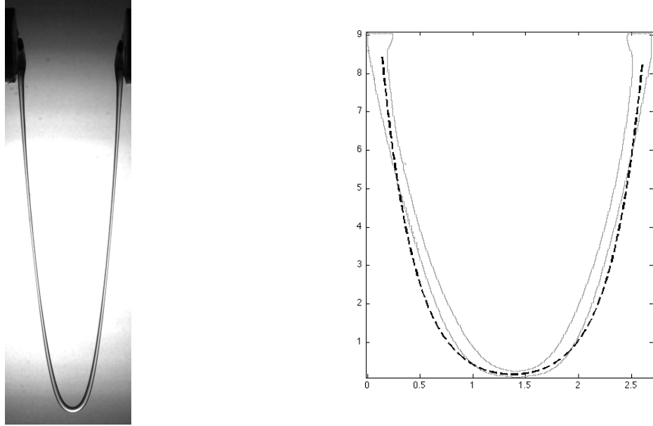
FIGURE 7.15 – À gauche : chaînette visqueuse d'huile silicone ( \eta = 9,7 \text{ Pa} \cdot \text{s} , L = 24 \text{ mm} et D = 2,3 \text{ mm} ), aux grandes déformations. À droite : on superpose à la forme de ce filament visqueux (en gris) la forme d'une chaînette (pointillés noirs) ayant les mêmes dimensions (les axes sont en centimètres).
