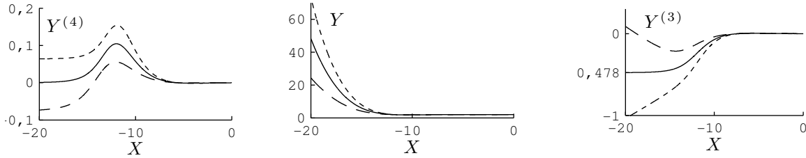
FIGURE 4.16 – Forme du racloir dynamique pour trois valeurs de Y(0) (figure centrale). La courbe en traits pleins présente Y(0) - 2 = 0,0012 , qui est comme l'illustre la première figure la valeur pour laquelle Y_{XXXX} \xrightarrow{X \rightarrow -\infty} 0 ). La dérivée troisième du profil tend alors vers une constante (égale à -0,4780 ) lorsque X \rightarrow -\infty (figure de droite). Les autres courbes correspondent à Y(0) - 2 = 0,0017 (tirets courts) et Y(0) - 2 = 0,0007 (tirets longs).
