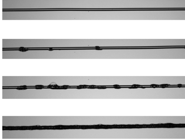
FIGURE D.3 – Dépôt de mousse sur une fibre de Nylon de 200\text{ }\mu\text{m} de diamètre, en fonction de la vitesse de la fibre. De haut en bas : V = 8\text{ mm/s} , V = 21\text{ mm/s} , V = 62\text{ mm/s} , V = 206\text{ mm/s} .
