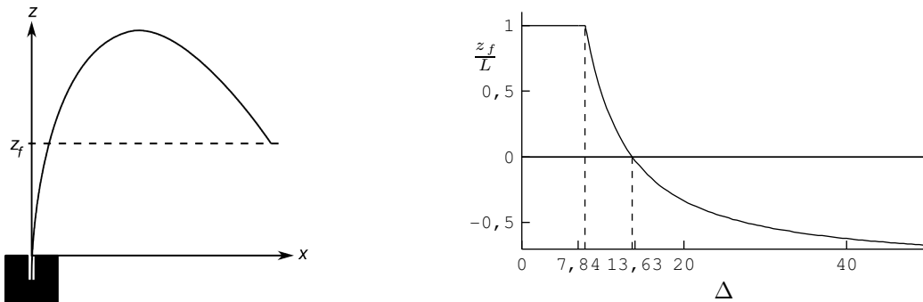
FIGURE B.2 – Méthode de mesure de la rigidité des racloirs : le racloir est encastré verticalement (à gauche), et on observe la hauteur z_f de son extrémité libre. La courbe de droite permet de relier cette hauteur au nombre sans dimension \Delta = \frac{\rho_s g L^3}{B} , ce qui permet de déterminer B (les tirets représentent \Delta = 7,837 , valeur analytique à partir de laquelle la poutre flambe sous son propre poids). En pratique, on recherche la longueur de racloir pour laquelle z_f = 0 , \Delta valant alors 13,634.
