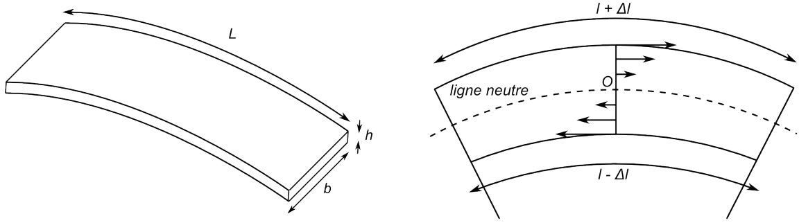
FIGURE 4.3 – Notations utilisées pour décrire les dimensions des racloirs utilisés (à gauche), et schéma d’une poutre courbée (à droite) : les flèches représentent l’allongement local.
