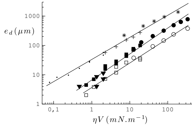
FIGURE 4.10 – Épaisseur déposée en fonction de \eta V , pour b = 3 \text{ cm} , \eta = 0,1 \text{ Pa} \cdot \text{s} ( \nabla et \cdot ), \eta = 0,98 \text{ Pa} \cdot \text{s} ( \square et + ) et \eta = 17,4 \text{ Pa} \cdot \text{s} ( \circ et * ). Les grands symboles ( \circ , \square , \nabla ) sont pour L = 4 \text{ cm} , les symboles pleins correspondant à un racloir de rigidité B = 4,2 \cdot 10^{-3} \text{ N} \cdot \text{m} et les symboles vides à B = 14,3 \cdot 10^{-3} \text{ N} \cdot \text{m} . Les petits symboles ( \cdot , + , * ) représentent L = 6 \text{ cm} et B = 4,2 \cdot 10^{-3} \text{ N} \cdot \text{m} . Les lois de puissance représentées sont d'exposant 0,75, 0,88 et 0,83.
