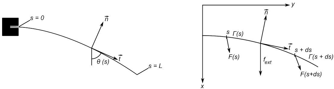
FIGURE 4.4 – Notations utilisées pour exprimer l'équilibre mécanique d'une poutre. \vec{F}(s) et \Gamma(s) sont la force et le couple exercés en un point de la poutre par la portion de poutre située "à sa droite".
