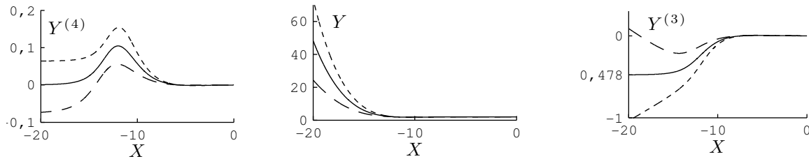
FIGURE 4.16 – Forme du raclor dynamique pour trois valeurs de Y(0) (figure centrale). La courbe en traits pleins présente Y(0) - 2 = 0,0012 , qui est comme l'illustre la première figure la valeur pour laquelle Y_{XXXX} \xrightarrow{X \rightarrow -\infty} 0 ). La dérivée troisième du profil tend alors vers une constante (égale à -0,4780 ) lorsque X \rightarrow -\infty (figure de droite). Les autres courbes correspondent à Y(0) - 2 = 0,0017 (tirets courts) et Y(0) - 2 = 0,0007 (tirets longs).
