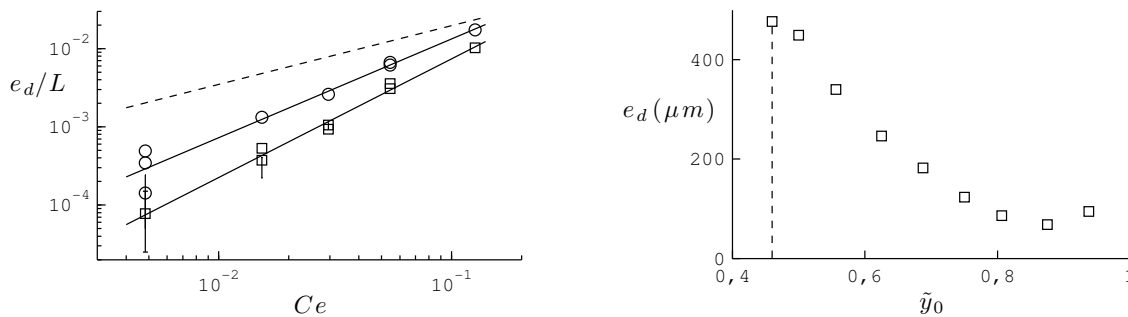
FIGURE 4.23 – Épaisseur de liquide déposée dans le régime de "mouillage partiel", pour B = 4,2 \cdot 10^{-3} \text{ N} \cdot \text{m} , L = 4 \text{ cm} , \eta = 17,4 \text{ Pa} \cdot \text{s} . À gauche : effet de V (de 0,7 \text{ mm/s} à 19 \text{ mm/s} ) sur l'épaisseur déposée pour y_0 = 25 \text{ mm} ( \circ , soit \tilde{y}_0 = 0,63 ) et y_0 = 30 \text{ mm} ( \square , soit \tilde{y}_0 = 0,75 ). La courbe en pointillés décrit le dépôt dans le cas mouillant, tandis que les ajustements en lois de puissance représentés sont d'exposants 1,3 et 1,5. À droite : e_d en fonction de \tilde{y}_0 , pour V = 8 \text{ mm/s} . Les pointillés figurent le cas mouillant.
