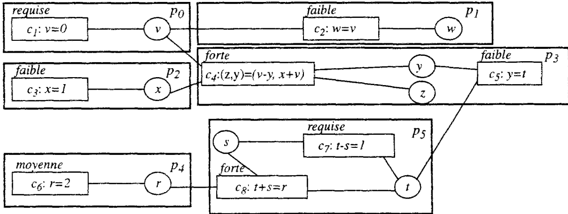
FIGURE 61 : Graphe admissible composé de cellules de contraintes
