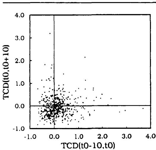
Figure VI.10.b: tcd sur 10 minutes avant et après t_0 pour 492 cellules de pluie convective
