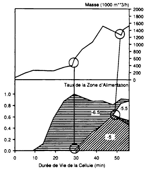
Figure VI.12.f: Cellule F (23.4.1990)
