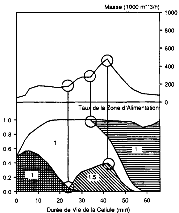
Figure VI.12.c: Cellule C (6.6.1989)
