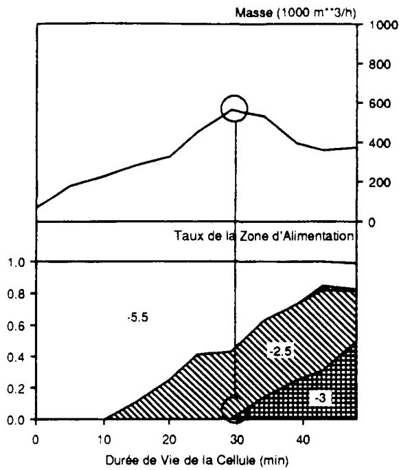
Figure VI.12.e: Cellule E (23.4.1990)
