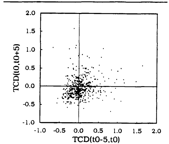
Figure VI.10.a: tcd sur 5 minutes avant et après t_0 pour 492 cellules de pluie convective
