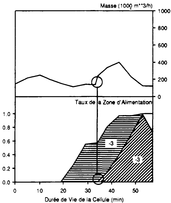
Figure VI.12.g: Cellule G (9.6.1990)
