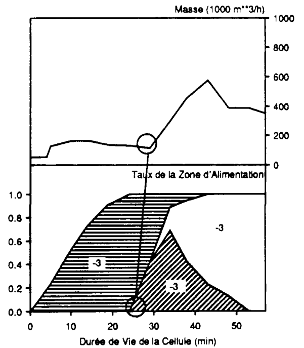
Figure VI.12.h: Cellule H (9.6.1990)
