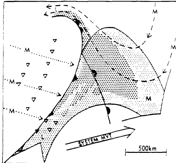
Figure I.3: Modèle des flux de masses d'air autour d'une perturbation (d'après Harrold et Austin 1974)
