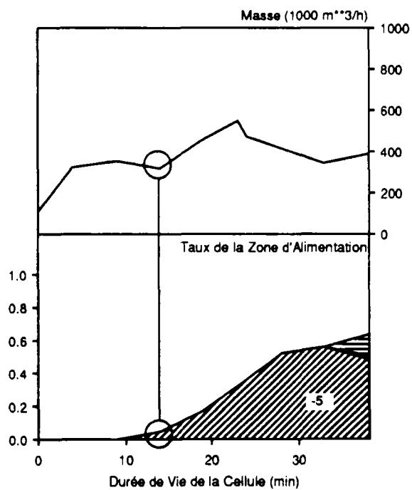
Figure VI.12.d: Cellule D (7.8.1989)
