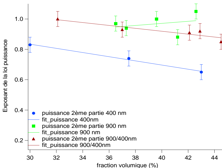
Figure 90 : Etude de la puissance observée en fonction de la fraction volumique dans la deuxième partie de la zone de rhéofluidification pour les différentes suspensions de particules de silice.
