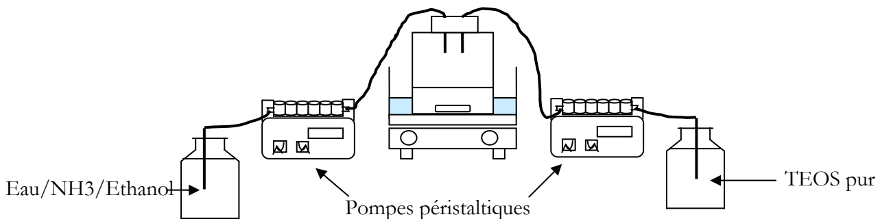
Figure 36 : Schéma du montage réalisé pour la croissance automatisée.
