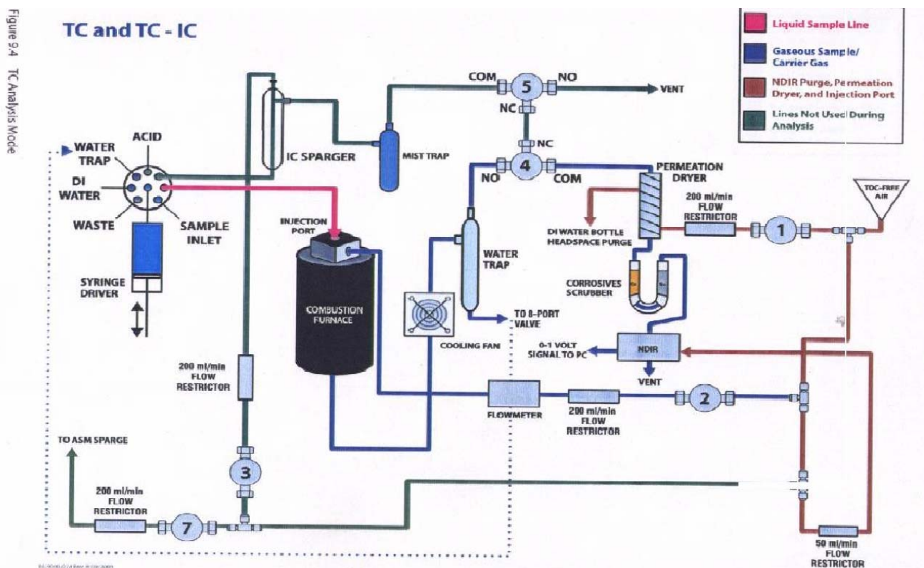
Figure 48 : Schéma de fonctionnement de l'analyseur de carbone total.
