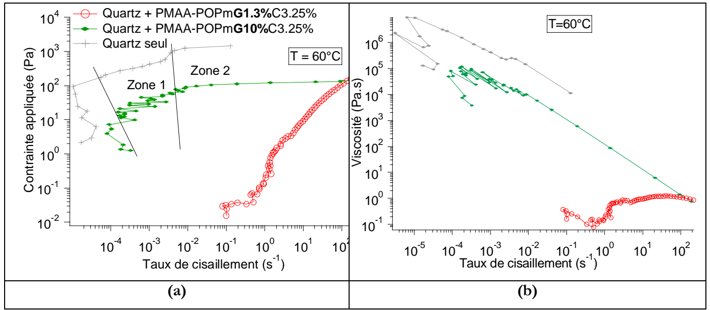
Figure 113 : Etude en écoulement des propriétés rhéologiques à 60^\circ\text{C} de suspensions de quartz sans polymère (en gris), avec du PMAA-POPm greffé à 1,3% (en rouge), avec du PMAA-POPm greffé à 10% (en vert). (a) Contraite en fonction du taux de cisaillement ; (b) Viscosité en fonction du taux de cisaillement.
