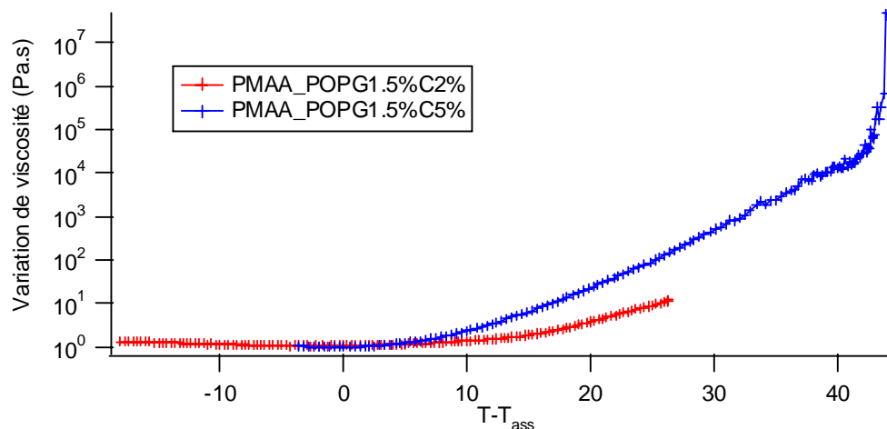
Figure 60 : Etude de la variation de viscosité du PMAA-POPm pour une concentration de 2% (en rouge) et de 5% (en bleu) en fonction de la température réduite par la température d'association T_{ass} .
