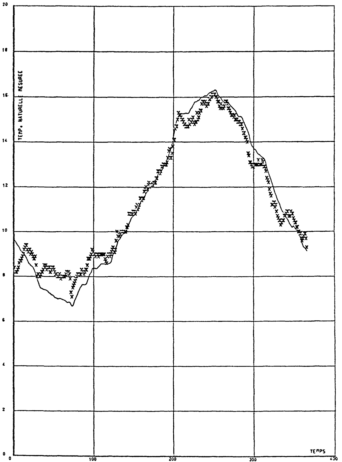
Figure 9 B : Comparaison calcul-mesures à Bassurelle.
