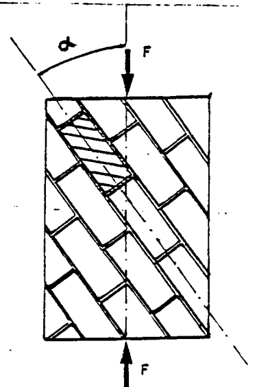
Fig. 7.6 MATERIAU ORTHOTROPE SIMPLEMENT COMPR SELON UNE DIRECTION QUELCONQUE
