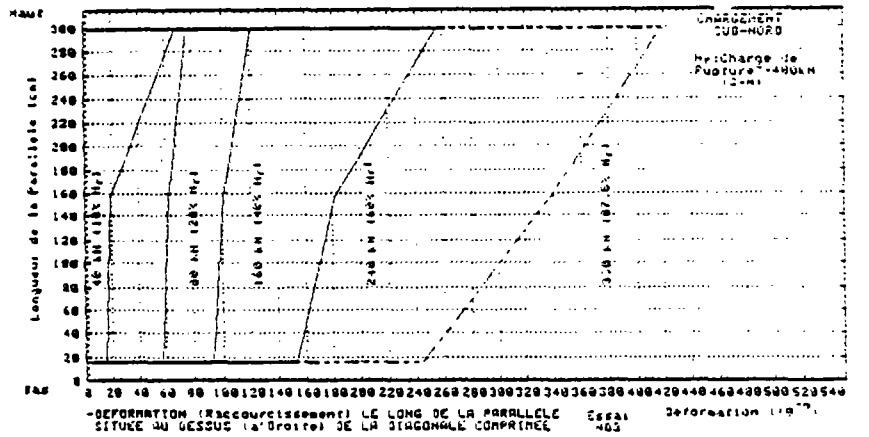
Fig. 3.3.5.6. - DEFORMATION LE LONG DES PARALLELES A LA DIAGONALE COMPRIMÉE
