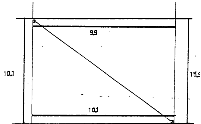
FIG. H.5 DIAGRAMME DES EFFORTS TRANCHANTS (kN) (H=380 kN)
