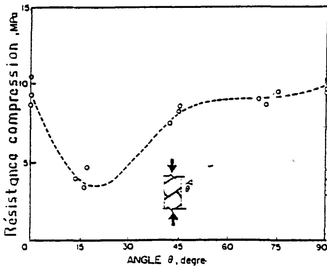
FIG. 7.7. : Effet de l'orientation des joints sur la résistance de compression axiale (d'après HAMID et DRYSDALE)
