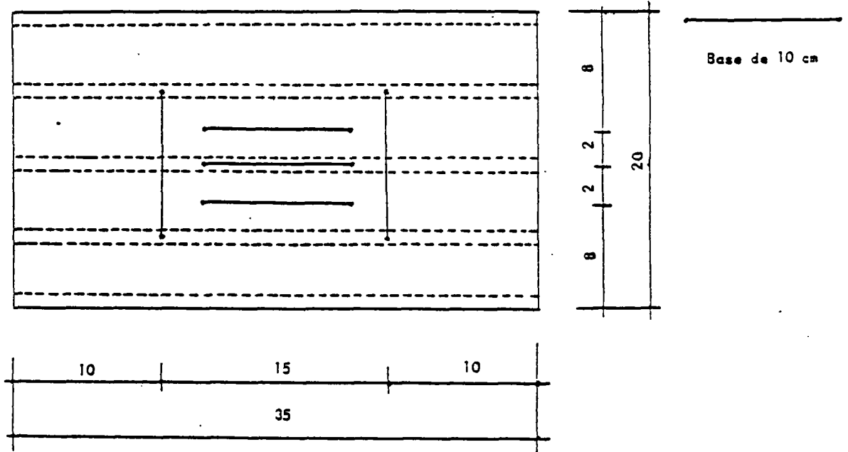
a.) BRIQUE CHARGÉE PERPENDICULAIREMENT AUX ALVEOLES
