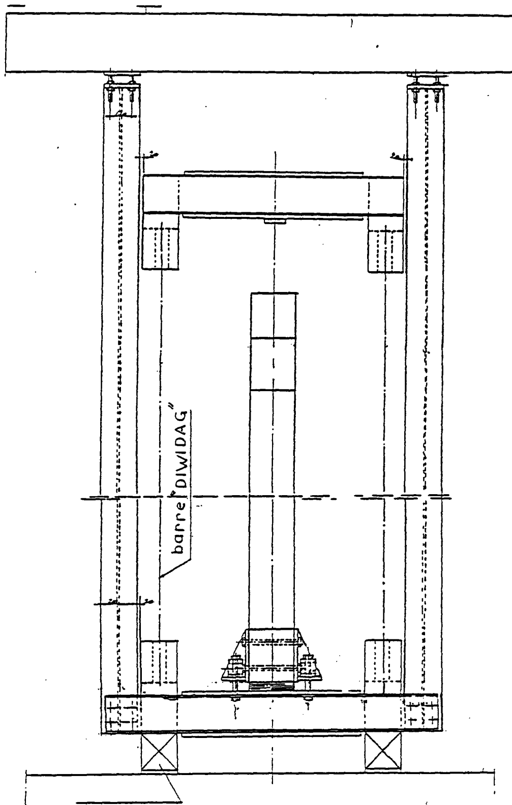
FIGURE 2.7.3. - Vue latérale
