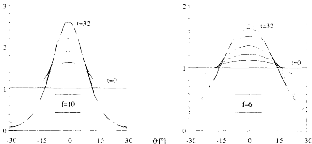
Fig.6: Evolution de la fonction d'orientation g(θ) en compression pour f réel.
