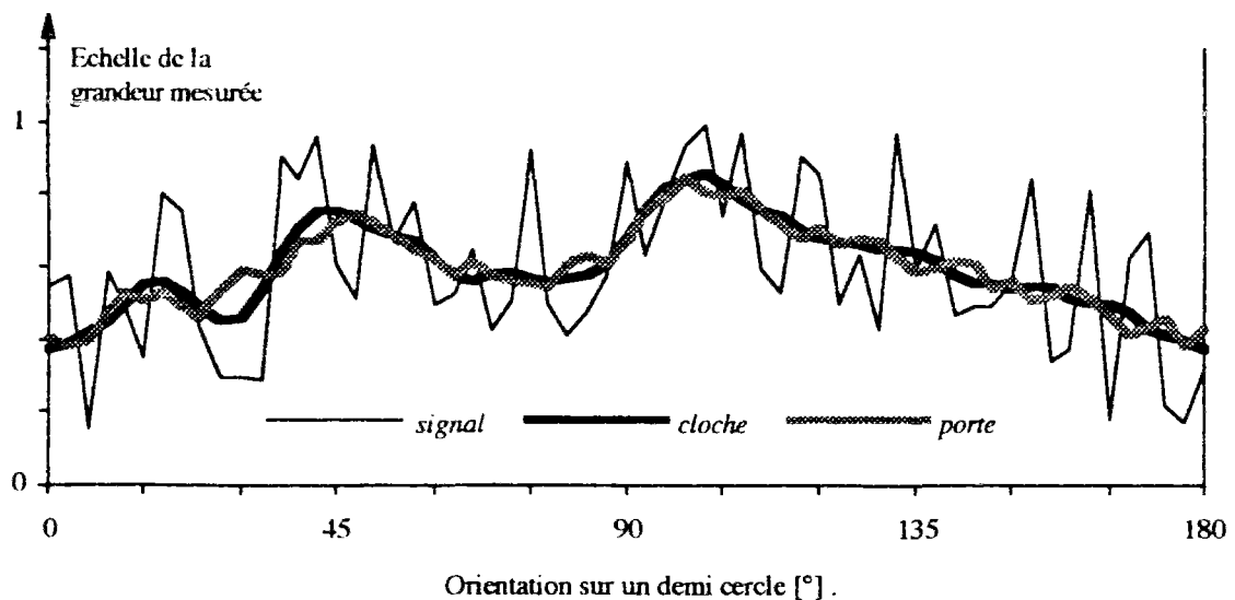
Fig.6: Comparaison des mesures par distribution cloche et par distribution porte d'un même signal.
