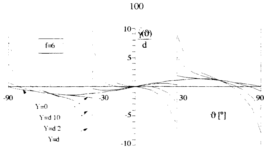
Fig.4: Graphe du taux de glissement pour f réel.
