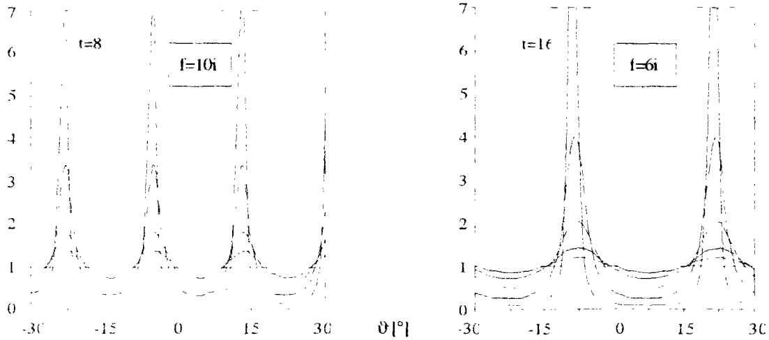
Fig. 11: Evolution de la fonction d'orientation g(\vartheta) en cisaillement pour f imaginaire.
