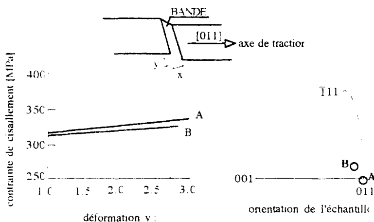
Fig.2: Ecroutissage positif après apparition des bandes de cisaillement (d'après [Dève et al. 1988]).
