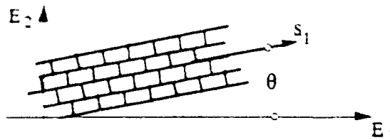
Fig.2: poly-lamelle à un glissement (d'après [van der Giessen et van Houtte 1992])
