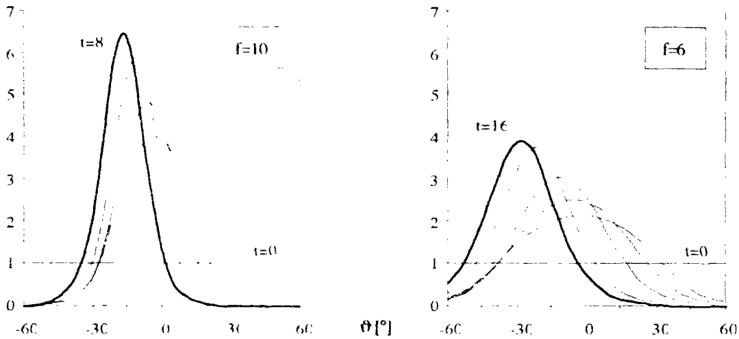
Fig.9: Evolution de la fonction d'orientation g(\vartheta) en cisaillement pour f réel.
