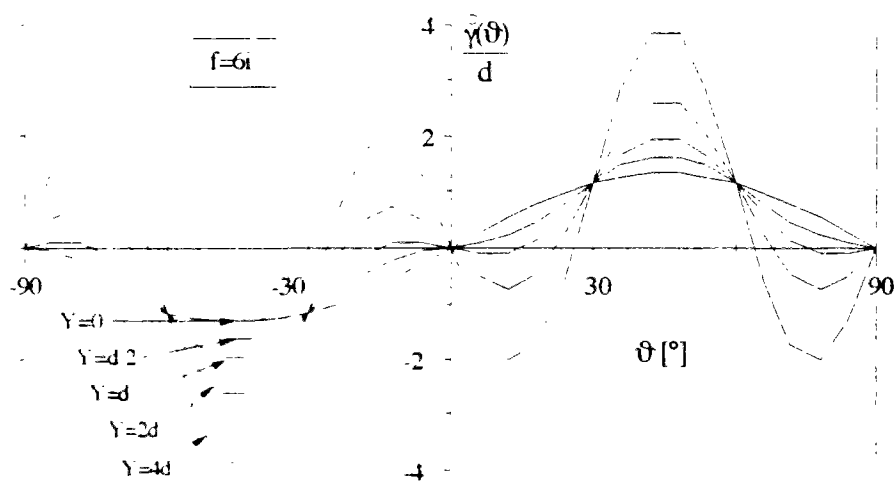
Fig.5: Graphe du taux de glissement pour f imaginaire.
