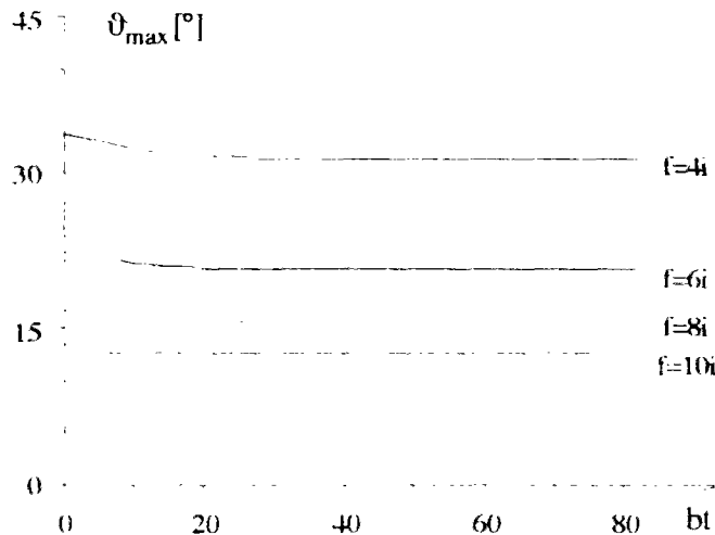
Fig. 12: Evolution de l'orientation plus fréquent en cisaillement pour f imaginaire.
